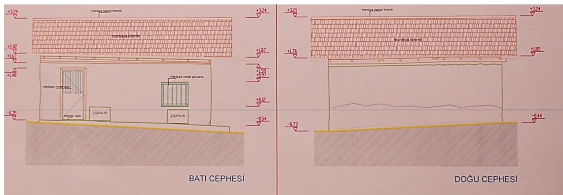
Çizim 23: Ali Kâhya Efendi Türbesi, Doğu ve Batı Cephesi Rölövesi
