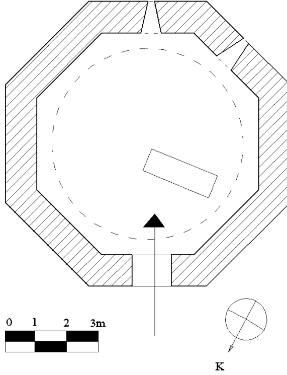
Çizim 12: Ali Baba Türbesi, Planı
