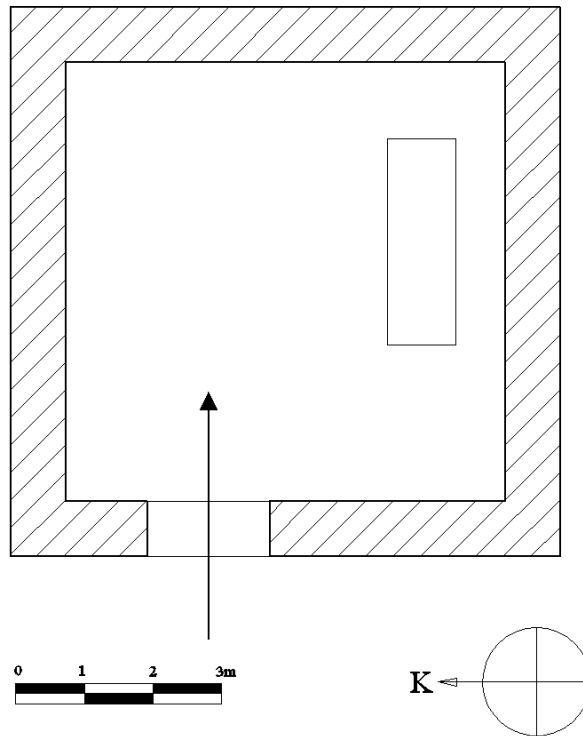
Çizim 29: Yukarı Tekke Dede Türbesi, Planı
