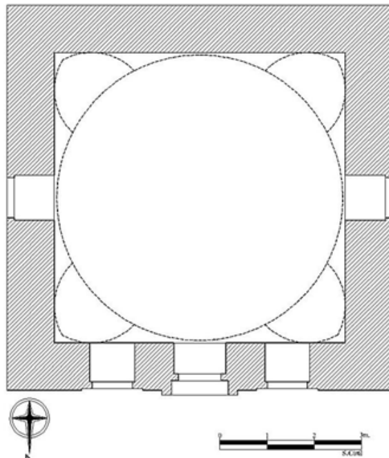
Çizim 11: Hüsameddin Bey Türbesi, Planı (S. Cirtil'den)
