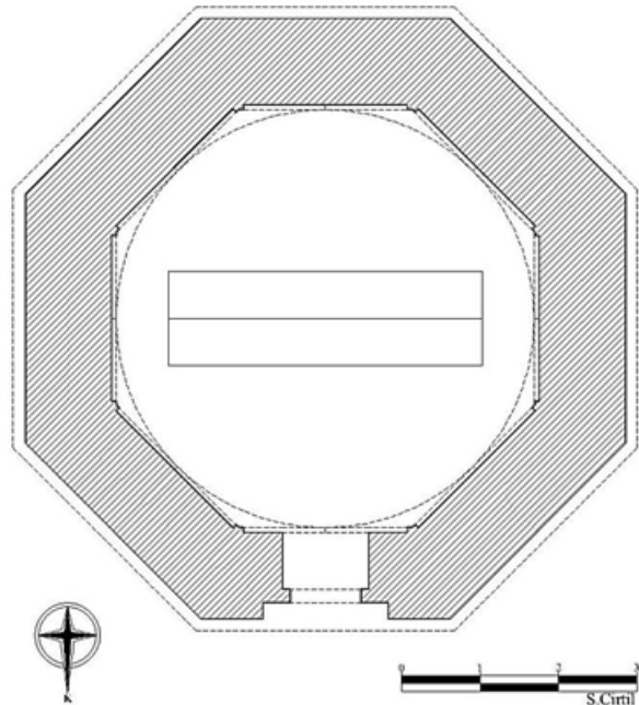
Çizim 10: Büyük Tekke (Emir Sultan) Türbesi, Planı (S. Cirtil'den)
