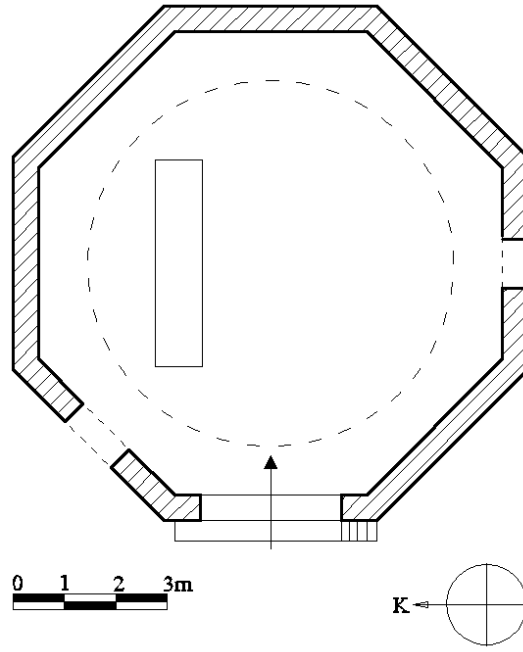
Çizim 31: Dedeler Dedesi Türbesi, Planı
