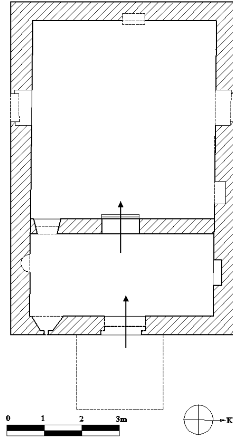
Çizim 21: Dediği Yaser Ali Sultan Türbesi, Planı
