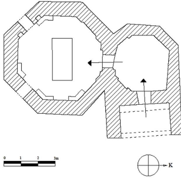
Çizim 13: Sultan Sarı Baba Türbesi, Planı
