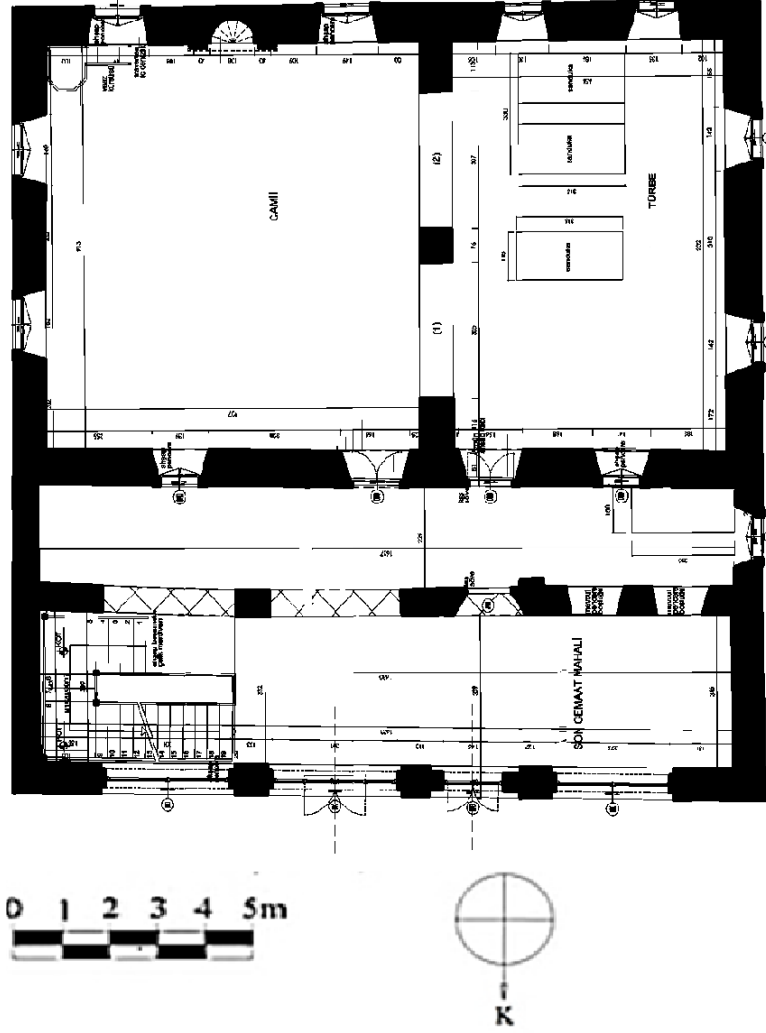
Çizim 20: Hasan Feyzi Efendi Cami ve Türbesi Planı (Zuhal Keskin, Denizli
