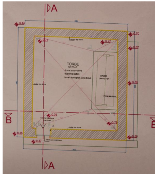
Çizim 22: Ali Kâhya Efendi Türbesi, Planı (Yonca Tarhan, Denizli Büyükşehir Belediyesi Arşivinden)
