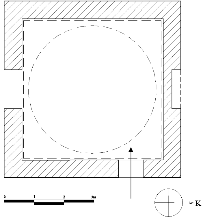
Çizim 9: Anonim Türbe I, Planı
