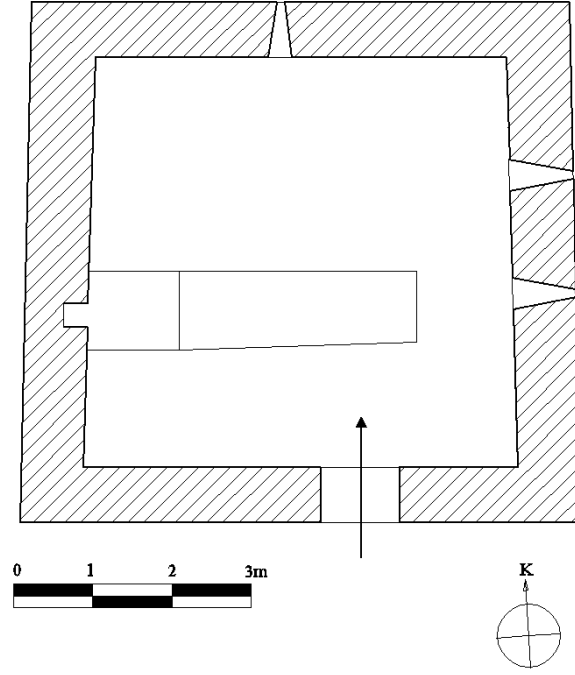
Çizim 16: Kazak Abdal(Sarı Gazak Baba) Türbesi, Planı
