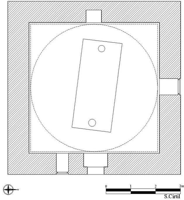
Çizim 2: Mahmud Gazi Türbesi, Planı (S. Cirtil'den)
