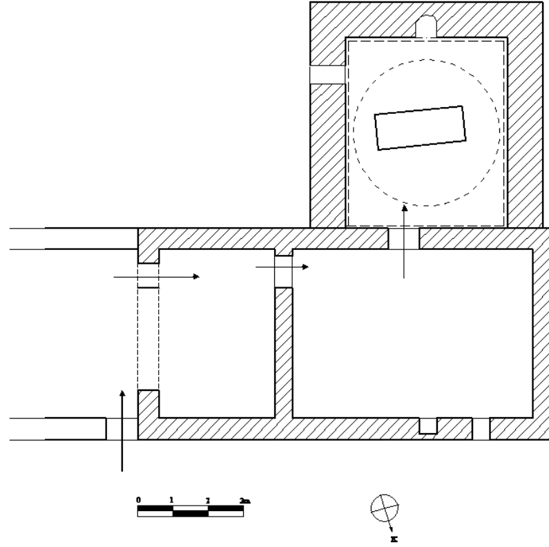
Çizim19: Karaca Ahmed Sultan Türbesi, Planı
