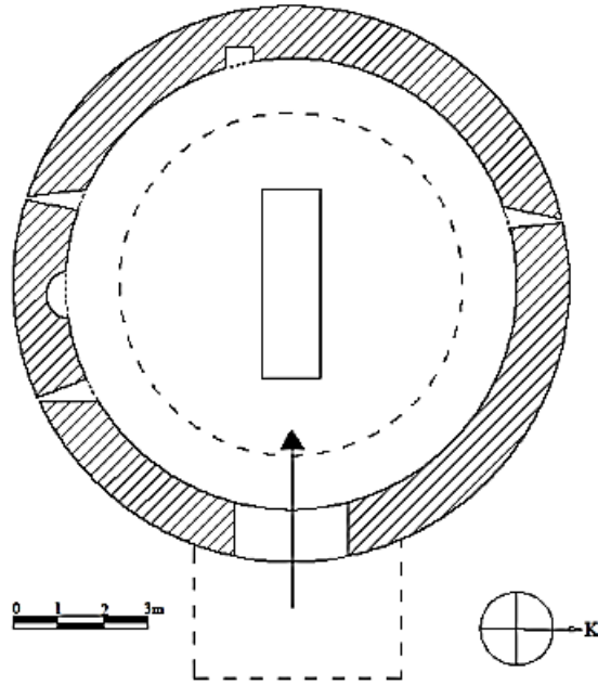
Çizim 30: Dümülcü Sultan Türbesi, Planı
