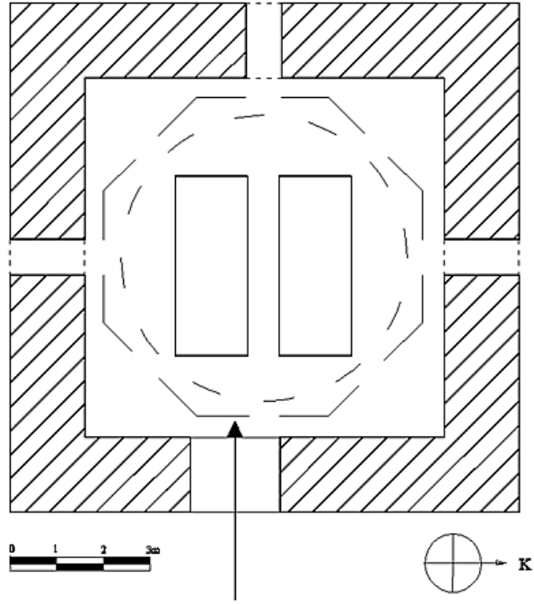
Çizim18: İmze Dede Sultan Türbesi, Planı
