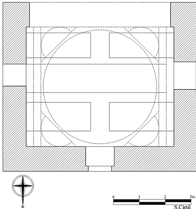
Çizim 15: Aşağı Cami Türbesi, Planı (S. Cirtil'den)
