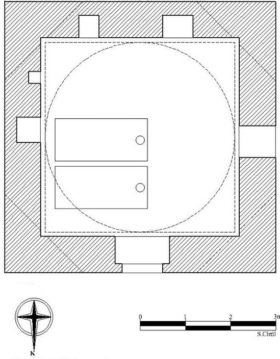
Çizim 14: Şaban Dede Türbesi, Planı.(S. Cirtil'den)
