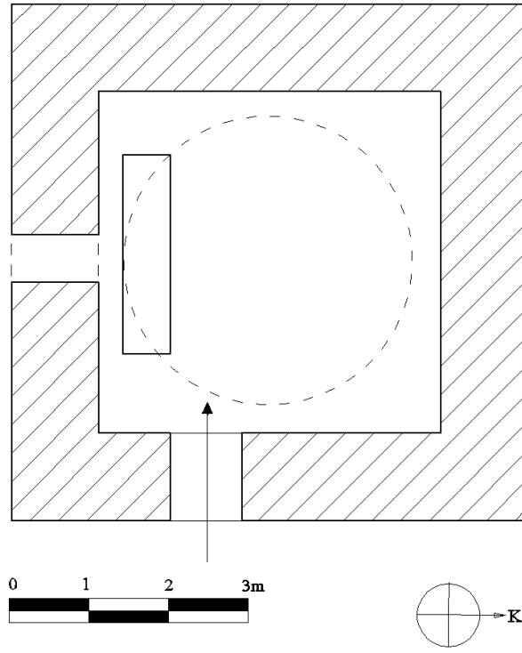
Çizim 27: Teslim Abdal Sultan Türbesi, Planı
