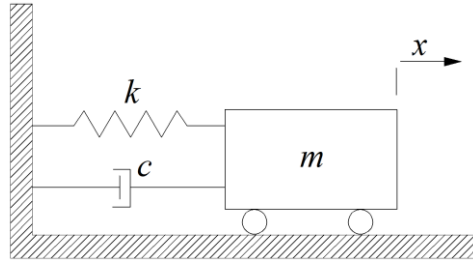
Şekil 2.10: TSD sistemin matematiksel modeli
