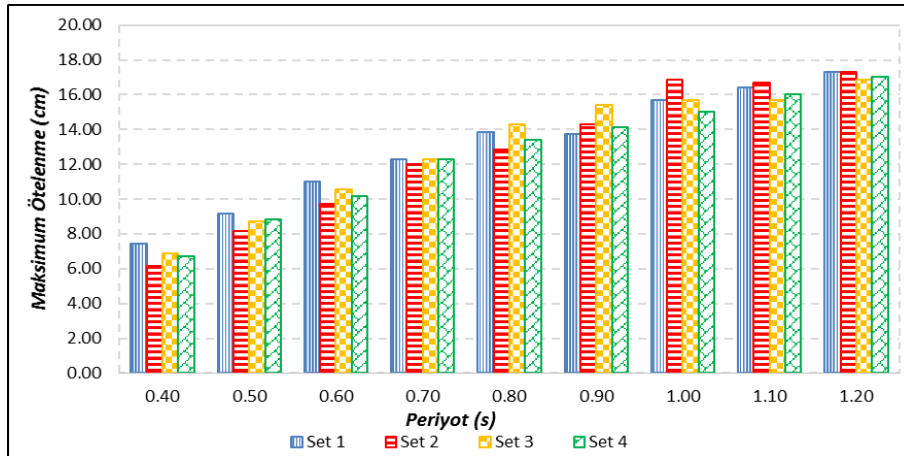
Şekil C.12: TSD sistemlerde Z3 için setlere ait \mu_{\Delta} değerleri (EDP model, F_y/W=0.2 )
