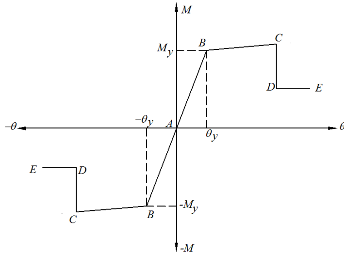
Şekil 2.7: Plastik mafsal için moment-dönme değerleri
