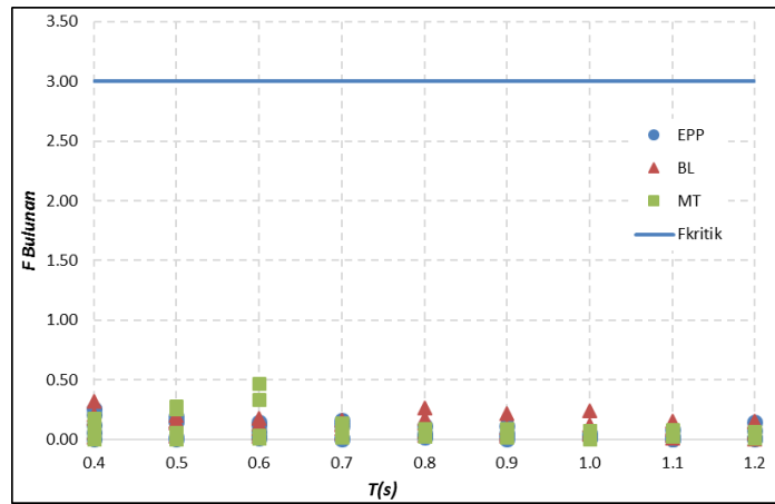
Şekil 6.3: TSD sistemlerde setlere ait \mu_{\Delta} değerleri için varyans analizi sonuçları (Z3)
