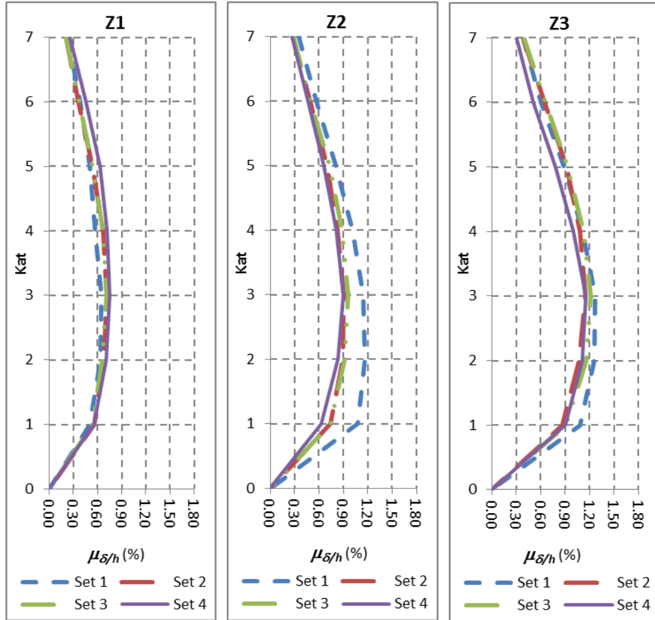
Şekil 5.31: 7 katlı çerçevede görel kat ötelenmesi oranı talebinin değişimi
