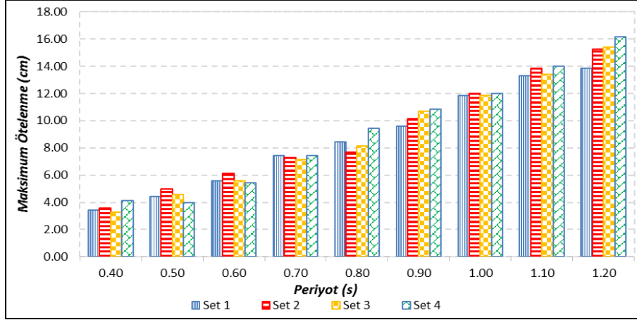
Şekil C.10: TSD sistemlerde Z2 için setlere ait \mu_{\Delta} değerleri (EDP model, F_y/W=0.5 )
