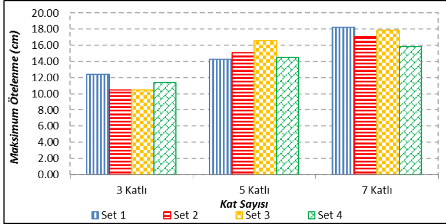
Şekil 5.24: Düzlem çerçevelerde Z3 için setlere ait \mu_A değerleri
