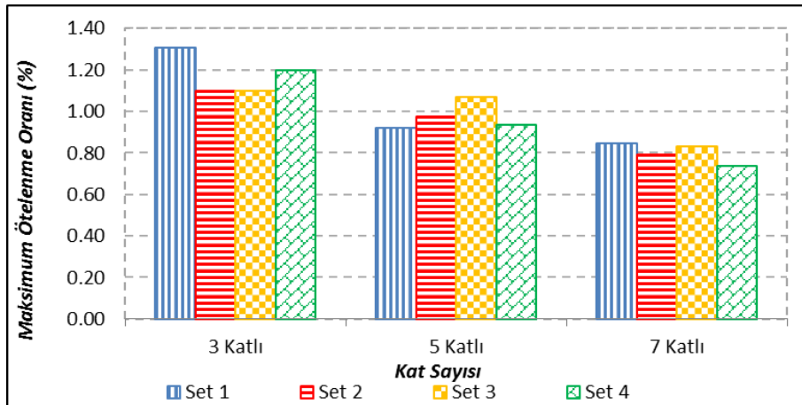
Şekil 5.25: Düzlem çerçevelerde Z3 için setlere ait \mu_{AH} değerleri
