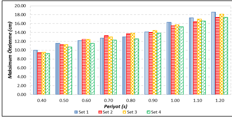
Şekil C.11: TSD sistemlerde Z3 için setlere ait \mu_{\Delta} değerleri (EDP model, F_y/W=0.1 )
