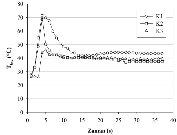
Şekil 13. Kullanım suyu sıcaklık farkının ve çıkış sıcaklığının zamanla değişimi (Time dependent change of temperature difference and outlet temperature of domestic water)
