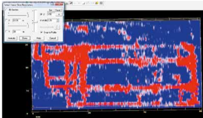
Res. 7 Kuzey Bazilikası'nın yer radarı ile çıkarılan planı.
