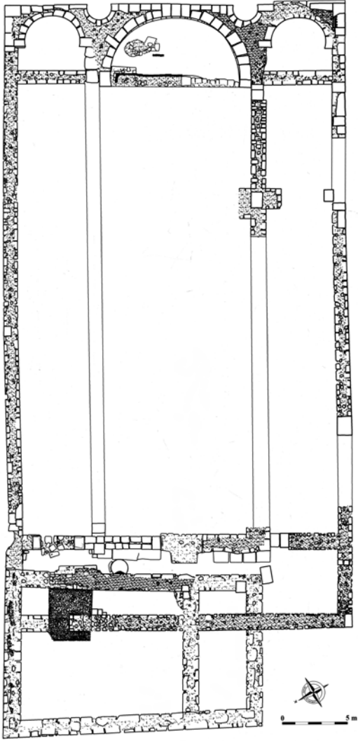
Res. 8 Kuzey Bazilikası'nın kazı sonunda çıkarılan planı.
