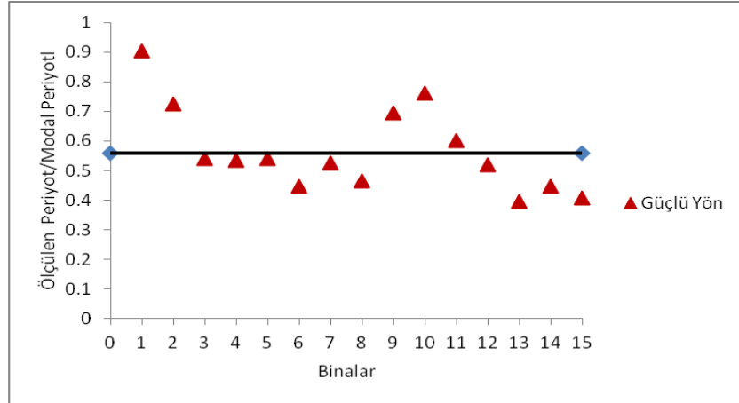
Şekil 5.5: Güçlü Yön Ait Ölçülen Periyot/Modal Periyot Oranları
