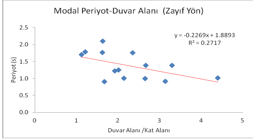
Şekil 5.50: Zayıf Yöne Ait Modal Yöntemle Bulunan Periyot- Bina Duvar Oranı Grafiği
