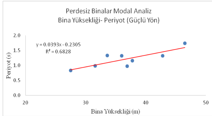
Şekil 5.29: Perdesiz Binalar Güçlü Yön Ait Bina Yüksekliği-Modal Periyot Grafiği
