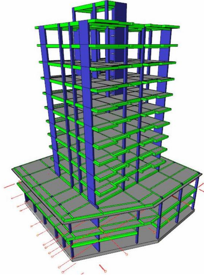
Şekil 3.25: 08 Nolu Binanın Bilgisayar Modeli.
