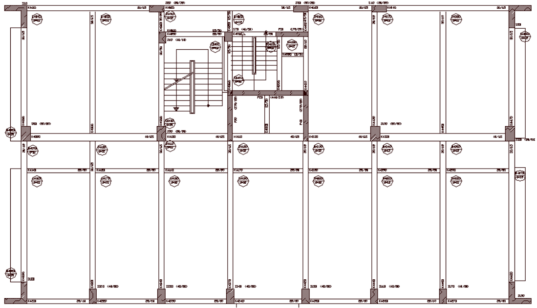
Şekil 3.16: 05 Nolu Bina'nın Üst Katlarına Ait Kalıp Planı.
