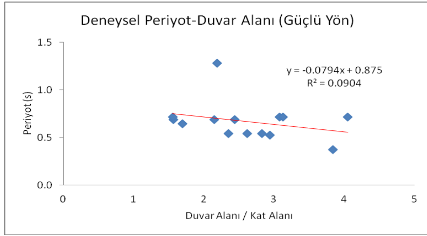
Şekil 5.51: Güçlü Yöne Ait Deneyisel Yöntemle Bulunan Periyot- Bina Duvar Oranı Grafiği
