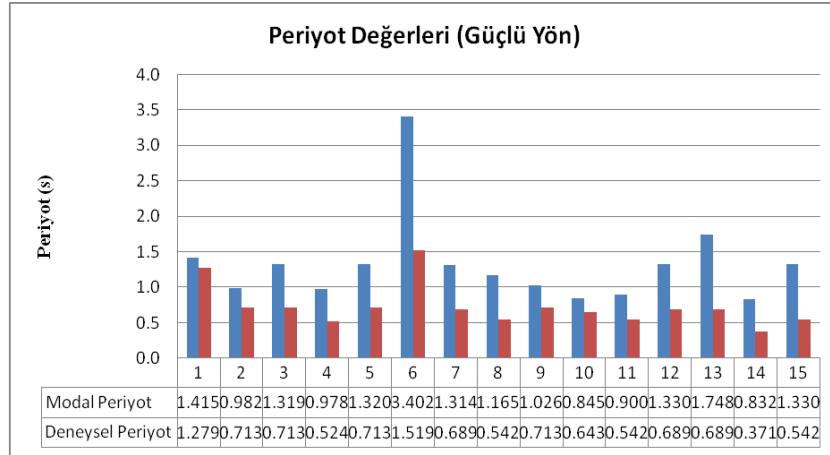
Şekil 5.3: Güçlü Yöne Ait İki Yöntemle Bulunan Periyot Değerlerinin Karşılaştırılması.
