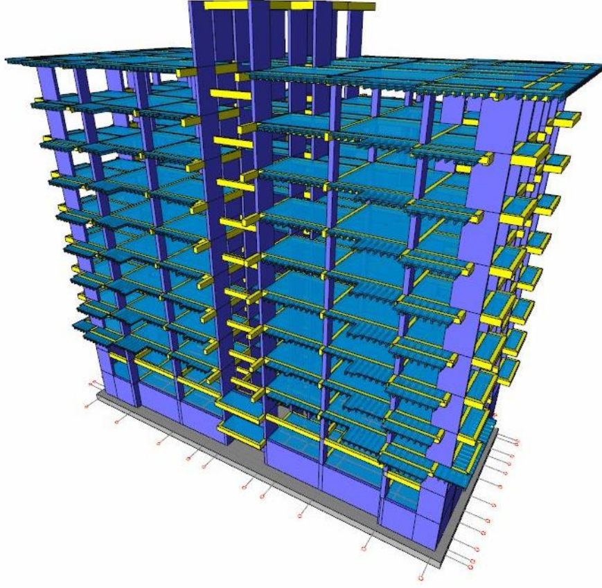
Şekil 3.7: 02 Nolu Binanın Bilgisayar Modeli.
