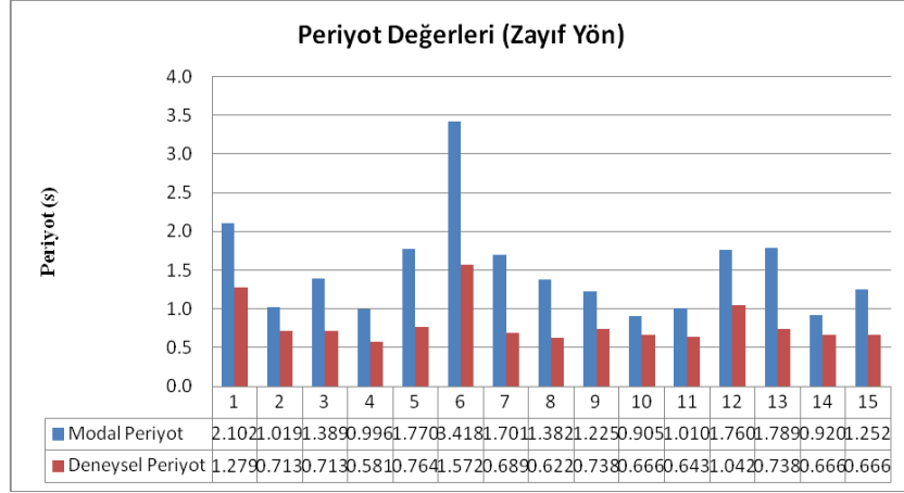
Şekil 5.4: Zayıf Yön Ait İki Yöntemle Bulunan Periyot Değerlerinin Karşılaştırılması.
