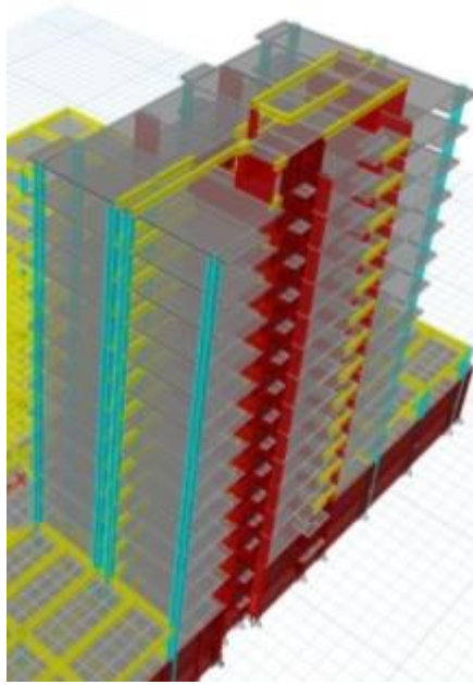
Şekil 3.36: 11 Nolu Binanın Bilgisayar Modeli.
