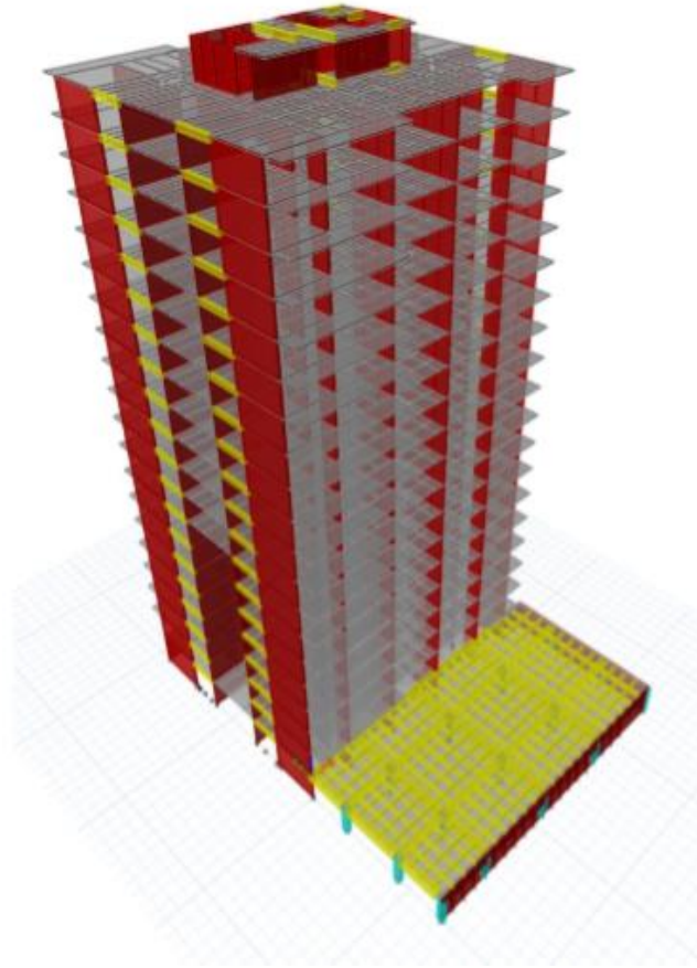
Şekil 3.28: 09 Nolu Binanın Bilgisayar Modeli.
