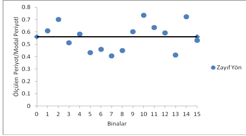
Şekil 5.6: Zayıf Yön Ait Ölçülen Periyot/Modal Periyot Oranları
