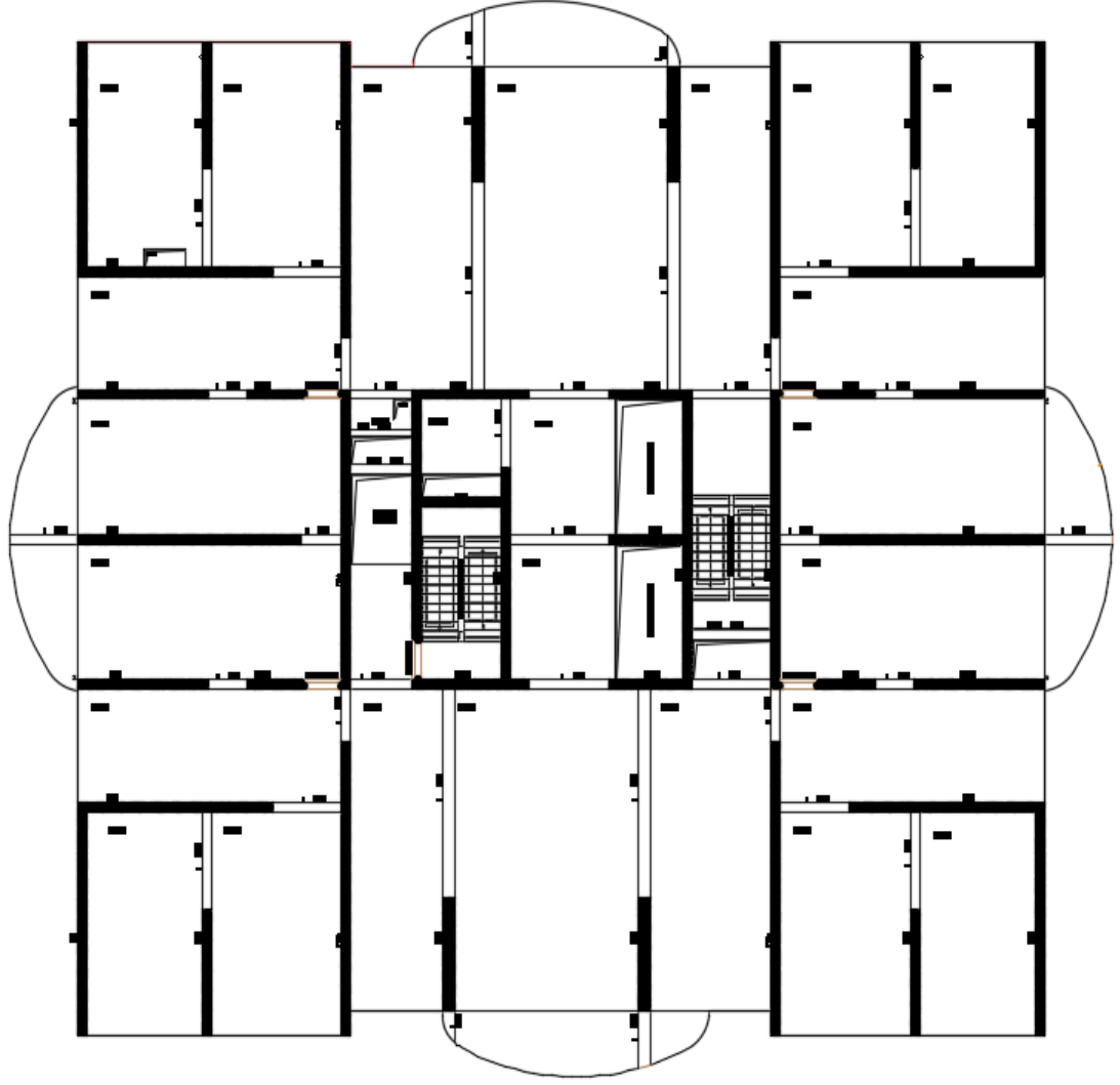
Şekil 3.19: 06 Nolu Binaya Ait Kalıp Planı
