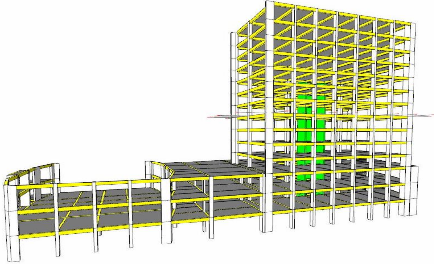
Şekil 3.17: 05 Nolu Binanın Bilgisayar Modeli.
