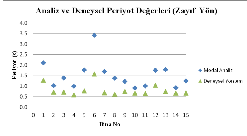
Şekil 5.2: Zayıf Yöne Ait Her İki Yöntemle Bulunan Periyot Değerleri.
