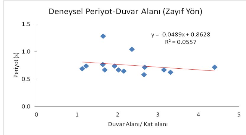
Şekil 5.52: Zayıf Yöne Ait Deneyisel Yöntemle Bulunan Periyot- Bina Duvar Oranı Grafiği
