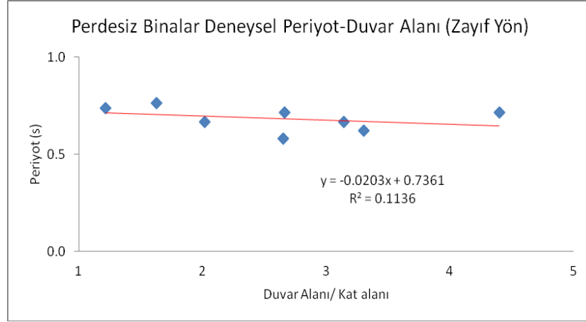
Şekil 5.62: Perdesiz Binalar Zayıf Yönüne Ait Bina Duvar Oranı-Deneyisel Periyot Grafiği
