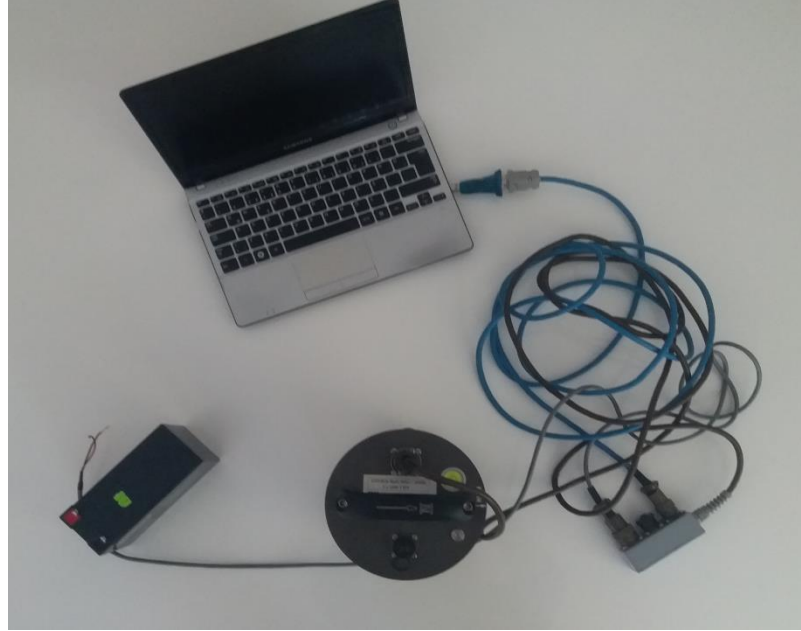
Şekil 2.1: Guralp CMG-6TD Mikrotremor Cihazı ve Diğer Ekipmanlar
