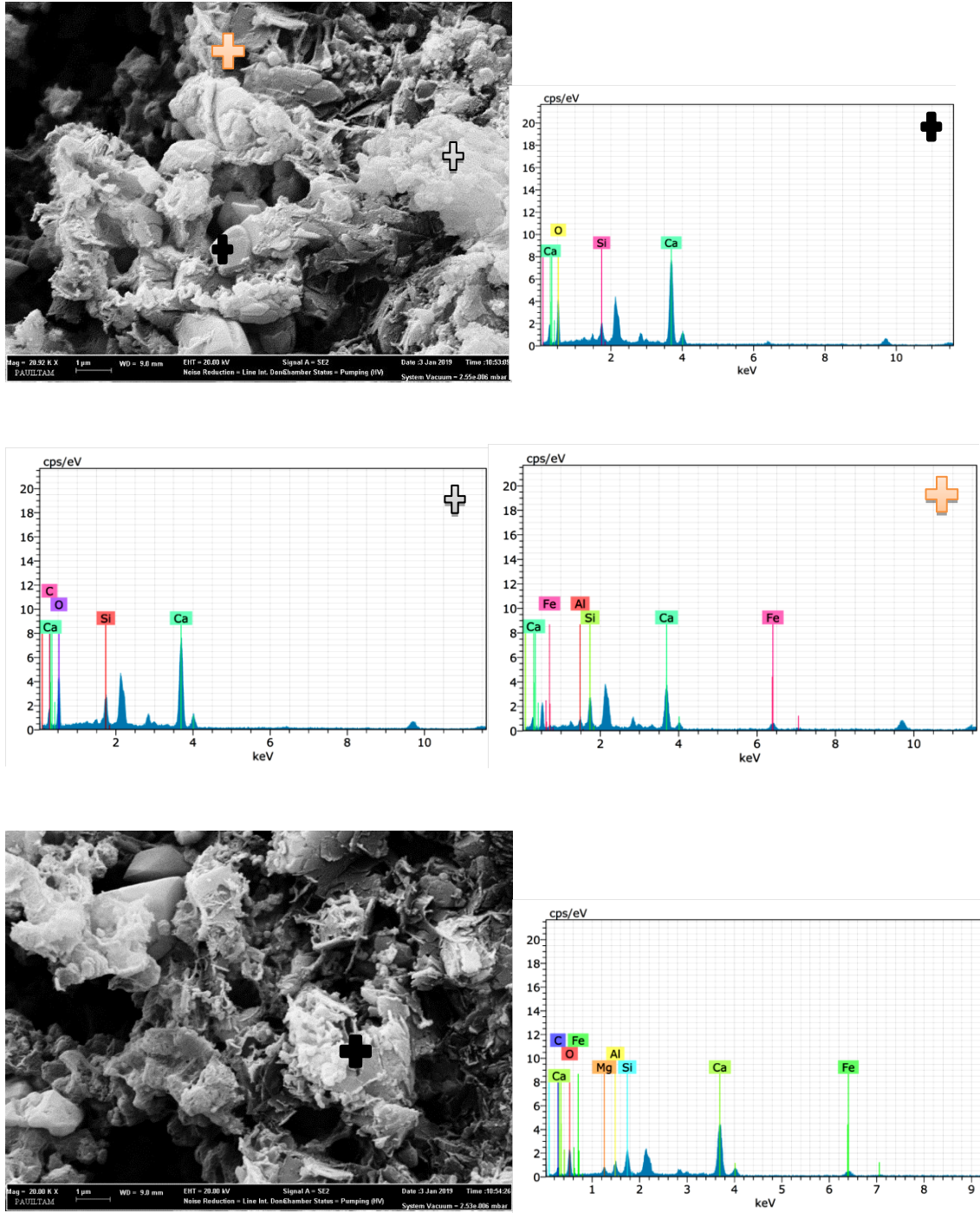
Figür 4.40 H12 örneğinin farklı noktalardan alınan SEM görüntüleri ve EDS diyagramları
