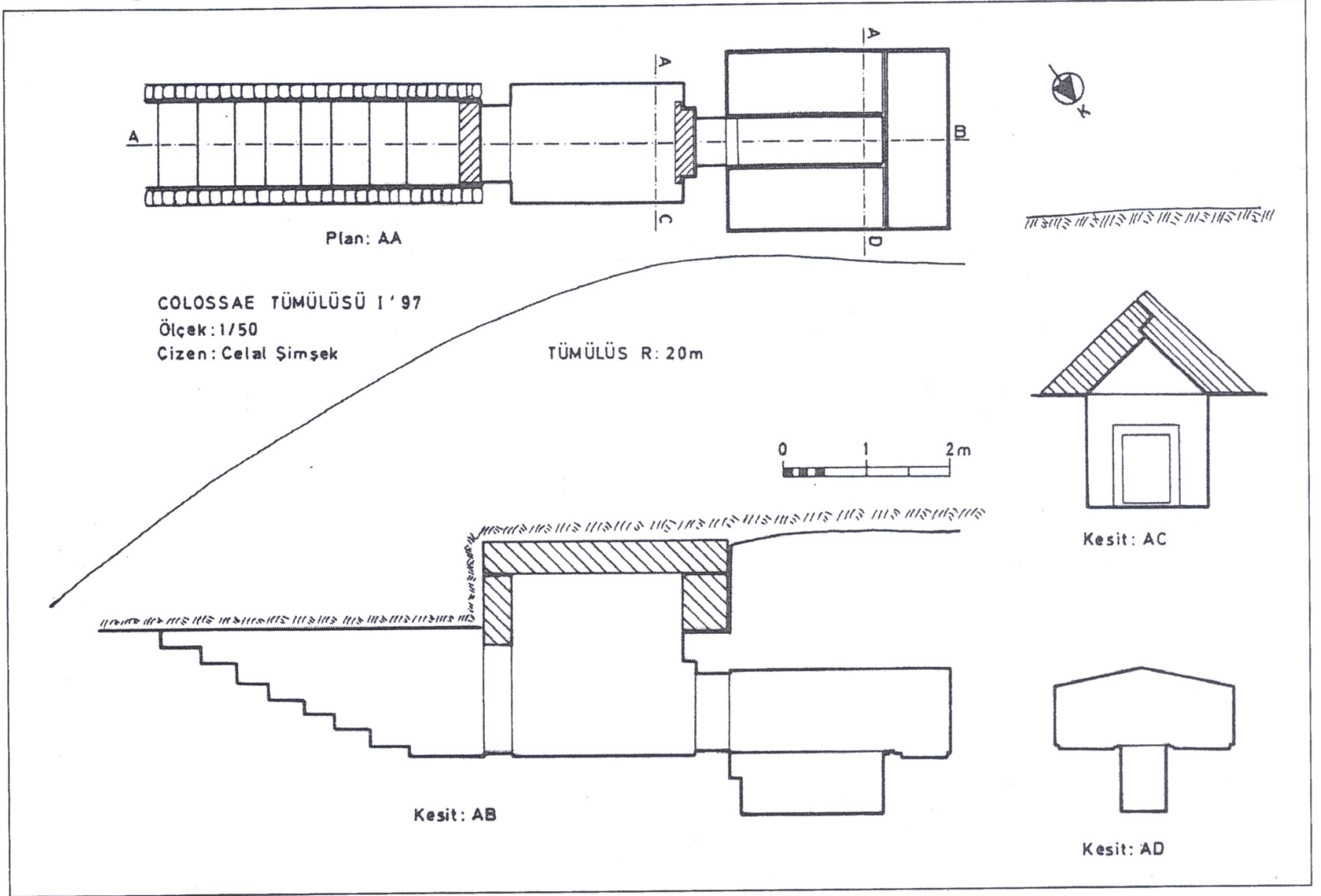
Çizim 1: Kolossai I nolu tümülüs mezar.
