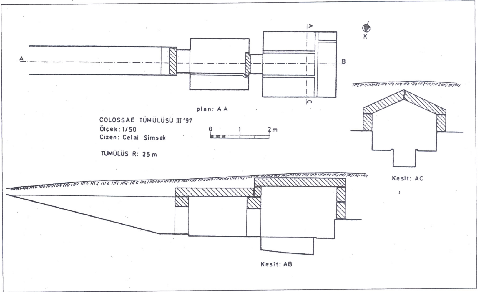
Çizim 2: Kolossai III nolu tumulus mezar.
