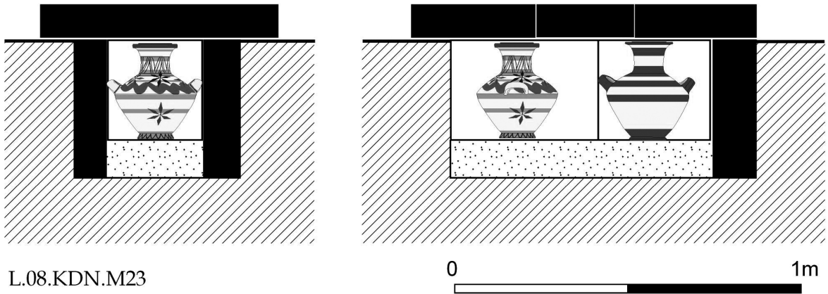
Res. 61 Kuzeydoğu Nekropolü'nden, içine kremasyon kapları yerleştirilen L.08.KDN.M23 numaralı traverten örgü tekne mezarın kesiti
