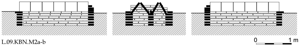
Res. 56 Kuzeybatı Neropolü'nden, tuğla örgülü ikiz tekne mezarın kesiti
