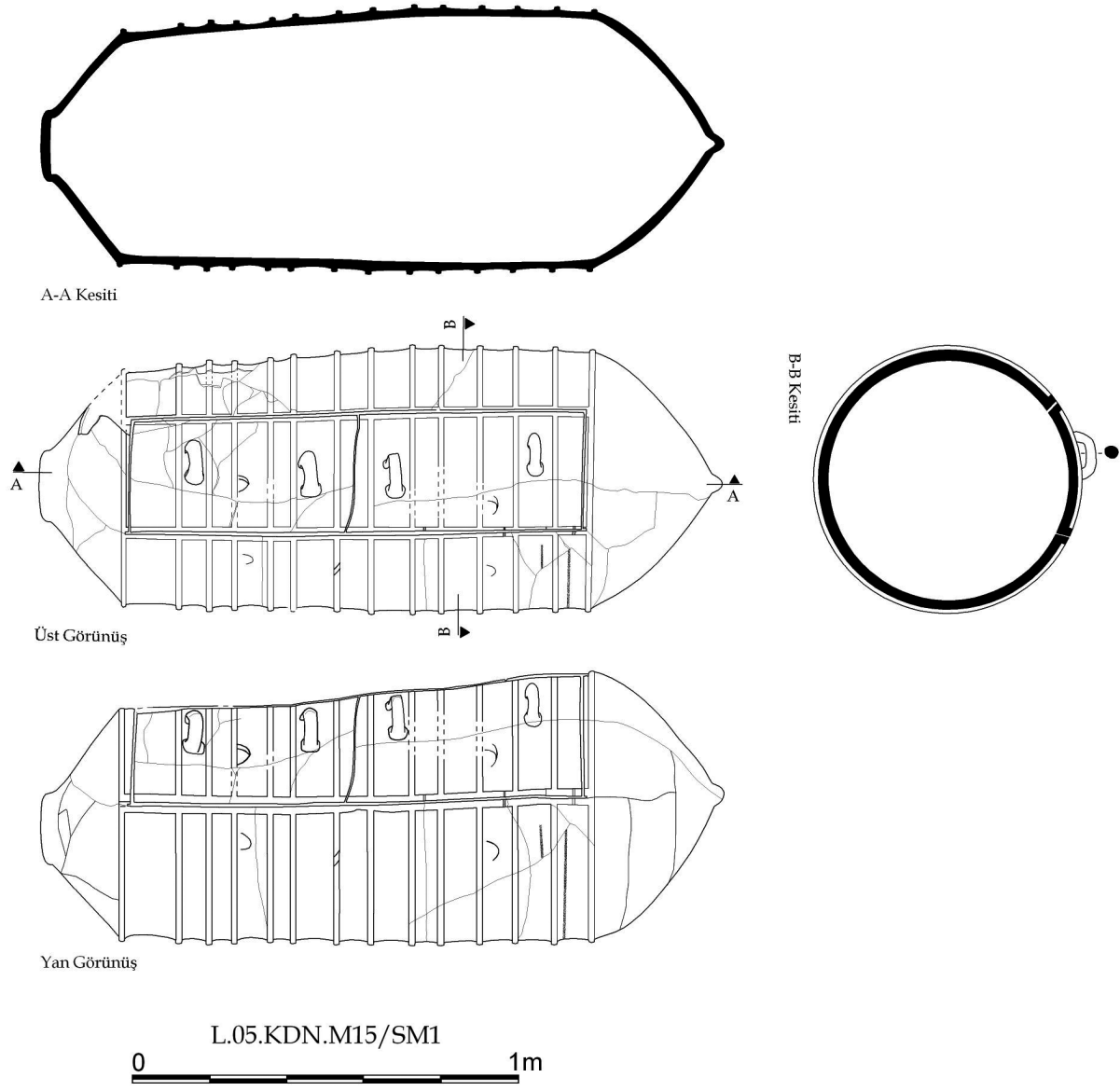
Res. 59 Kuzeydoğu Nekropolü'nden, pişmiş toprak silindirik mezarın görünüş ve kesiti
