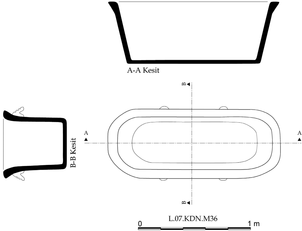
Res. 60 Kuzeydoğu Nekropolü, pişmiş toprak küvet tekne mezarın görünüş ve kesiti
