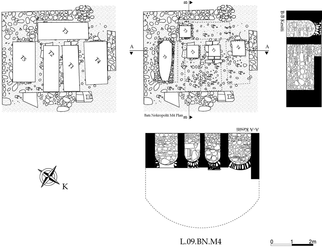
Res. 51 Batı Nekropolü'nden, tonozlu mezar odasının altına yapılan yan yana sıralı tonozlu mezar hücrelerinin plan ve kesiti (L.09.BN.M4)
