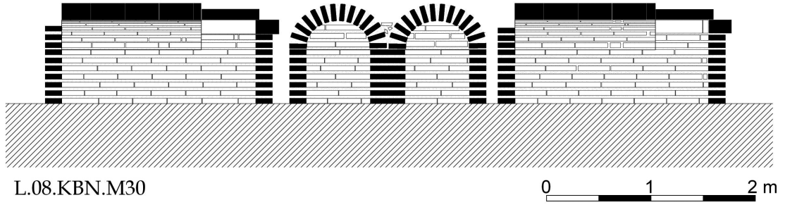
Res. 52 Kuzeybatı Nekropolü'nden, çift hücreli tuğla örgülü tonozlu mezar kesiti (L.08.KBN.M30a-b)
