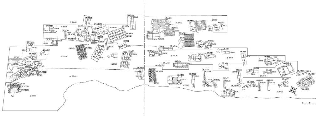
Res. 42 2008-2009 yılı Kuzeybatı Nekropolü kazı alanı planı
