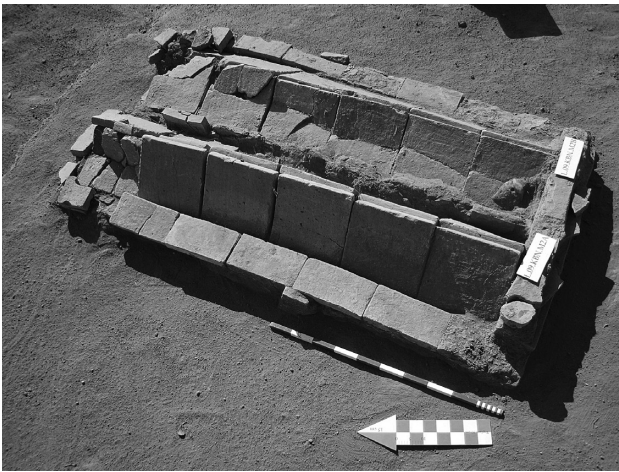
Res. 25a-b Kuzeybatı Nekropolü'nde yamaca teraslanarak yapılan tuğla örgülü ikiz tekne mezarlar (L.09.KBN.M2A-B)
