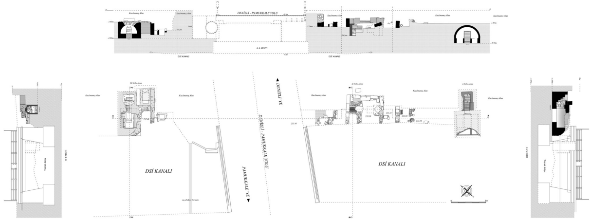
Res. 44 2013 yılı Doğu Nekropolü kurtarma kazısı ile ortaya çıkartılan mezarların planı
