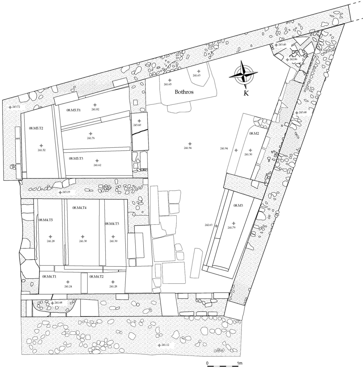
Res. 48 Kuzey Nekropolü'nden, avlu-tonozlu mezar kompleksi (2008 Yılı)
