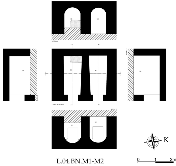
Res. 50 Batı Nekropolü'nden, yan yana sıralı olarak yapılmış tonozlu hücreli mezarların plan ve kesiti (L.04.BN.M1-M2)
