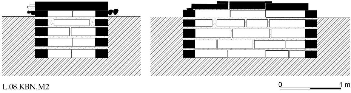
Res. 58 Kuzeybatı Nekropolü'nden, traverten örgü tekne mezarın kesiti
