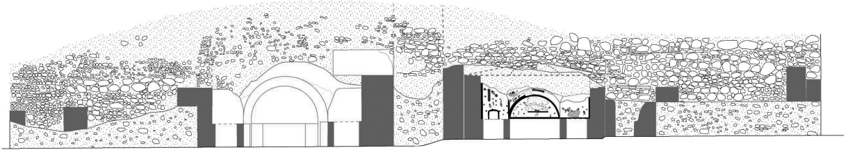
B-B Kesiti
