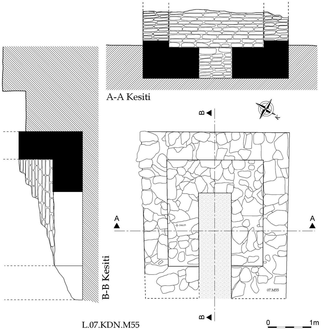
Res. 53 Kuzeydoğu Nekropolü'nden, düz çatılı mezar evin plan ve kesiti (L.07.KDN.M55)
