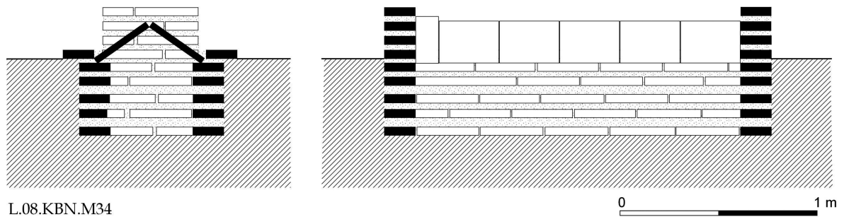
Res. 57 Kuzeybatı Nekropolü'nden, tuğla örgü tekne mezarın kesiti
