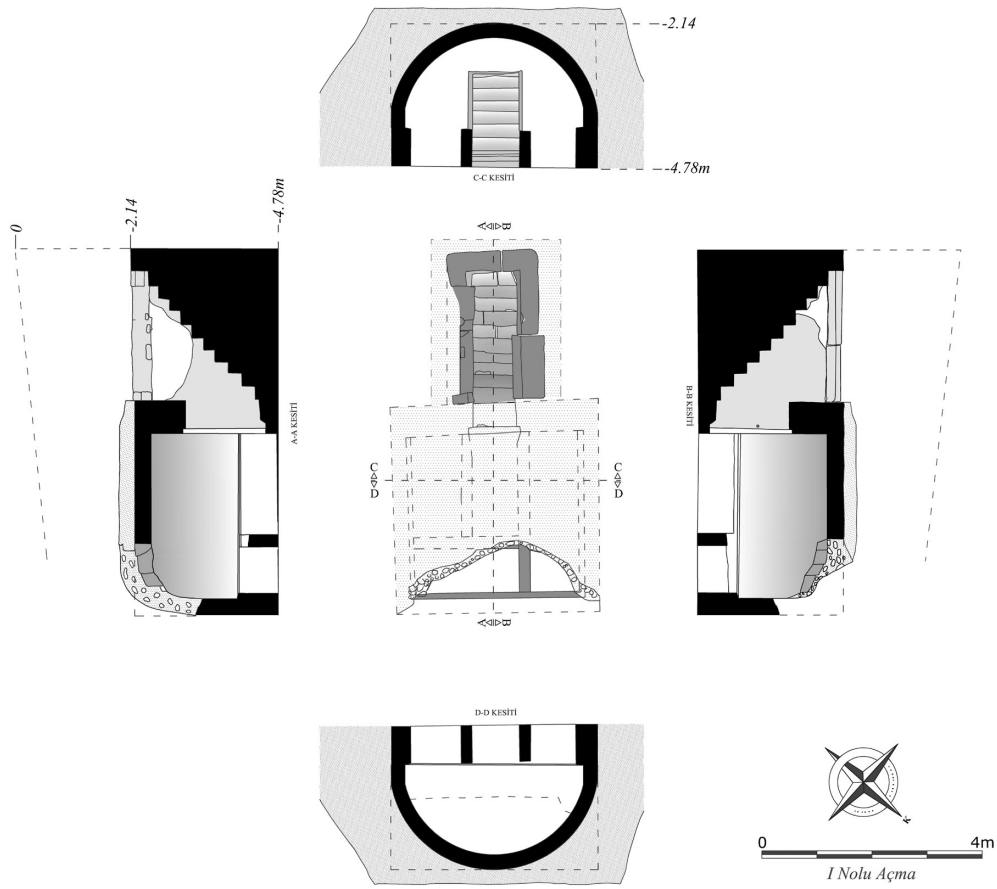
Res. 55 Doğu Nekropolü'nden, 1 no.lu hypoje mezarın plan ve kesiti
