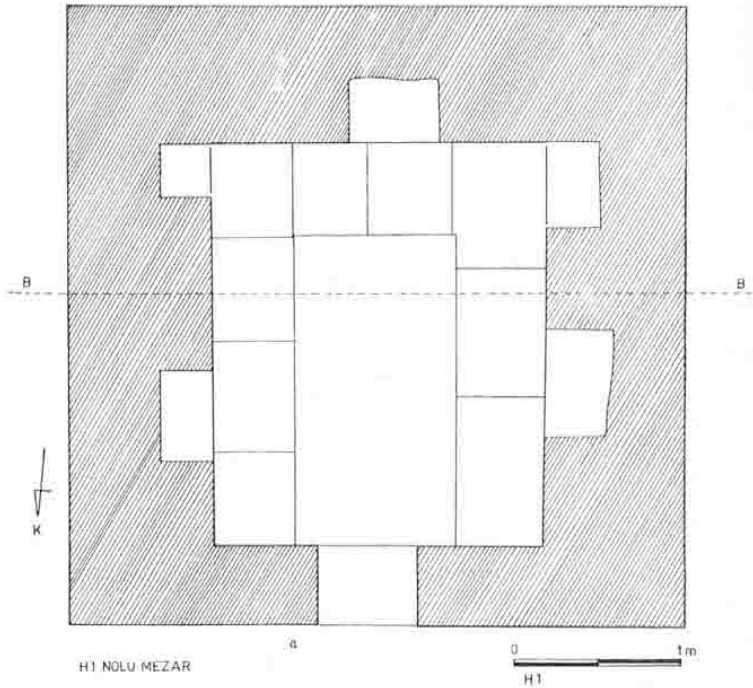
Fig 15 Hisarkale, çokgen taş duvarlı mezarın; a-planı, b-kesiti.
