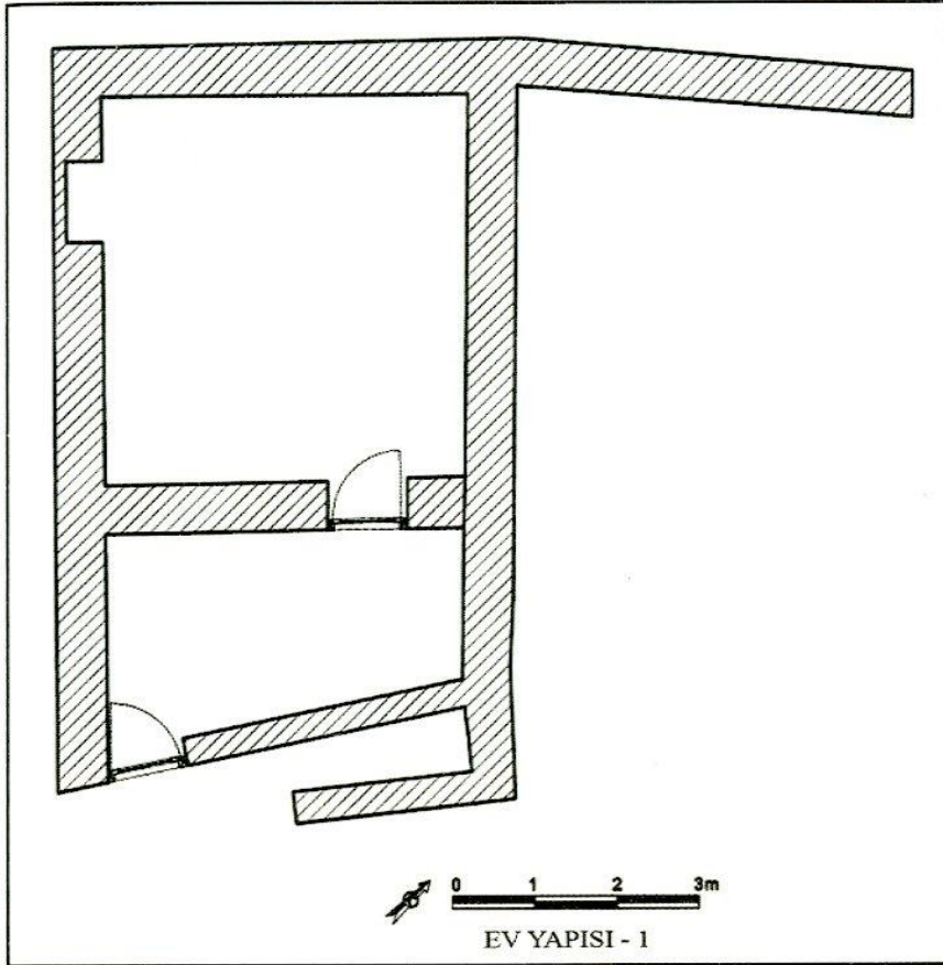
Çizim 1: Ev Yapısı 1'nin restitüsyon planı.
