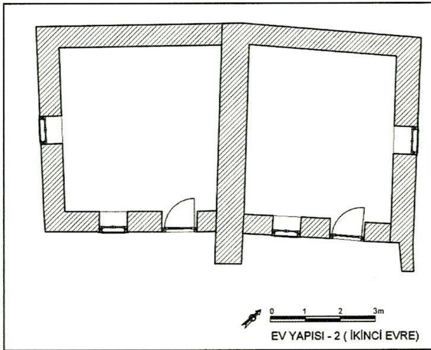
Çizim 2: Ev Yapısı 2'nin restitüsyon planı.
