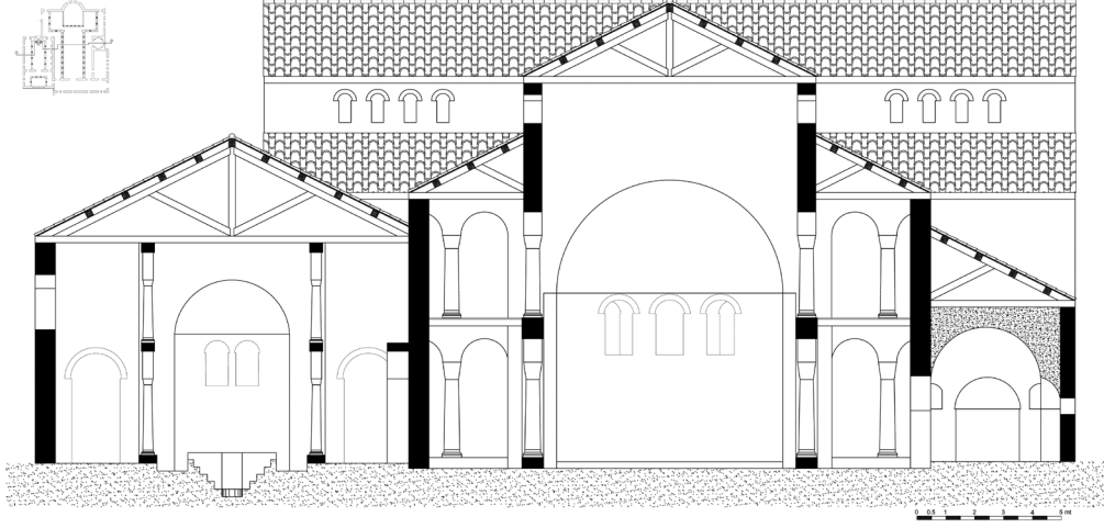
Çiz. 6 Kilise ve vaftizhane kesit restitüsyonu
