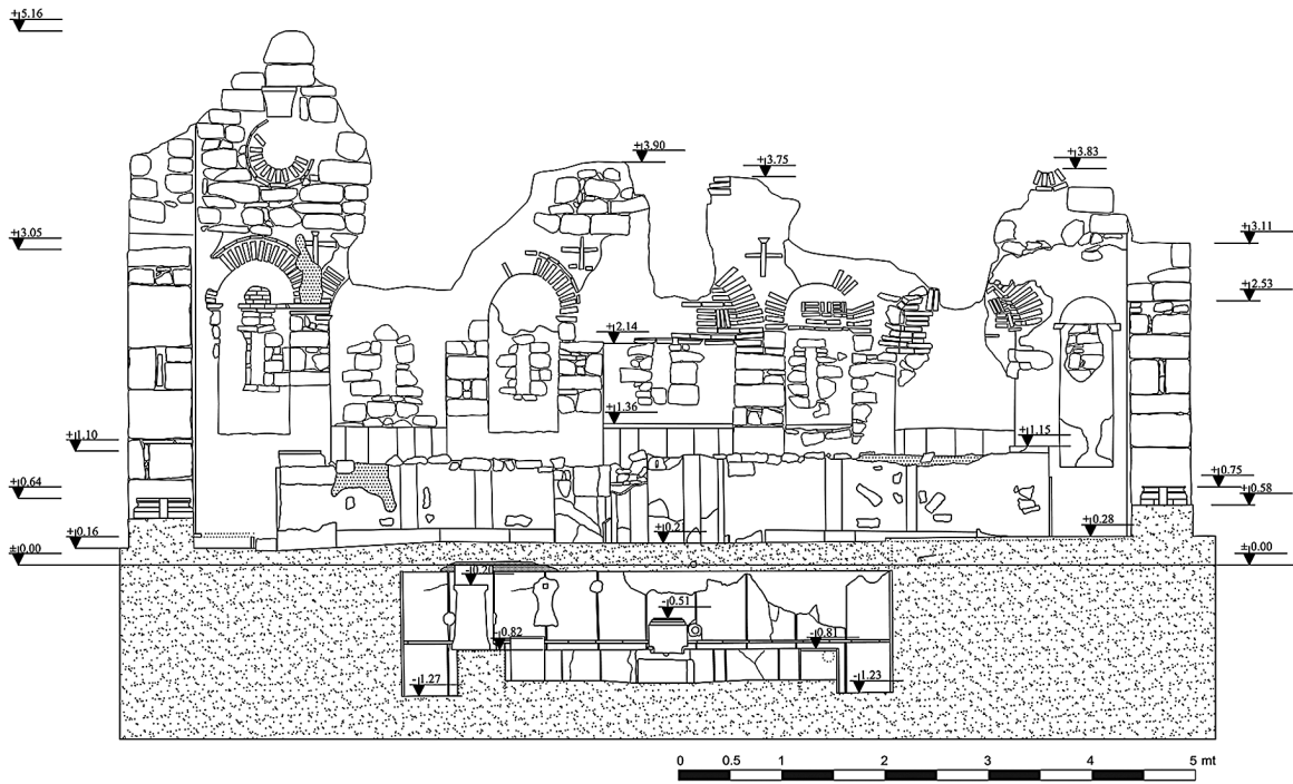
Çiz. 4 Peristylde yer alan çeşme ve implivium kesiti
