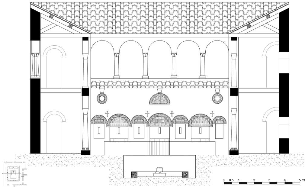
Çiz. 8 Peristyl kuzey-güney kesit restitüsyonu, batıya bakış
