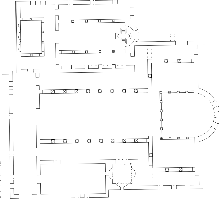
Çiz. 5 Kilise ve vaftizhane plan restitüsyonu
