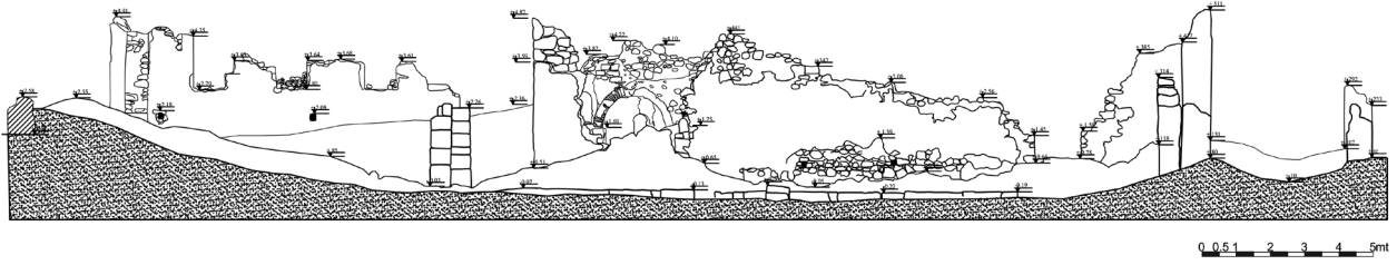
Çiz. 2 Kilise doğu-batı kesiti, güneye bakış
