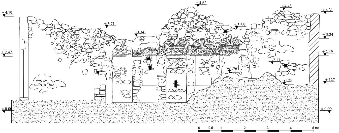
Çiz. 3 Vaftizhane vestibulum batı duvarı görünüşü
