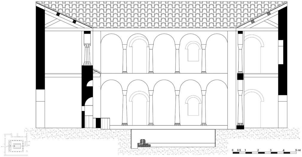
Çiz. 7 Peristyl doğu-batı kesit restitüsyonu, kuzeye bakış
