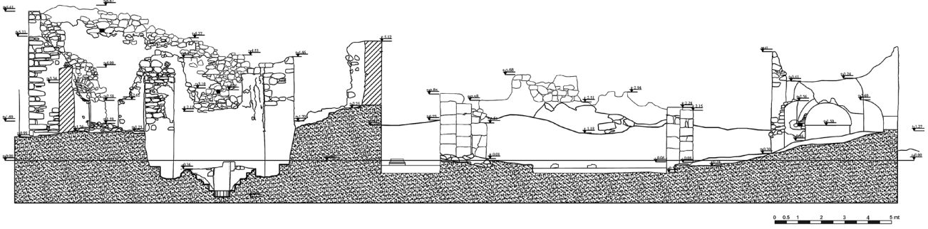
Çiz. 1 Kilise ve vaftizhane kuzey-güney kesiti, doğuya bakış
