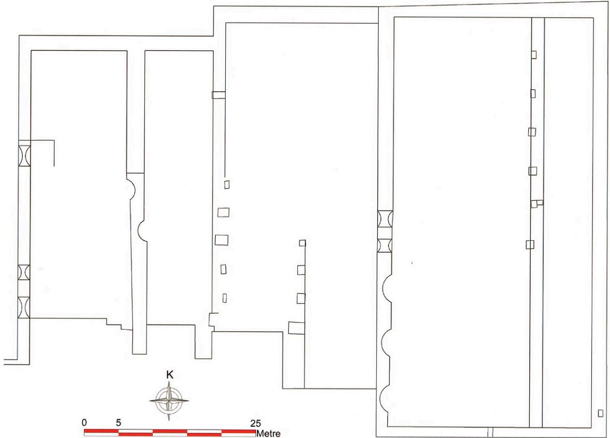
Fig. 4 Tripolis Roma Hamamı (Büyük Hamam) Planı (B. Duman, Tripolis kazı arşivi)
