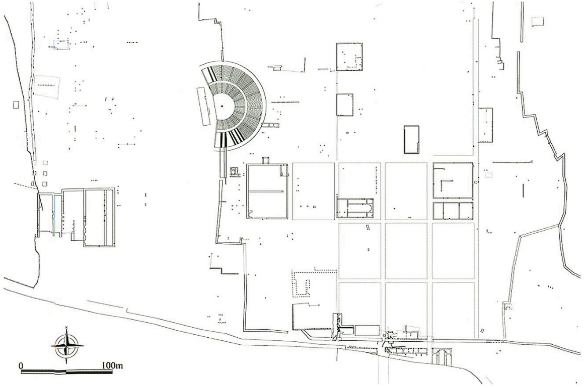
Fig. 1 Hamam ve kent yerleşim planı (Duman 2013, 186, Fig. 6)
