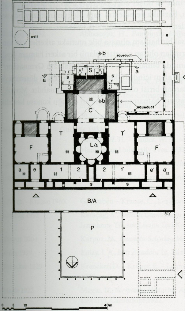
Çiz. 1 Lambaesis Askeri Hamamı (Yegül 1992, 216, Fig. 244)
