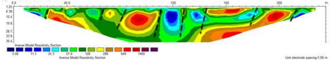
Şekil 5. 5: Profil-1 özdirenç tomografi kesiti.
