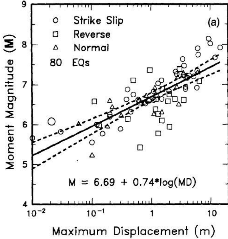
řekil 5. 20: Wells ve Coppersmith (1994)'ün maksimum yer deđiřtirme ile moment magnitud arasındaki bađlantısı.
