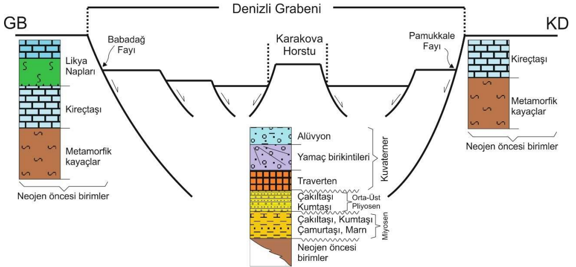
Şekil 3. 4: Denizli Grabeni'nin genel görünümü ve stratigrafisi (Hançer 2019).
