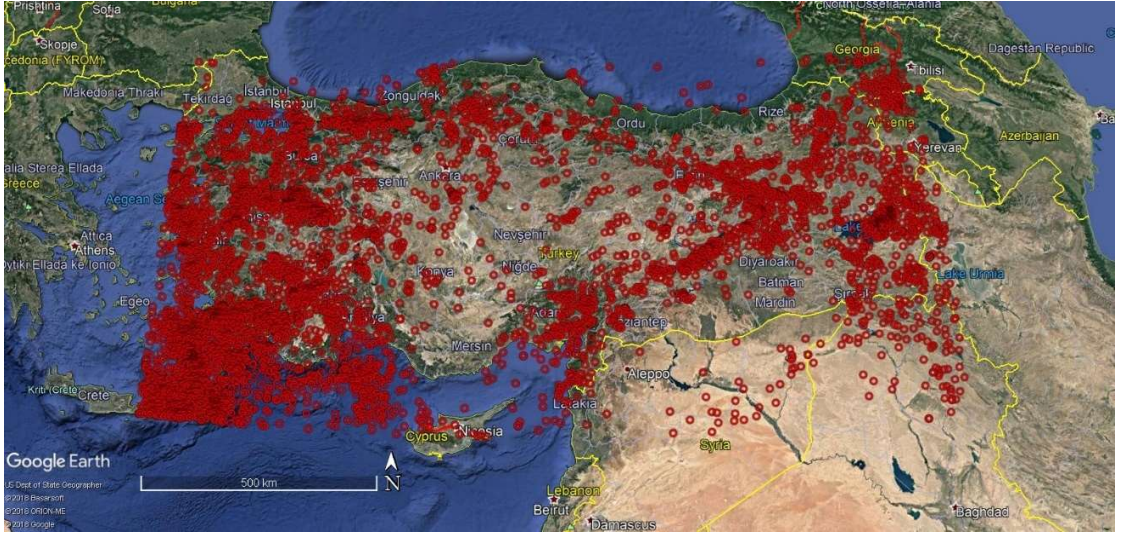
Şekil 4. 1: Türkiye geneli M>4 olan aletsel dönemde meydana gelmiş deprem episantırları (KOERİ).
