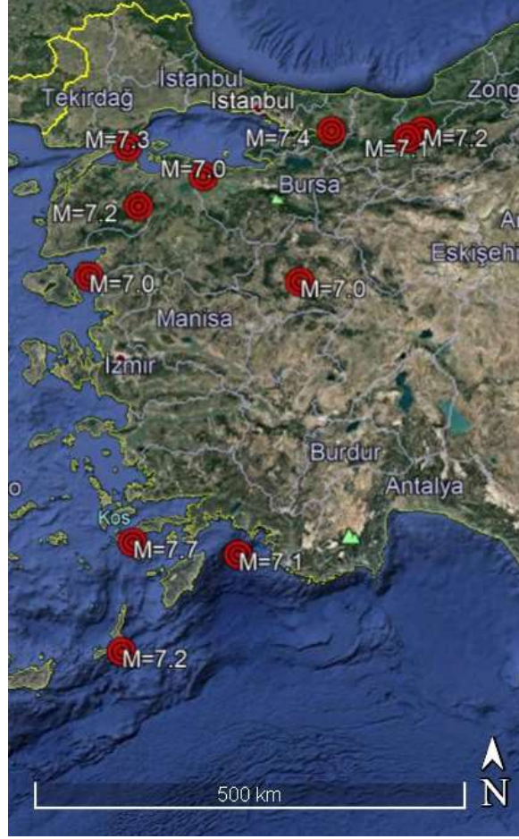
Şekil 4. 6: Batı Anadolu'da aletsel dönemde M > 7.0 olan depremler (KOERİ)
