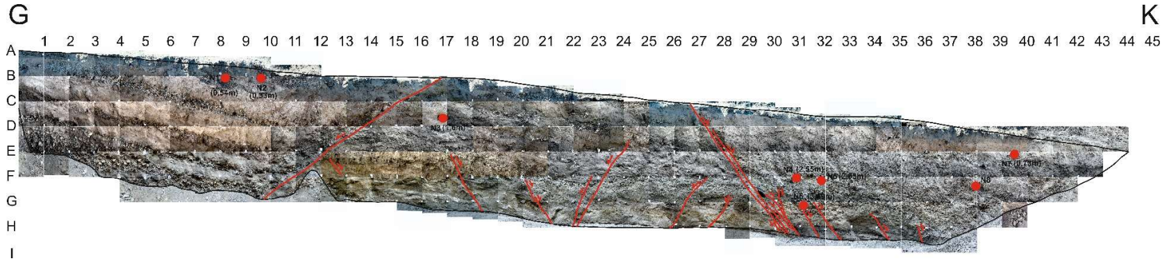
Şekil 5. 13: T1 hendeği batı duvarının mozayik fotoğrafı.
