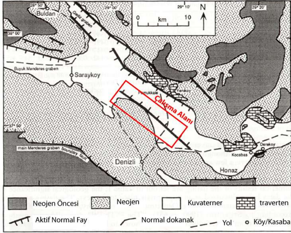
Şekil 3. 5: Çalışma alanı ve çevresinin jeoloji haritası (MTA 1964).
