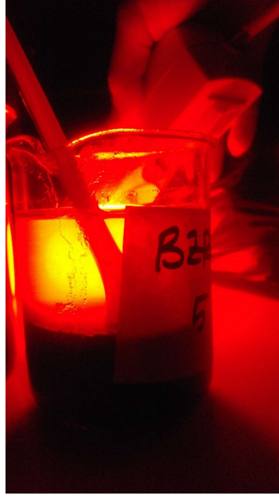
Şekil 5. 19: Karanlık oda koşullarına uygun laboratuvarında numune işleme süreci.
