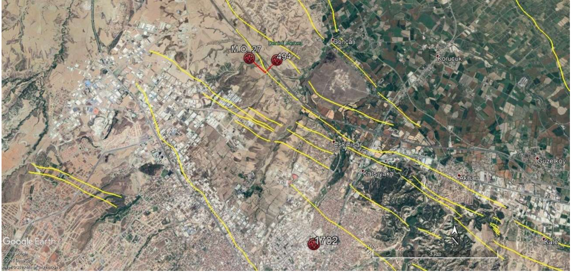
Şekil 4. 10: Çalışma alanında ve yakın çevresinde meydana gelmiş tarihsel deprem episentr noktaları (Tan ve diğ. 2008; MTA 2012).
