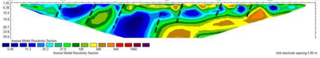
Şekil 5. 6: Profil-2 özdirenç tomografi kesiti.
