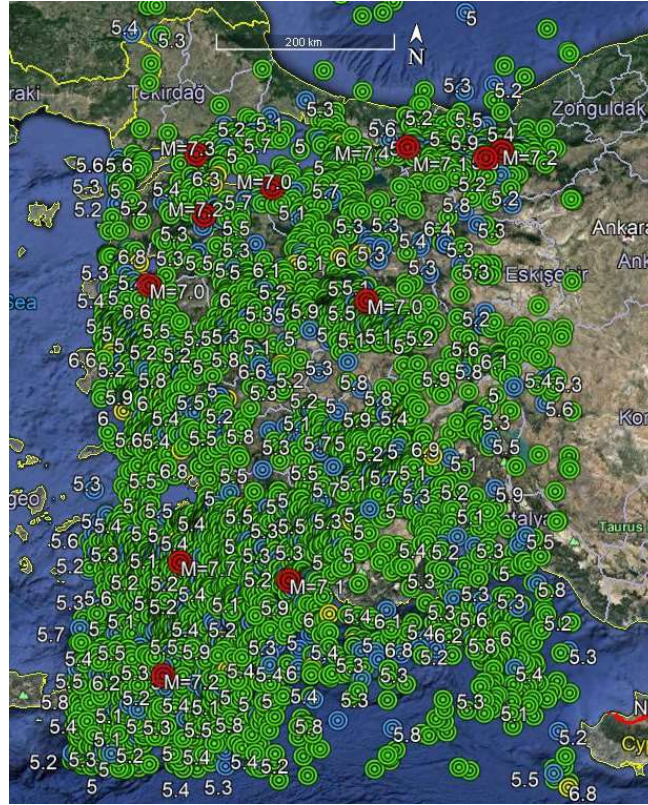
Şekil 4. 4: Batı Anadolu'da 1900 yılından günümüze kadar meydana gelmiş olan M>4.0 olan deprem episantrları (KOERİ)
