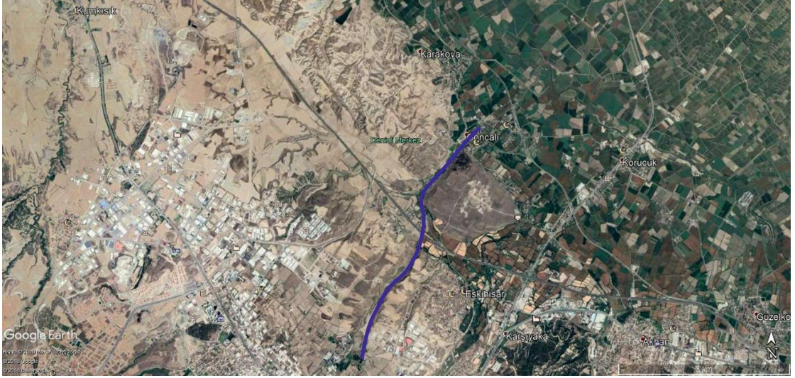
Şekil 4. 9: Gümüşçay deresinin günümüzdeki yatağı.
