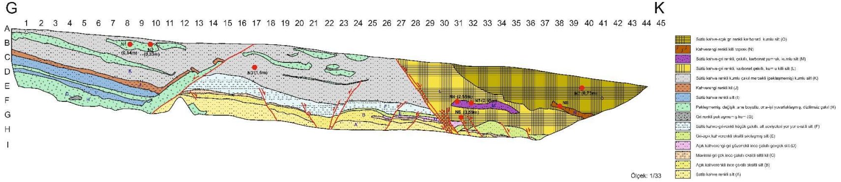
Şekil 5. 12: T1 hendeğinin batı duvarına ait enine jeolojik kesit (ölçek 1/33).
