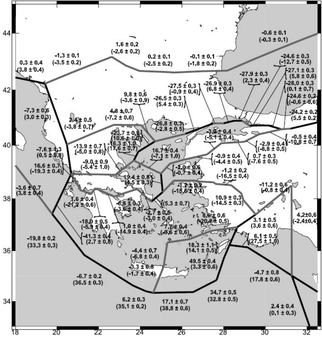
Şekil 3. 3: Batı Anadolu'daki fayların kayma hızlarını gösteren harita. Üstteki sayılar (parantezsiz olanlar) doğrultu atım hızlarını (pozitif değerler sol yönlü), alttaki sayılar (parantez içinde olanlar) normal atım hızlarını (pozitif değerler yaklaşım) gösterir harita (Reilinger ve diğ. 2006).
