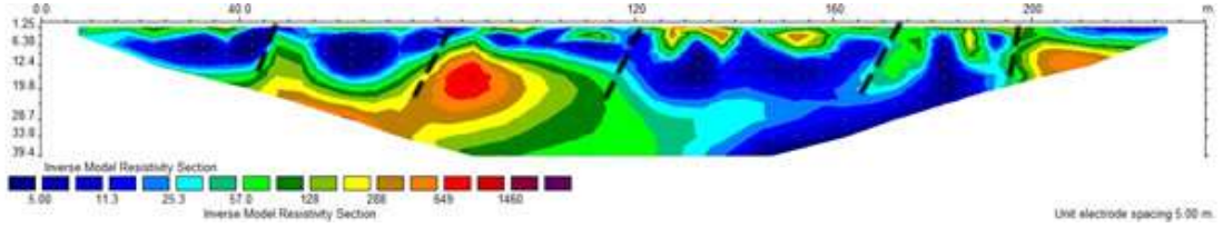
Şekil 5. 7: Profil-3 özdirenç tomografi kesiti.
