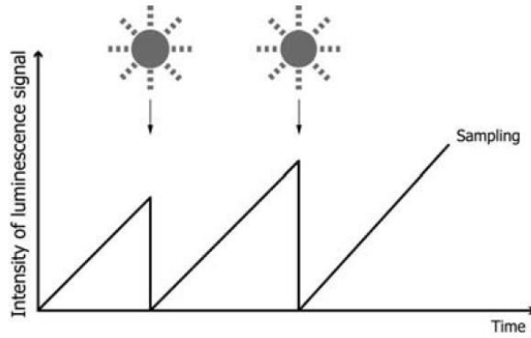
Şekil 5. 15: Paleodoz miktarının sıfırlanma süreci.
