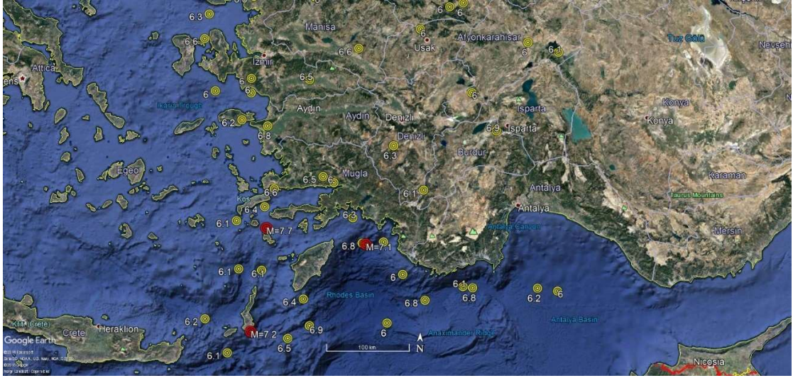
Şekil 4. 5: Fethiye-Burdur fayı üzerinde meydana gelmiş M>6 olan deprem episantr noktaları (KOERİ).
