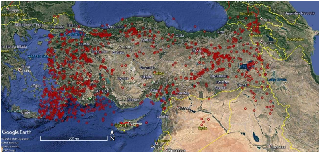
Şekil 4. 2: Türkiye geneli M>5 olan aletsel dönemde meydana gelmiş deprem episantırları (KEORİ).
