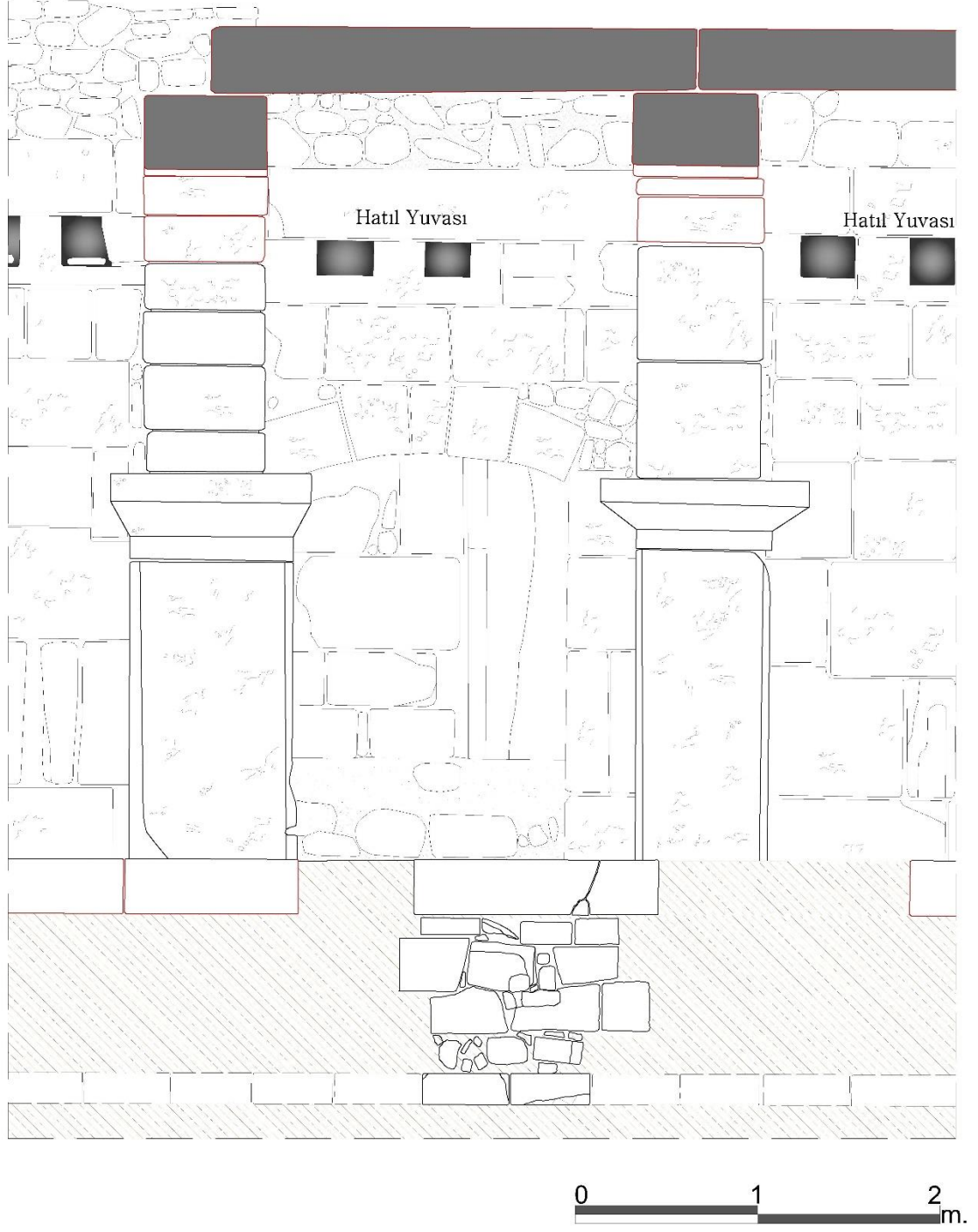
Fig. 10: Kemerli Yapı'daki Sondaj Çalışması Çizimi
