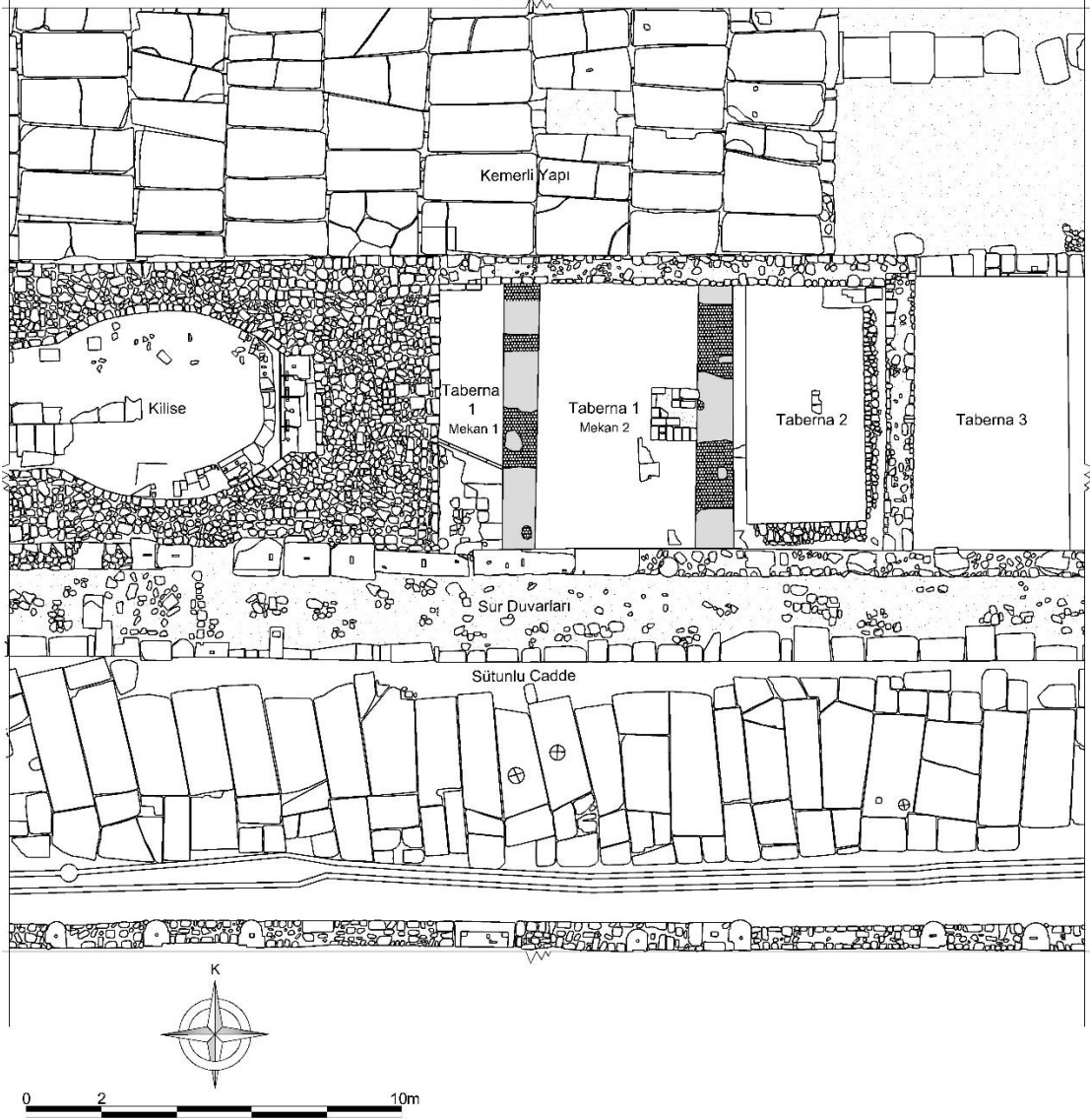
Fig. 12: Tabernaların ve Çevresindeki Yapıların Planı
