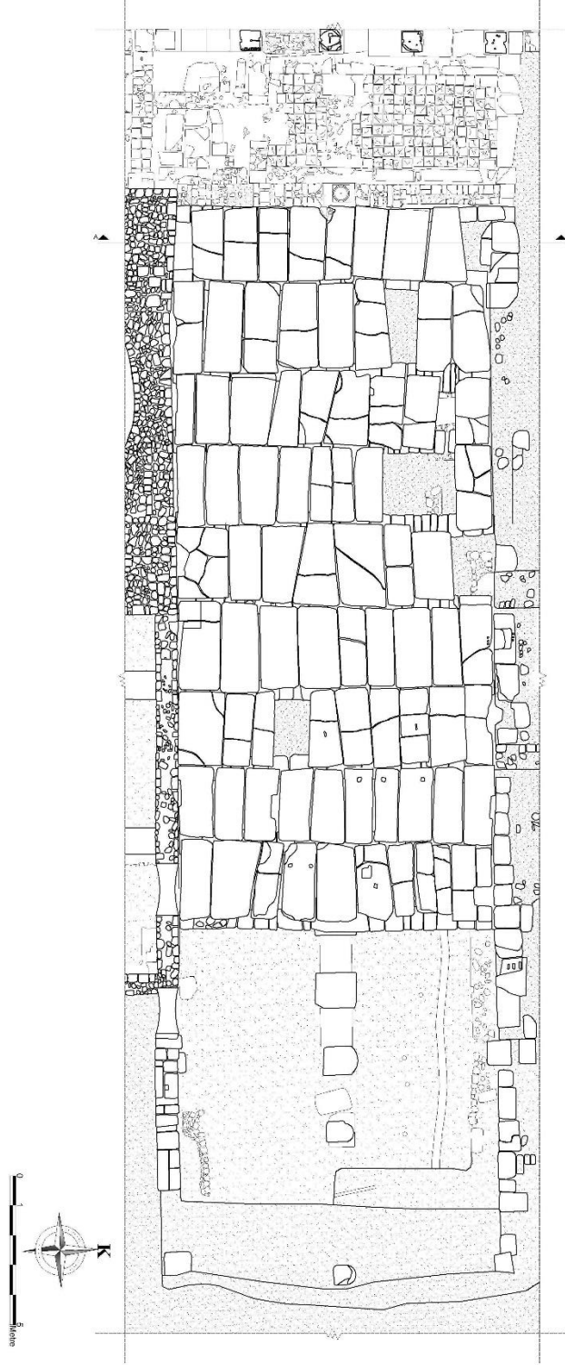
Fig. 9: Kemerli Yapı'nın Üstten ve Batı Cepheden Görünüş Çizimi
