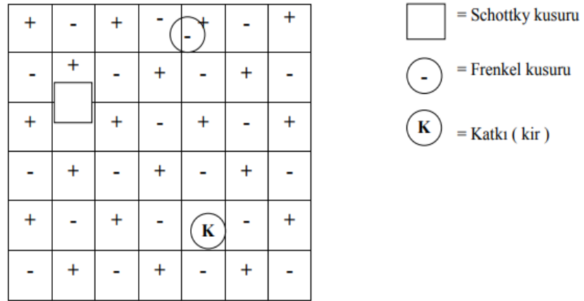
Şekil 1.1 Değişik tipte kristal kusurları 12 .
