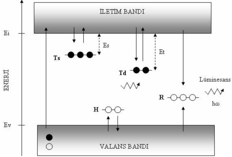
Şekil 1.2 Band modeline göre lüminesans mekanizmasının enerji diyagramı 13 .
