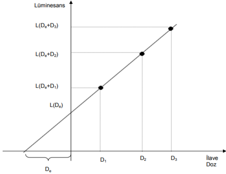
Şekil 2.1 MAAD yöntemiyle eşdeğer doz hesabı için ilave dozlar ile lüminesans sayımları arasında çizilen grafik 38 .
