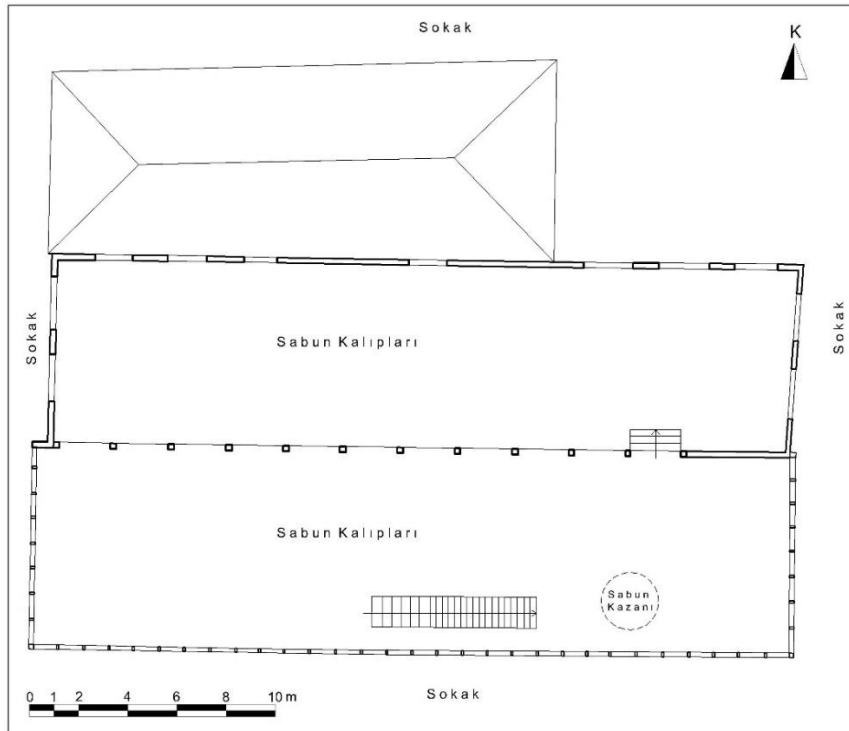
Çizim 40: Ayvalık Cömertler Sabunhanesi Birinci Kat Rölöve Plânı, 1976 (Ayvalık Belediyesi Arşivinden İşlenerek)
