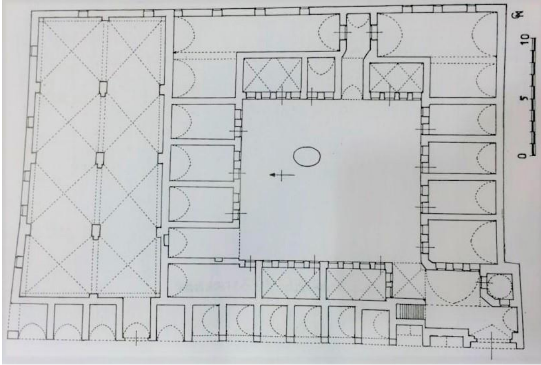
Çizim 97: Gaziantep Elbeyli Sabunhanesi Zemin Kat Plânı (N. Çam, age, s. 449)
