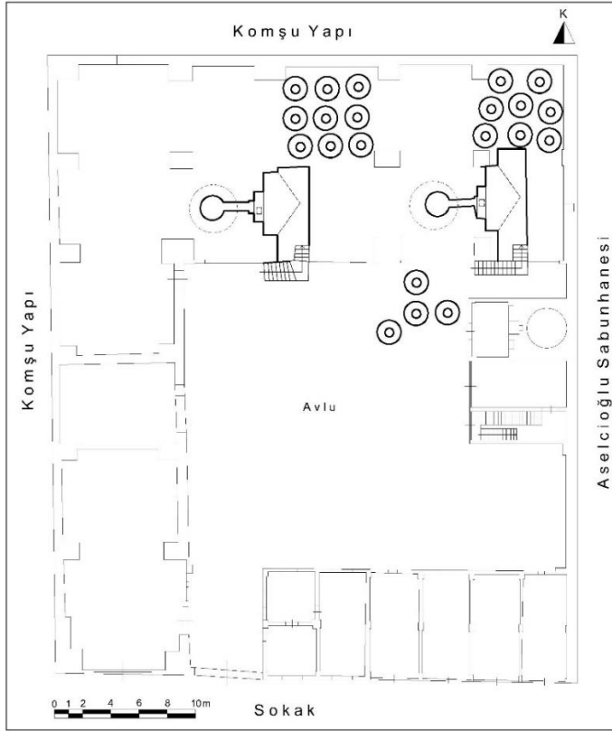
Çizim 79: Antakya Hasan Ökten Sabunhanesi Ocaklık Plânı (Hatay KVKBKM Arşivinden İşlenerek)
