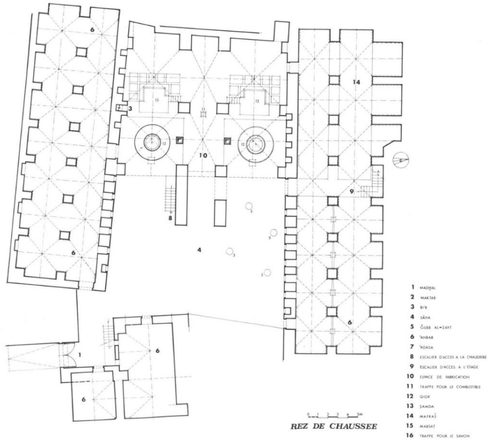
Çizim 12: Halep Zenabîli Sabunhanesi Zemin Kat Plânı (T. Grandin, agm, P. XA)
