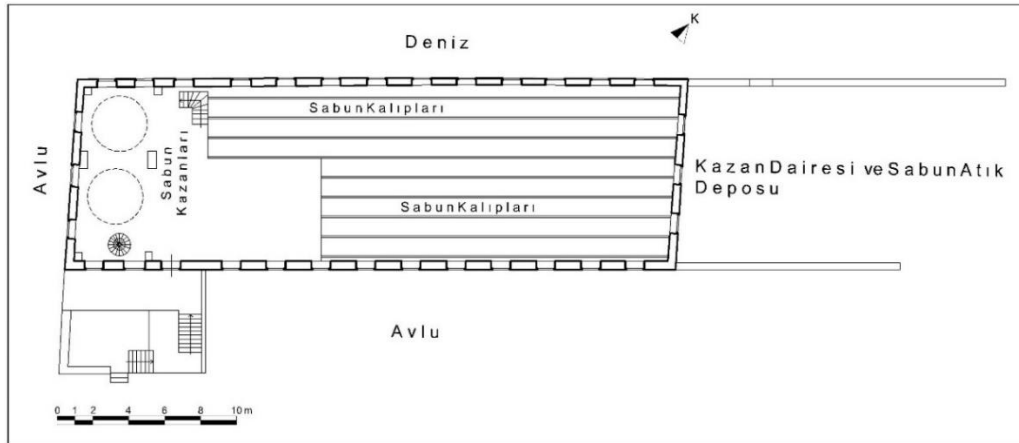
Çizim 34: Ayvalık Fazıl Doğan Sabunhanesi Birinci Kat Plânı (Bursa KVKBKM Arşivinden İşlenerek)
