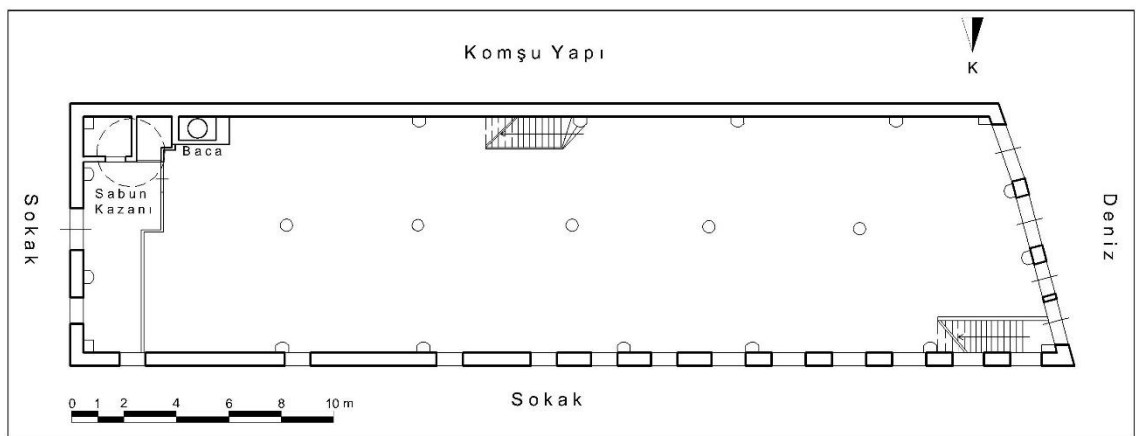
Çizim 24: Ayvalık Erman Sabunhanesi Zemin Kat Plânı (Ayvalık Belediyesi Arşivinden İşlenerek)
