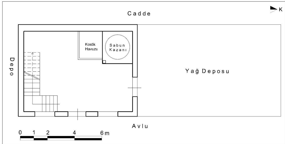
Çizim 53: Edremit Ali Rıza Karagözoğlu Sabunhanesi Zemin Kat Plânı (M. Çiftyürek)
