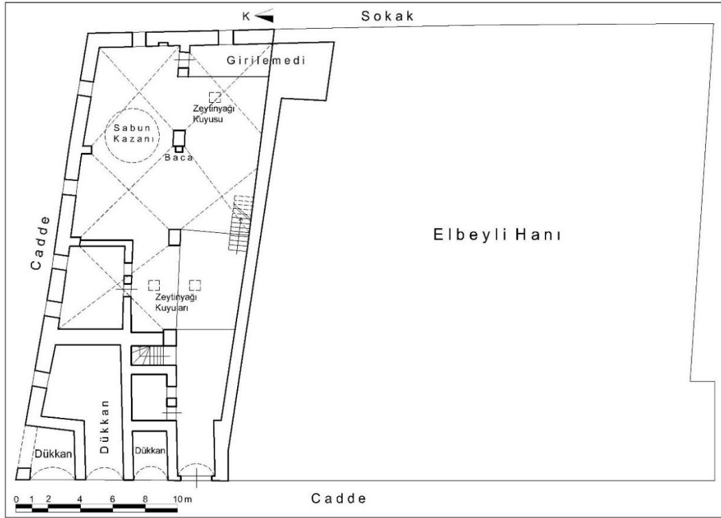
Çizim 98: Gaziantep Elbeyli Sabunhanesi Zemin Kat Plânı (Gaziantep KVKBKM Arşivinden İşlenerek)
