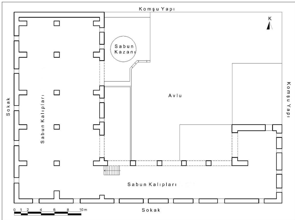
Çizim 110: Nizip Fındıklar Sabunhanesi Birinci Kat Plânı (H. Eker, YLT'den İşlenerek)
