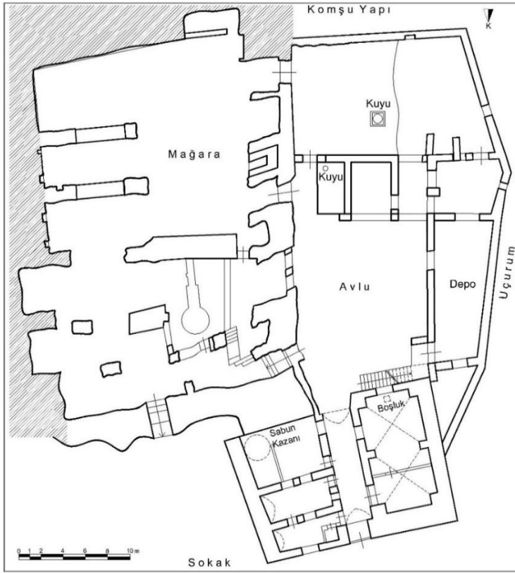
Çizim 102: Birecik Mıstıkoğlu Sabunhanesi Zemin Kat Plânı (M. Çiftyürek)
