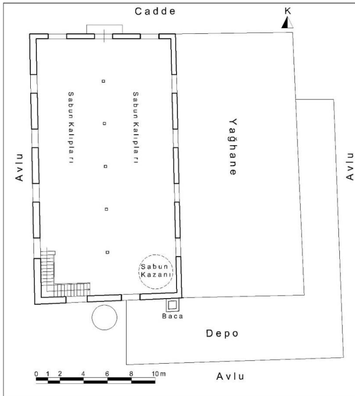
Çizim 31: Burhaniye Yağcı Sabunhanesi Birinci Kat Plânı (M. Çiftyürek)
