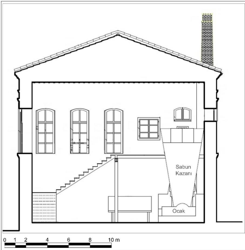
Çizim 51: Burhaniye Hüsnü Tolun Sabunhanesi Ocak ve Kazan Kesiti (D. Akın, YLT'den İşlenerek)
