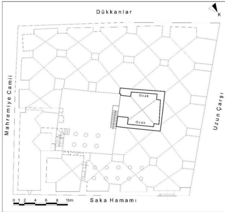
Çizim 74: Antakya Haytoğlu Sabunhanesi Ocaklık Plâni (Hatay KVKBKM Arşivinden İşlenerek)
