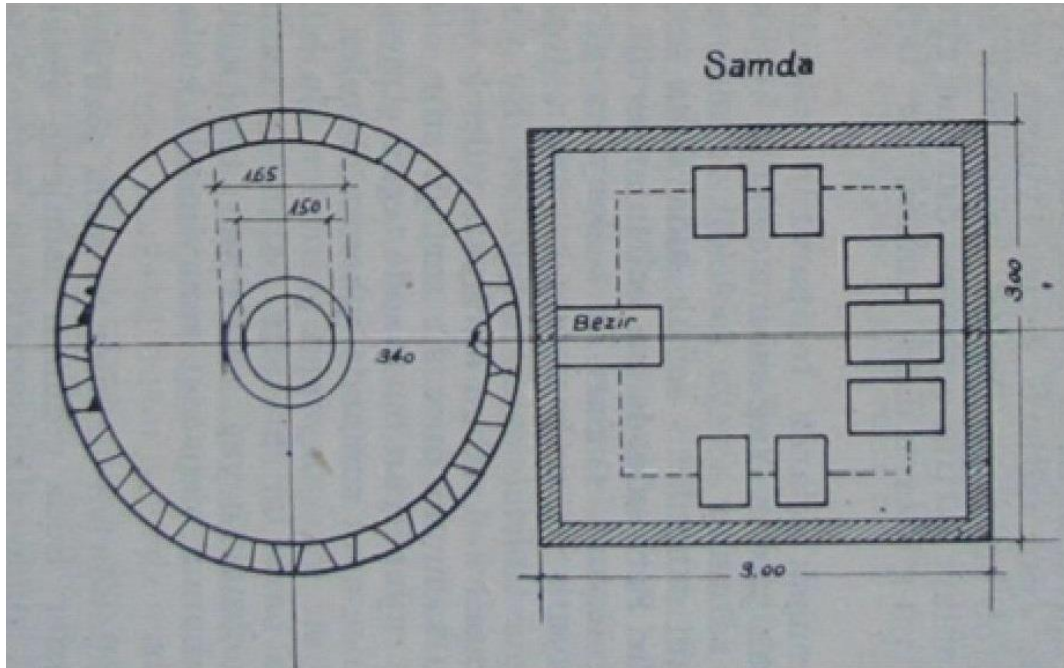
Çizim 72: Antakya Sabunhanelerindeki Taş Sabun Kazanı ve Kostik Havuzu (Samda) Plânı (TSOTBB, age, s. 11)
