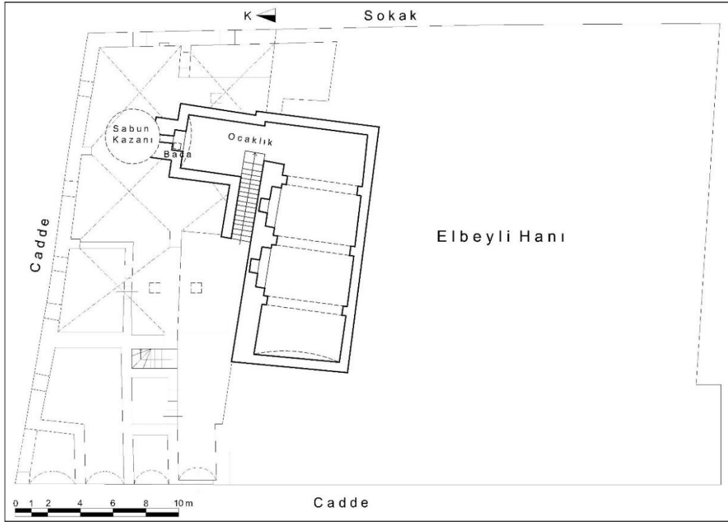
Çizim 99: Gaziantep Elbeyli Sabunhanesi Ocaklık Plânı (Gaziantep KVKBKM Arşivinden İşlenerek)
