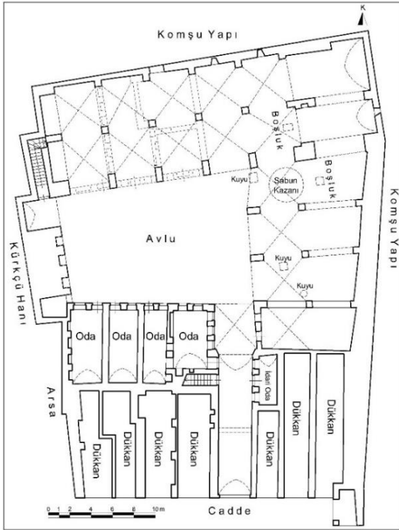
Çizim 94: Gaziantep Kürkçü Sabunhanesi Zemin Kat Plânı (Gaziantep KVKBKM Arşivinden İşlenerek)
