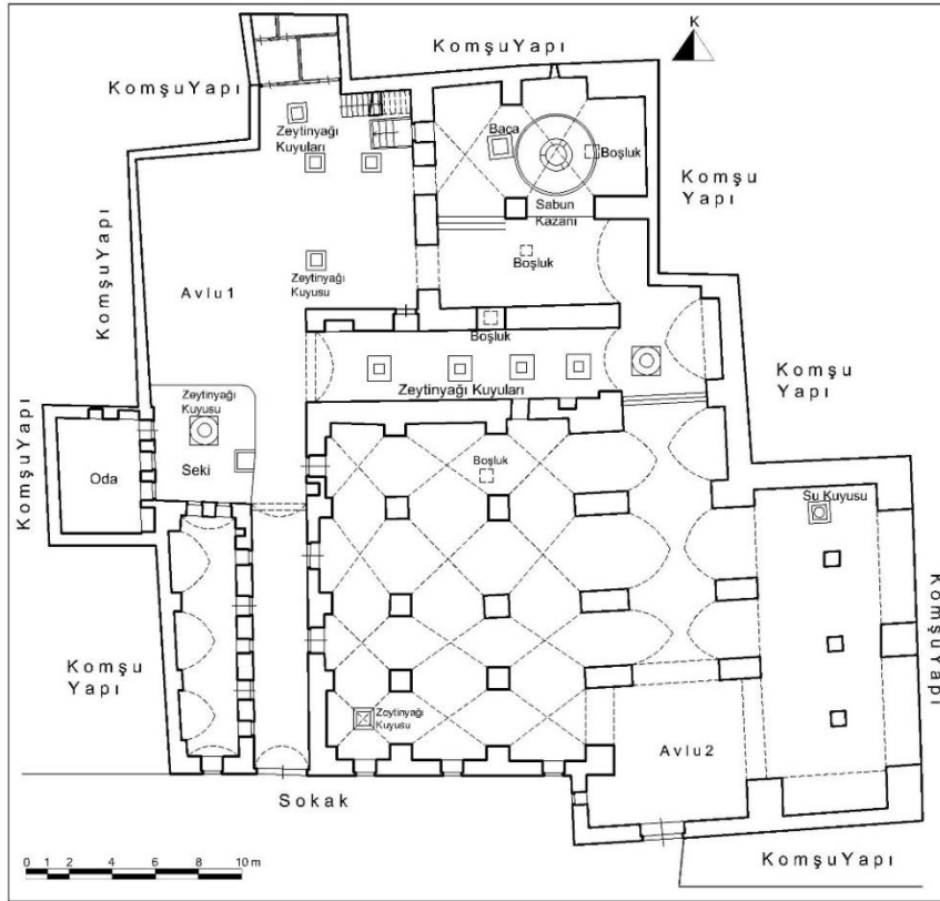
Çizim 114: Kilis Kalaycılar Sabunhanesi Zemin Kat Plânı (Gaziantep KVKBKM Arşivinden İşlenerek)
