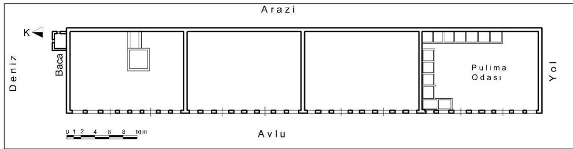
Çizim 60: Ayvalık Gümüşlü Eminzade Sabunhanesi Zemin Kat Plânı (M. Çiftyürek)
