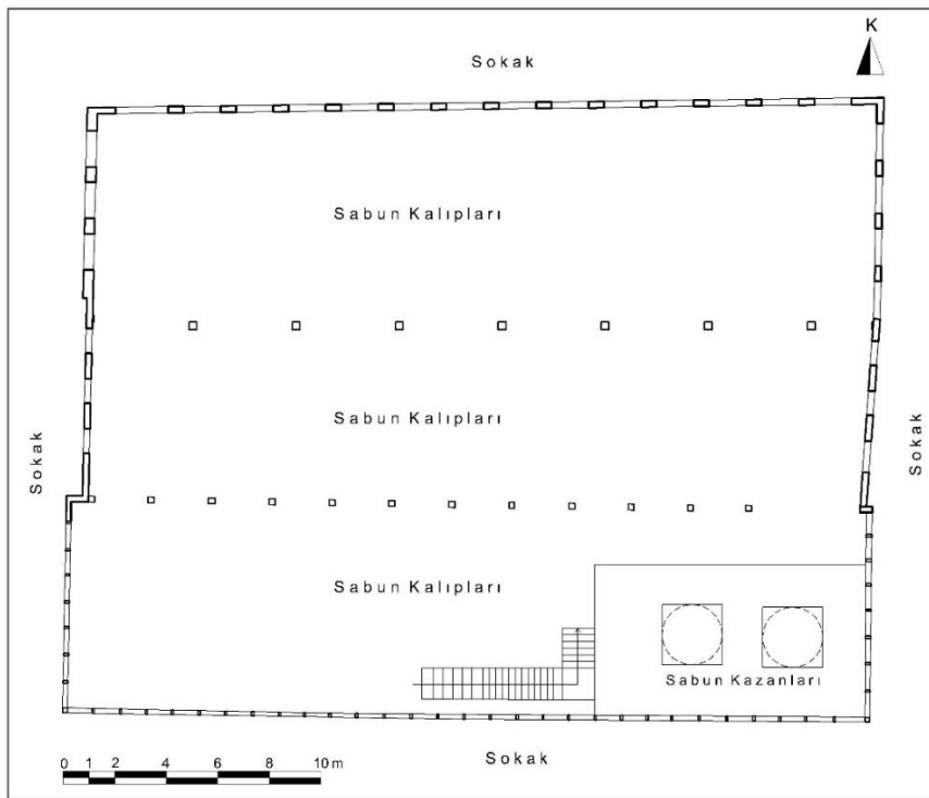
Çizim 42: Ayvalık Cömertler Sabunhanesi Birinci Kat Plânı (M. Çiftyürek)
