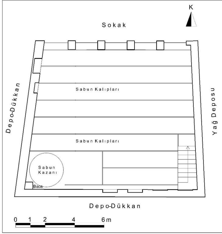
Çizim 131: Ayvalık Karşınlar Sabunhanesi Birinci Kât Plânı (M. Çiftyürek)
