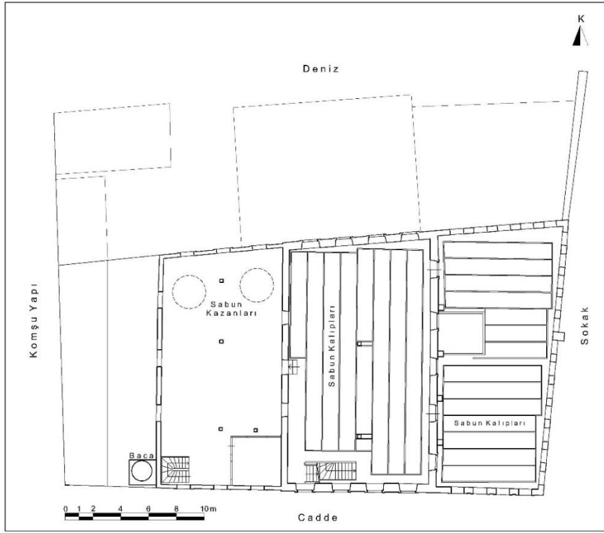
Çizim 123: Ayvalık Sezai Ömer Madra Sabunhanesi Birinci Kat Plânı (Bursa KVKBKM Arşivinden İşlenerek)
