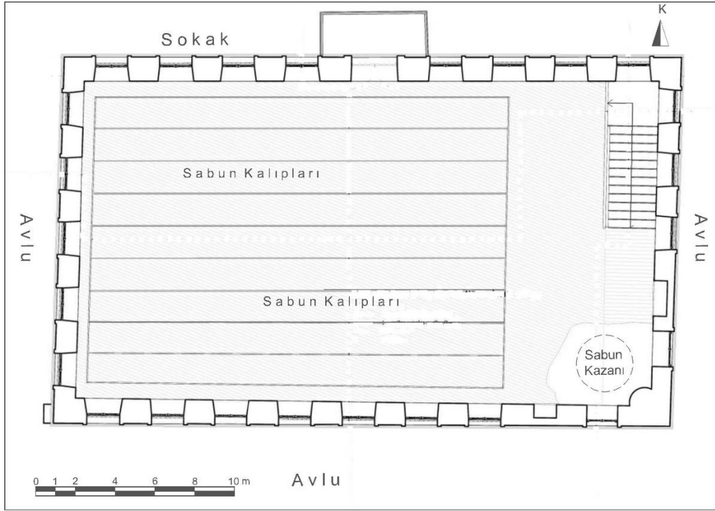
Çizim 50: Burhaniye Hüsnü Tolun Sabunhanesi Birinci Kat Plânı (D. Akın, YLT'den İşlenerek)
