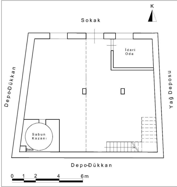
Çizim 129: Ayvalık Karşınlar Sabunhanesi Zemin Kat Plânı (M. Çiftyürek)
