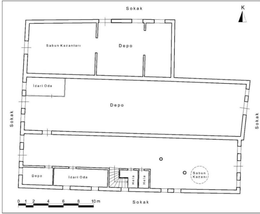
Çizim 39: Ayvalık Cömertler Sabunhanesi Zemin Kat Rölöve Plânı, 1976 (Ayvalık Belediyesi Arşivinden İşlenerek)
