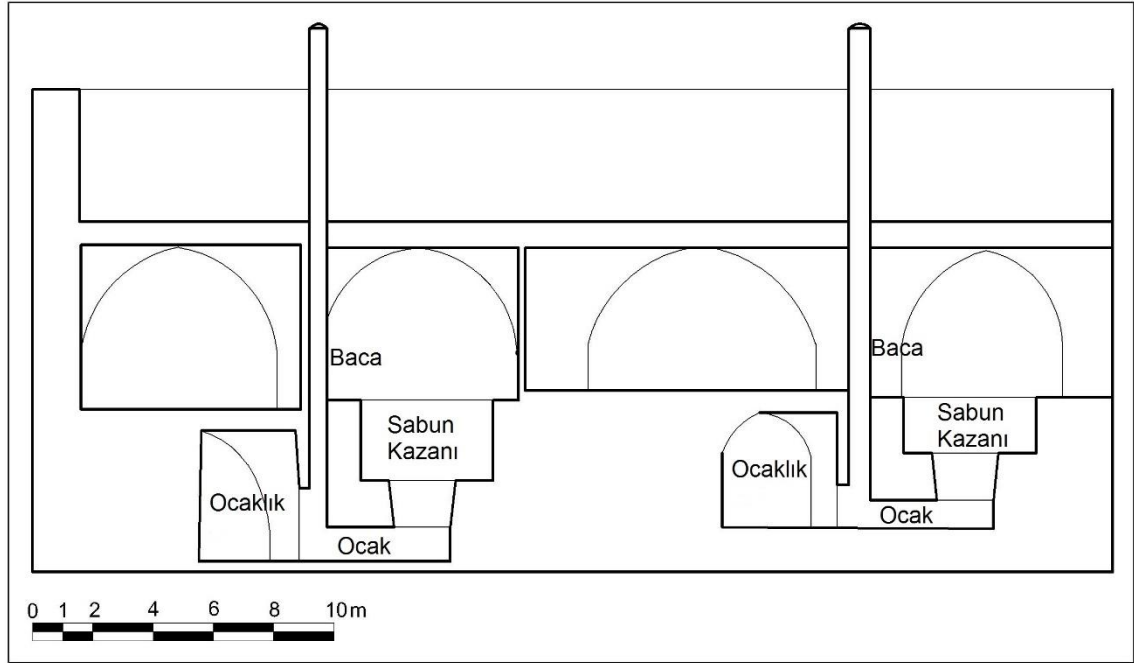
Çizim 80: Antakya Hasan Ökten Sabunhanesi Ocak, Sabun Kazanı ve Baca Kesiti (Hatay KVKBKM Arşivinden İşlenerek)
