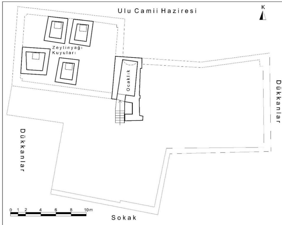
Çizim 120: Kahramanmaraş Cumhuriyet Hanı Sabunhanesi Ocaklık Plânı (Gaziantep KVKBKM Arşivinden İşlenerek)
