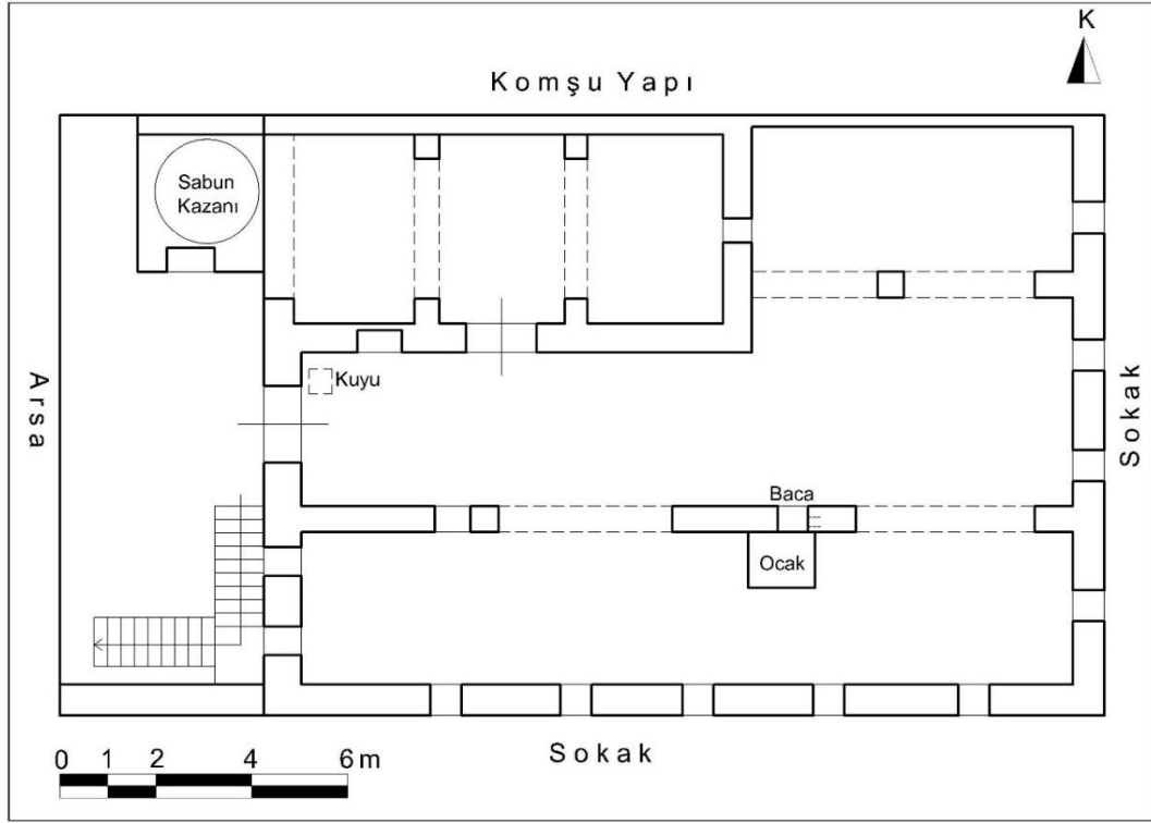
Çizim 111: Nizip Okanlar Sabunhanesi Zemin Kat Plânı (M. Çiftyürek)
