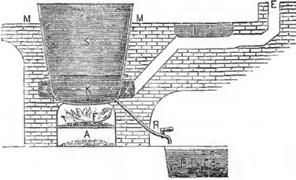
Çizim 3: Ateş Sistemi İle Çalışan Kazan Örneği (P. Wiltner-C. Calmels, age, 1914, s. 47)
