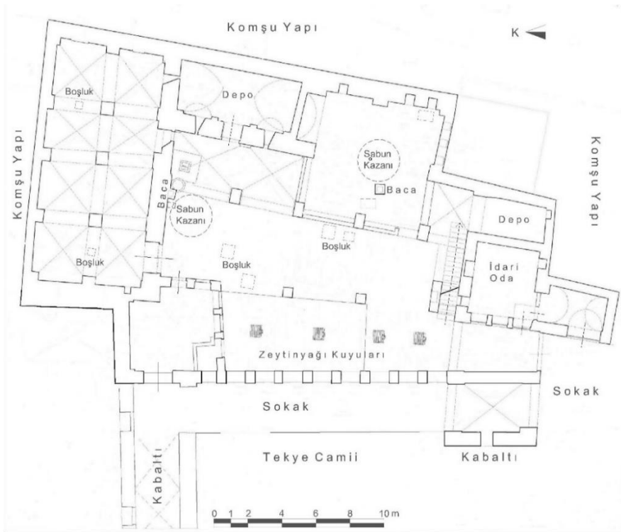
Çizim 106: Kilis Muharrem Bey Sabunhanesi Zemin Kat Plânı (F.R.Polat, YLT'den İşlenerek)
