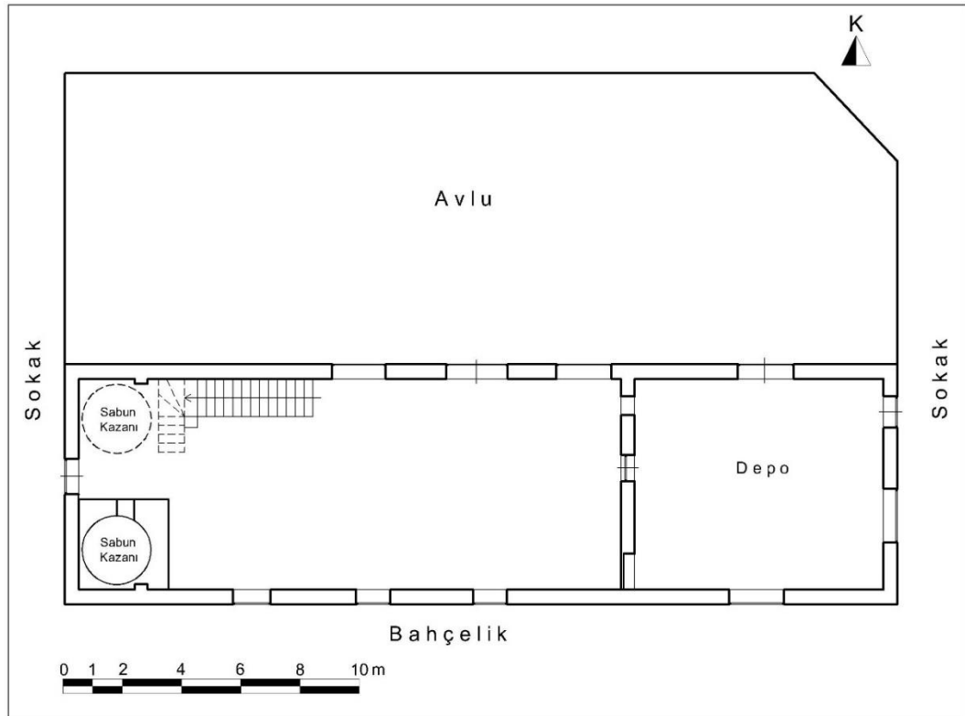
Çizim 64: Ayvacık Küçükkuyu Burnaz Sabunhanesi Zemin Kat Plânı (M. Çiftyürek)
