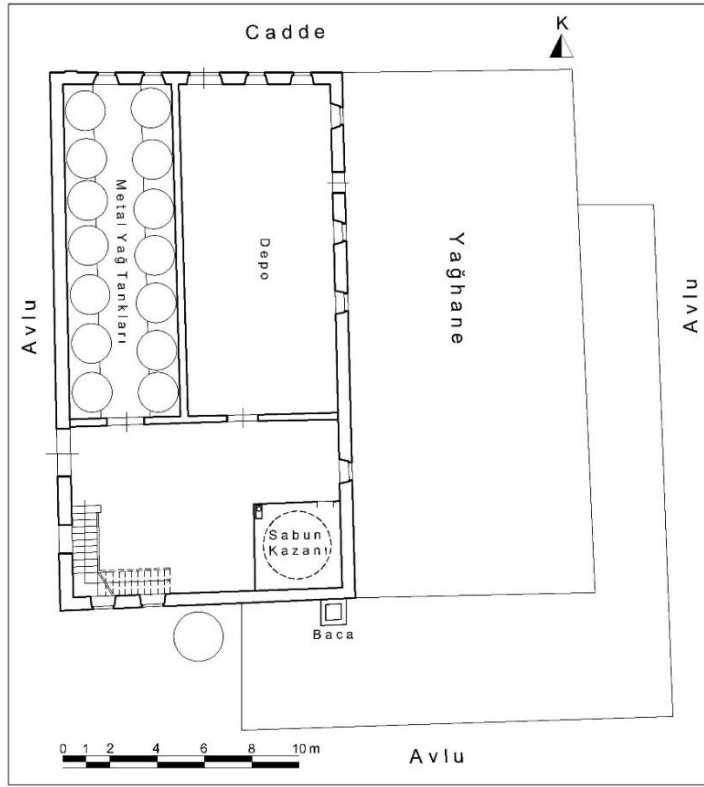
Çizim 30: Burhaniye Yağcı Sabunhanesi Zemin Kat Plânı (R. Lim, YLT'den İşlenerek)
