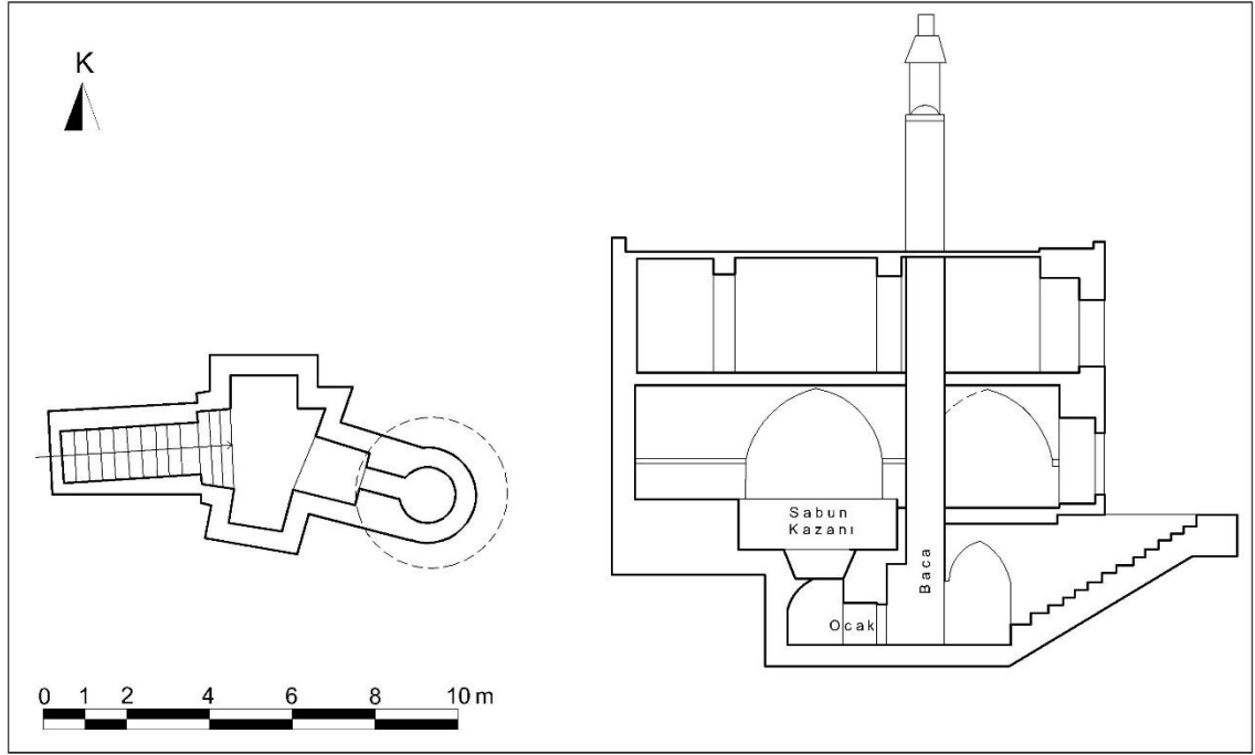
Çizim 115: Kilis Kalaycılar Sabunhanesi Ocaklık Plâni ve Kesiti (Gaziantep KVKBKM Arşivinden İşlenerek)
