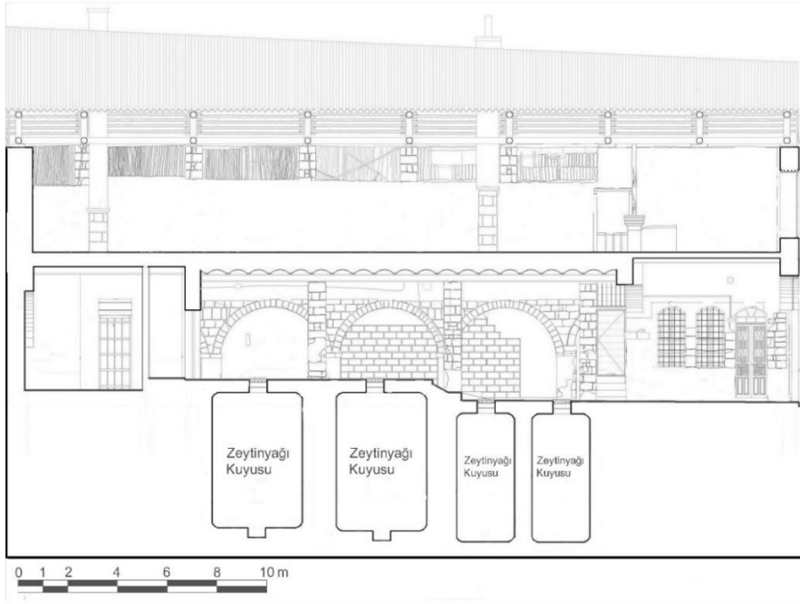
Çizim 107: Kilis Muharrem Bey Sabunhanesi Zeytinyağı Kuyuları Kesiti (F.R.Polat, YLT'den İşlenerek)
