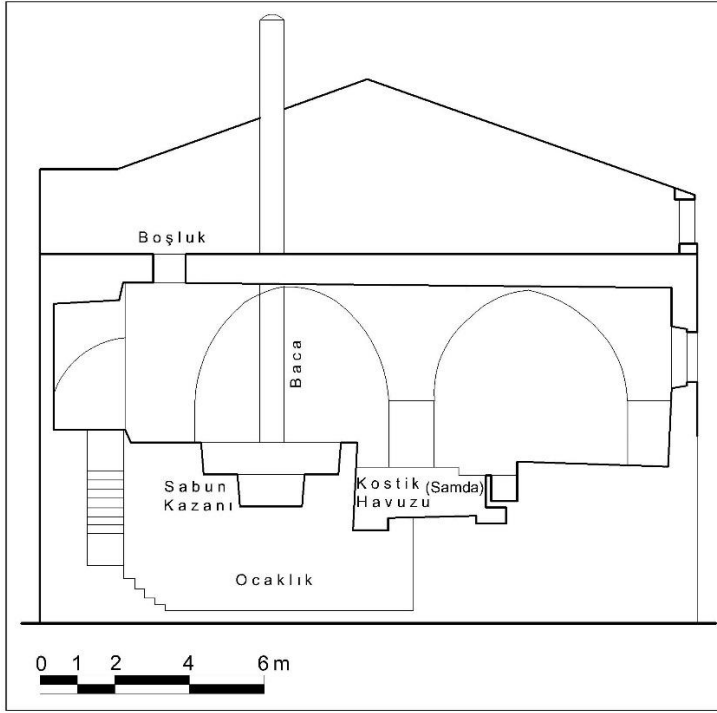
Çizim 77: Antakya Aşelcioğlu Sabunhanesi Ocaklık, Kazan, Kostik Havuzu ve Baca Kesiti (Hatay KVKBKM Arşivinden İşlenerek)
