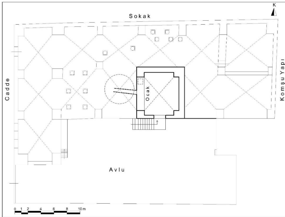
Çizim 86: Antakya Selahattin Ökten Sabunhanesi Ocaklık Plânı (M. Çiftiyürek)
