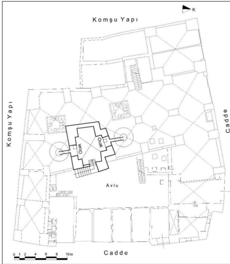
Çizim 89: Antakya Kuseyri Sabunhanesi Ocaklık Plânı (Mim. Deniz Emir)
