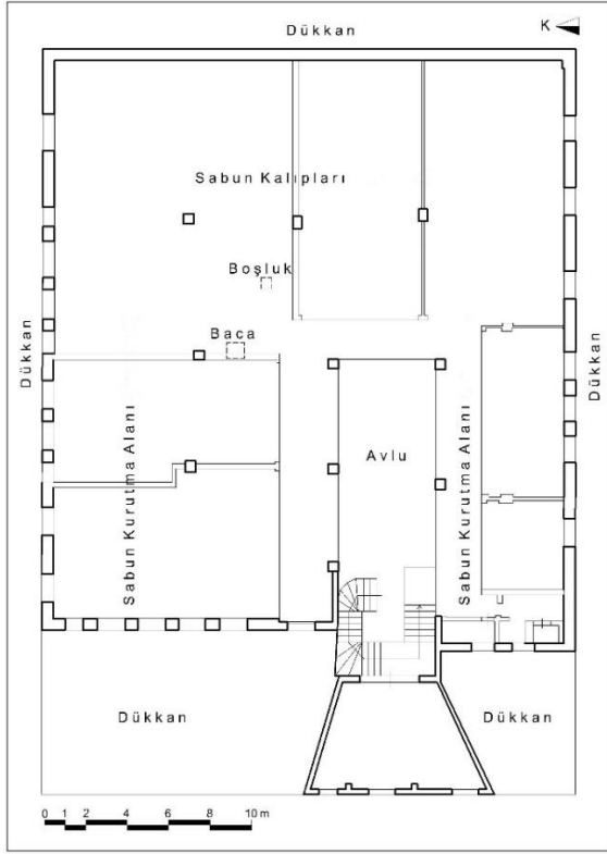
Çizim 93: Antakya Müftüoğlu Sabunhanesi Birinci Kat Plânı (M.Çiftiyürek)
