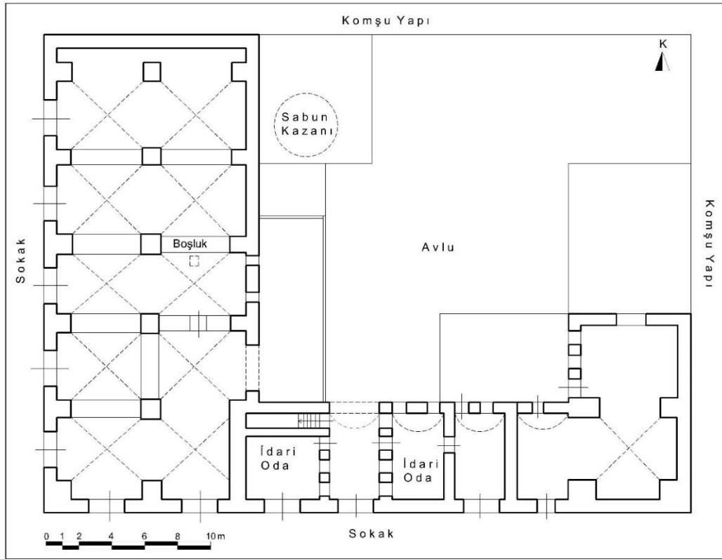
Çizim 109: Nizip Fındıklar Sabunhanesi Zemin Kat Plânı (H. Eker, YLT'den İşlenerek)
