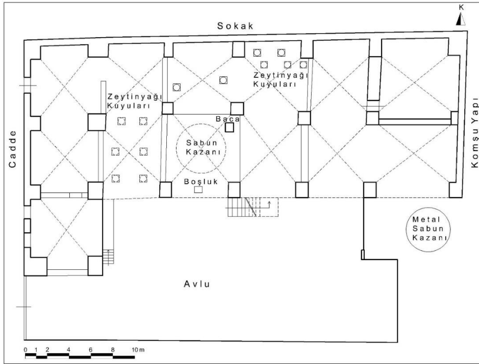
Çizim 85: Antakya Selahattin Ökten Sabunhanesi Zemin Kat Plânı (M. Çiftiyürek)
