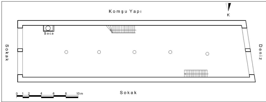
Çizim 26: Ayvalık Erman Sabunhanesi Asma Kat Plânı (Ayvalık Belediyesi Arşivinden İşlenerek)
