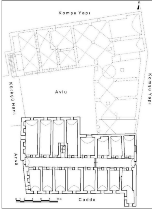
Çizim 95: Gaziantep Kürkçü Sabunhanesi Güney Bölüm Birinci Kat Plânı (Gaziantep KVKBKM Arşivinden İşlenerek)
