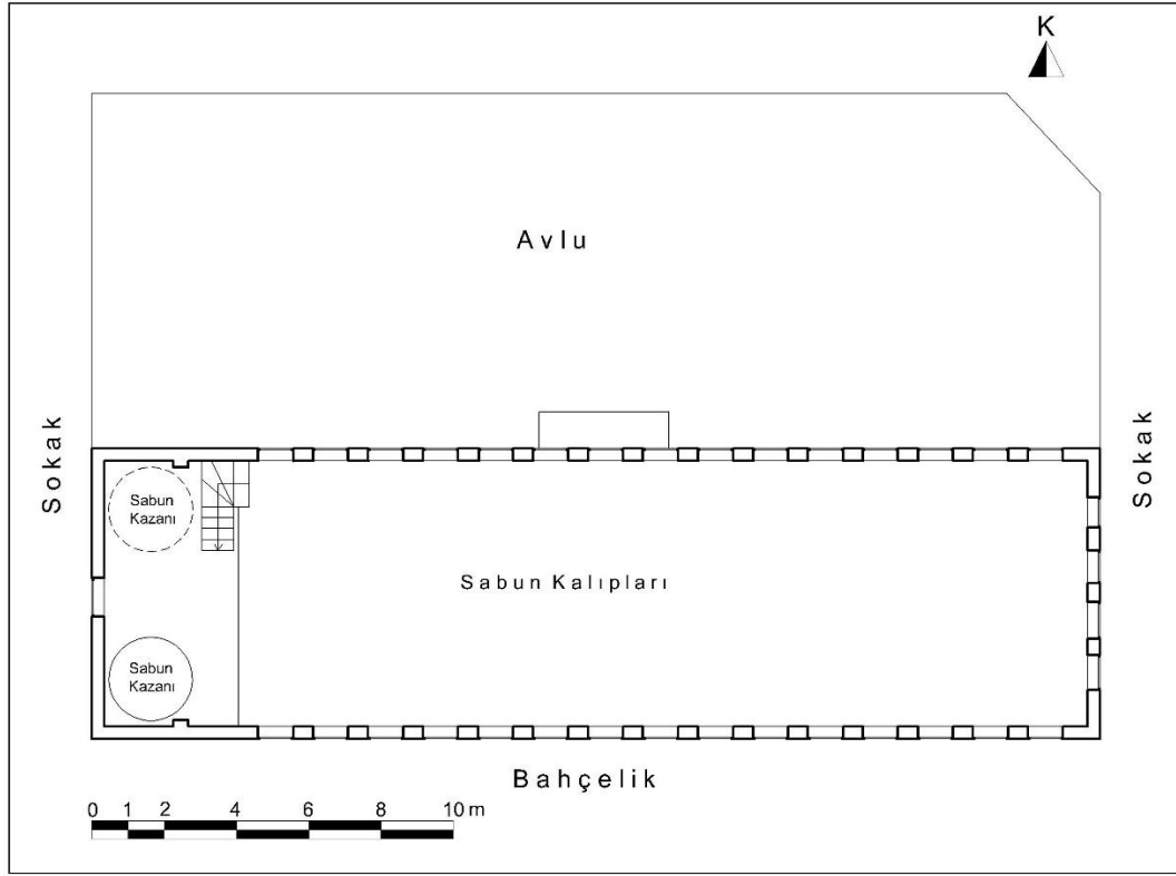
Çizim 65: Ayvacık Küçükkuyu Burnaz Sabunhanesi Birinci Kat Plânı (M. Çiftyürek)
