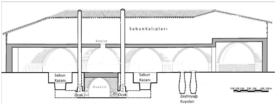
Çizim 90: Antakya Kuseyri Sabunhanesi Kazan, Ocak, Zeytinyağı Kuyusu ve Baca Kesiti (D. Camuz, YLT'den İşlenerek)
