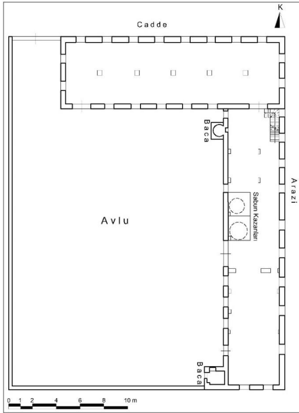
Çizim 69: Urla Sabunhanesi Zemin Kat Plânı (M. Çiftyürek)
