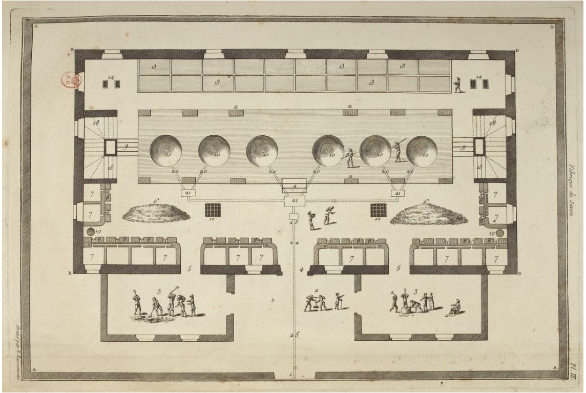
Çizim 1: Marsilya'da Bir Sabunhane Plânı (M. D. Monceau, age, P. III)
