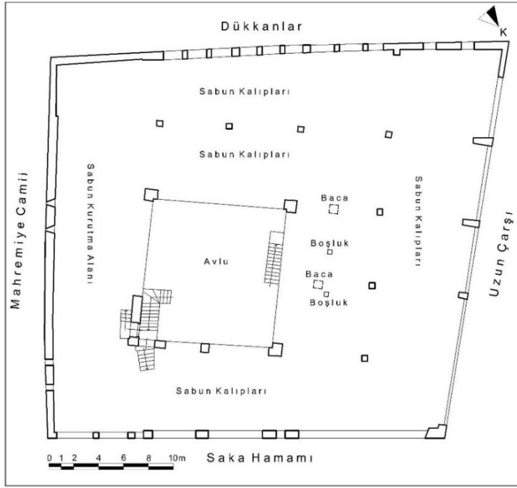
Çizim 75: Antakya Haytoğlu Sabunhanesi Birinci Kat Plânı (Hatay KVKBKM Arşivinden İşlenerek)
