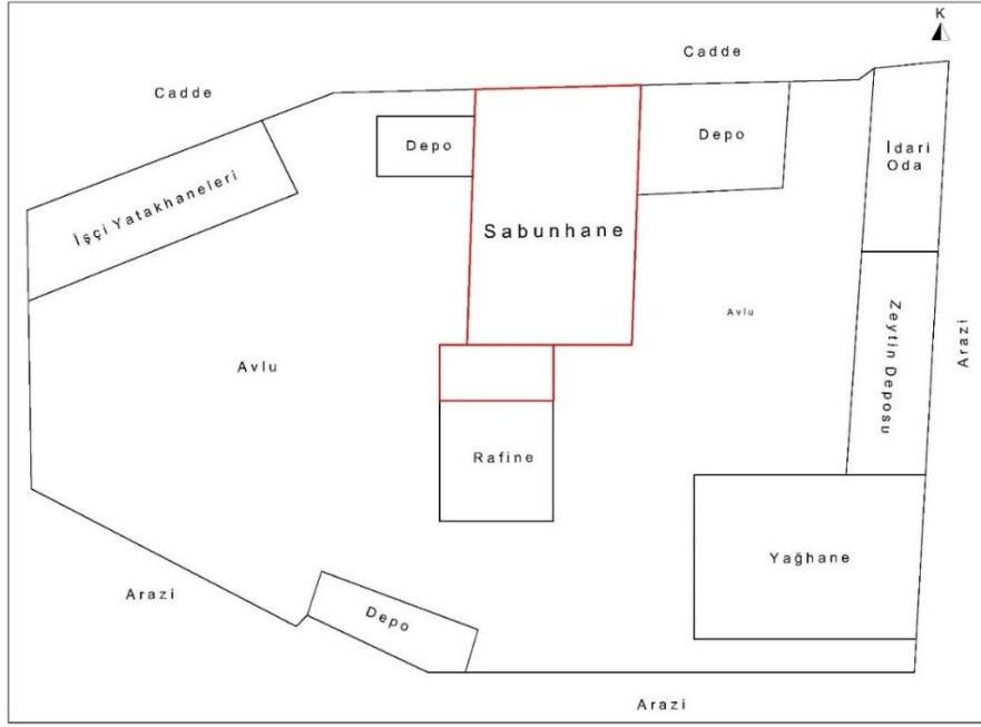
Çizim 61: Burhaniye Pelitköy Halil İbrahim Selçuk Sabunhanesi Vaziyet Plânındaki Yeri (M. Çiftyürek)
