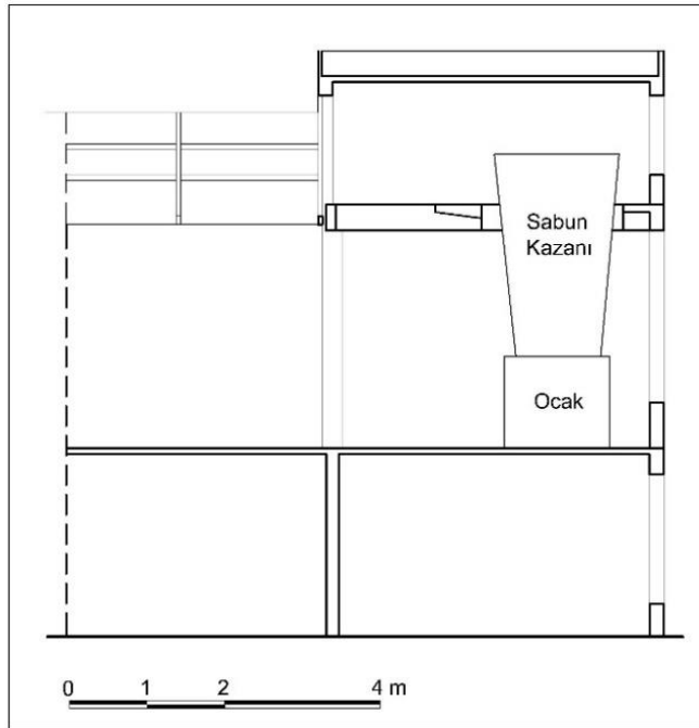
Çizim 36: Ayvalık Fazıl Doğan Sabunhanesi Ocak ve Sabun Kazanından Kesit (Ayvalık Belediyesi İşlenerek)
