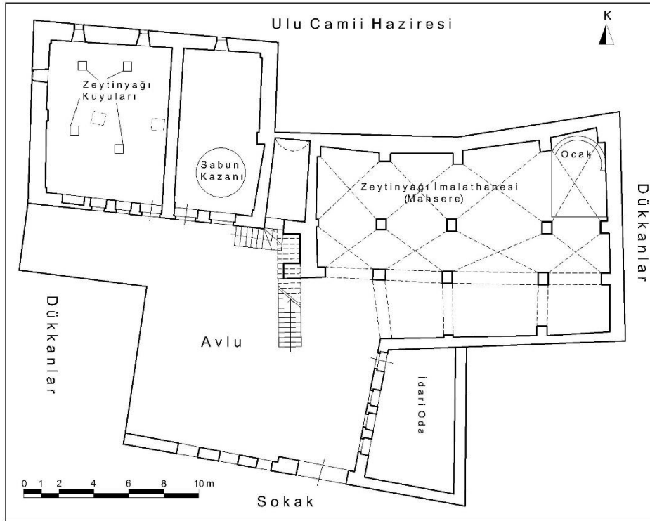
Çizim 118: Kahramanmaraş Cumhuriyet Hanı Sabunhanesi Zemin Kat Plânı (Gaziantep KVKBKM Arşivinden İşlenerek)
