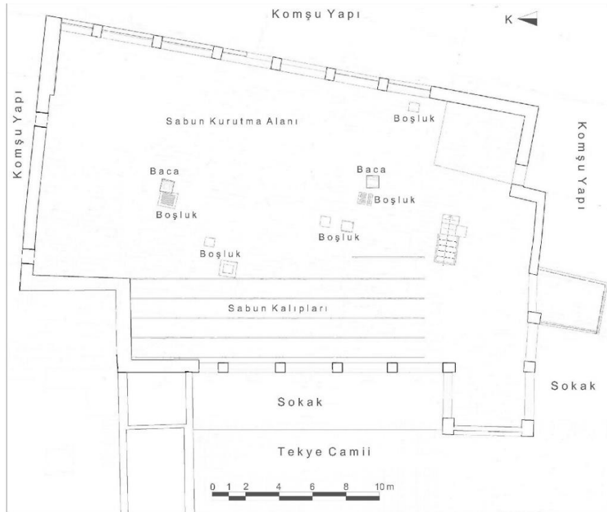
Çizim 108: Kilis Muharrem Bey Sabunhanesi Birinci Kat Plânı (F.R.Polat, YLT'den İşlenerek)
