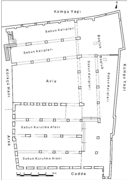
Çizim 96: Gaziantep Kürkçü Sabunhanesi Kuzey ve Doğu Bölümün Birinci Katı ile Güney Bölümün İkinci Kat Plânı (Gaziantep KVKBKM Arşivinden İşlenerek)
