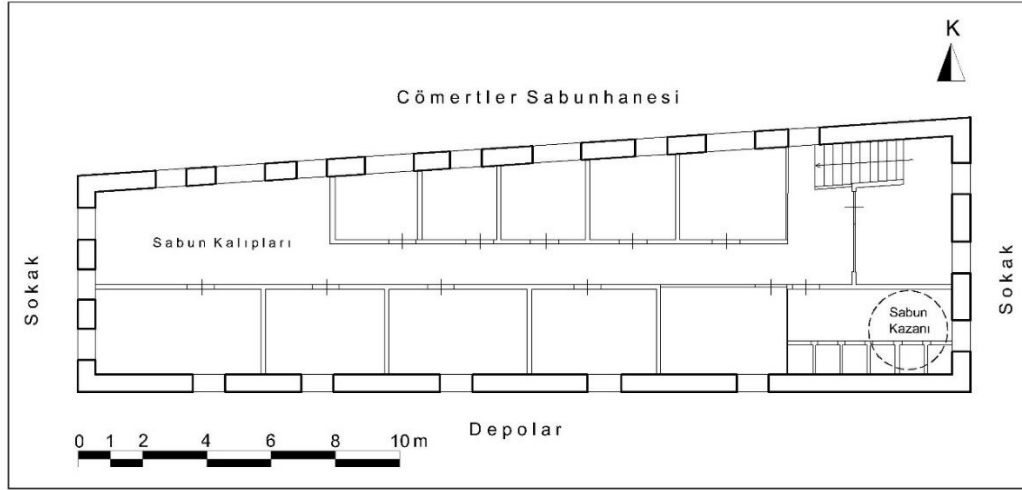
Çizim 28: Ayvalık Sabuncugil Sabunhanesi Birinci Kat Plânı ( http://cyddayvalikiktisadiisletme.com/ayvalik-cydd-konukevi/ İşlenerek)
