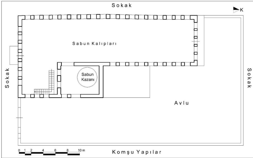
Çizim 57: Burhaniye Hüsnü Pazarbaşı Sabunhanesi Restorasyon Öncesi Birinci Kat Plânı (Ayvalık Belediyesi Arşivinden İşlenerek)
