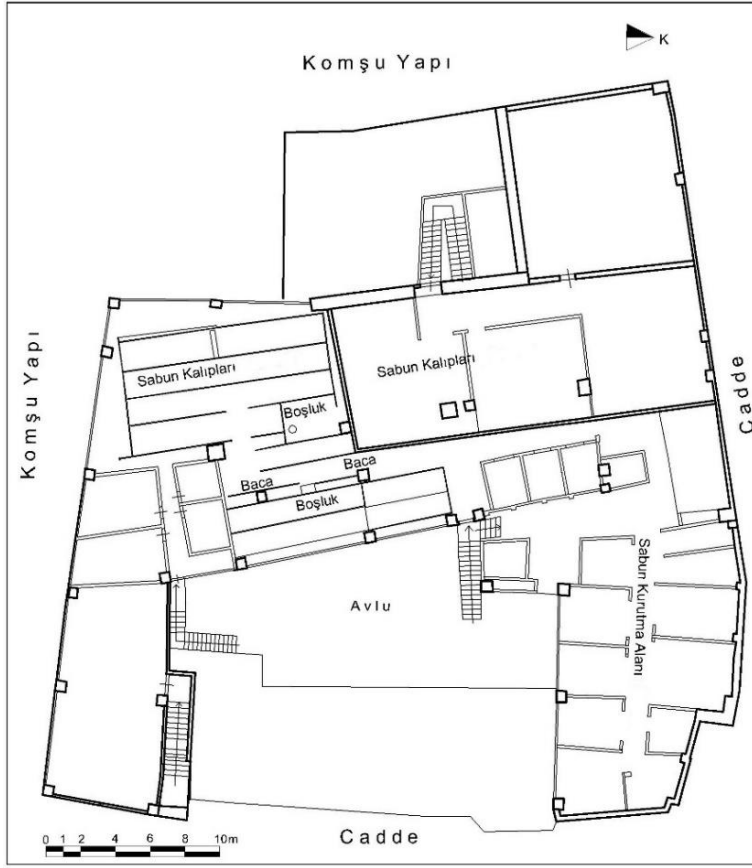
Çizim 91: Antakya Kuseyri Sabunhanesi Birinci Kat Plânı (Mim. Deniz Emir)
