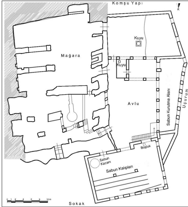
Çizim 103: Birecik Mıstıkoğlu Sabunhanesi Birinci Kat Plânı (M. Çiftiyürek)
