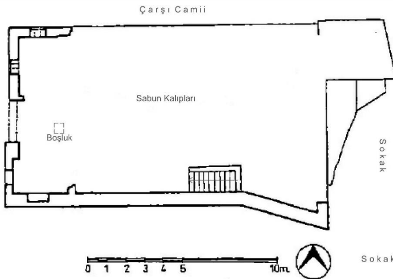
Çizim 48 BİRECİK SABUNHANE, ÜST KAT RÖLÖVE PLANI Rölöve : M. Görür-A. Durukan (Mayıs 1998) Çizen : M. Görür (Haziran 1998)
