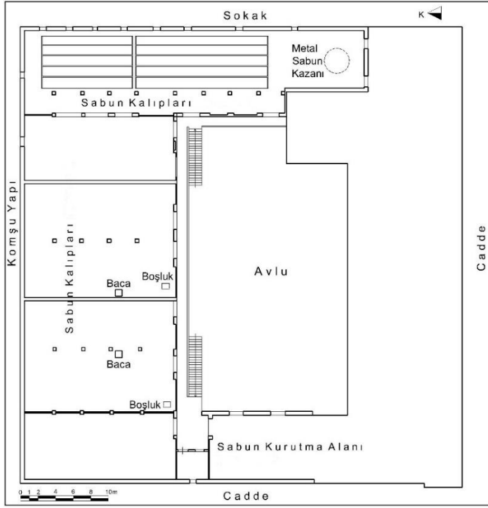
Çizim 83: Antakya Şehoğlu Sabunhanesi Birinci Kat Plânı (Hatay KVKBKM Arşivinden İşlenerek)
