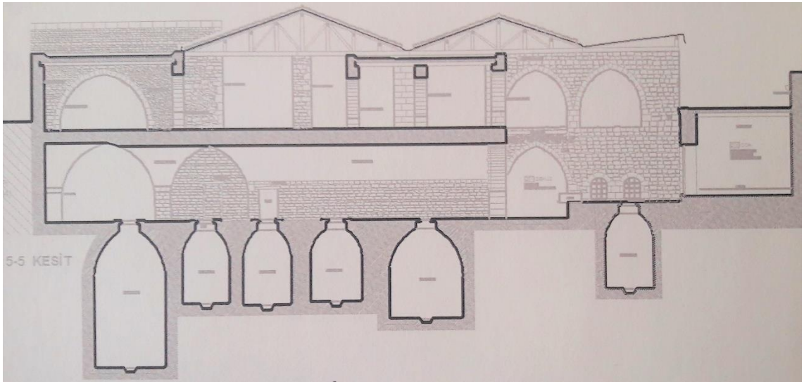
Çizim 116: Kilis Kalaycılar Sabunhanesi Zeytinyağı Kuyuları Kesiti (Gaziantep KVKBKM Arşivi)
