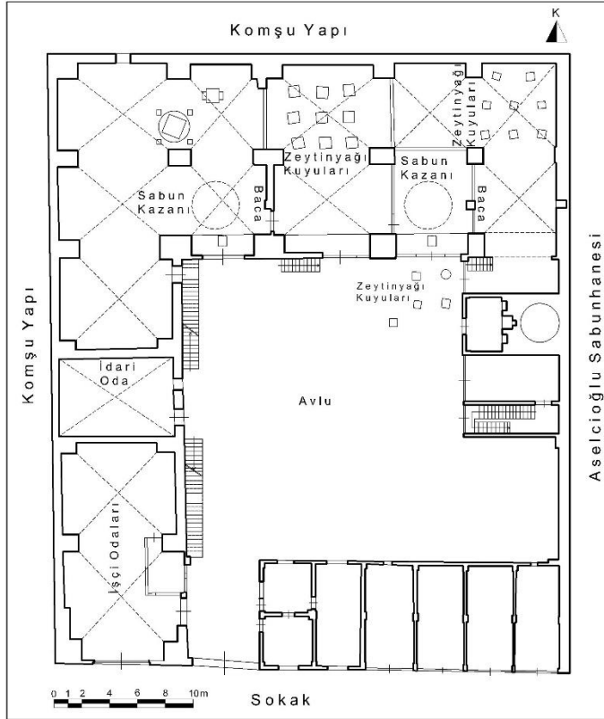
Çizim 78: Antakya Hasan Ökten Sabunhanesi Zemin Kat Plânı (Hatay KVKBKM Arşivinden İşlenerek)
