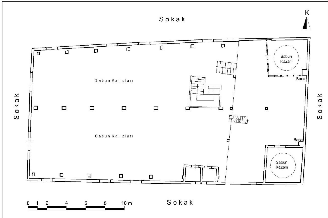
Çizim 21: Ayvalık Hüsnü Rıfki Kazaz Sabunhanesi Restorasyon Öncesi Birinci Kat Plânı (Ayvalık Belediyesi Arşivinden İşlenerek)
