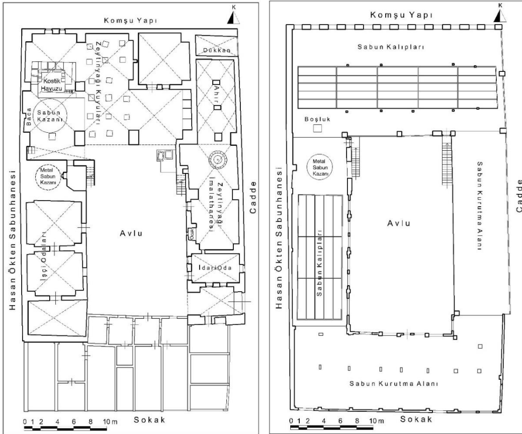
Çizim 76: Antakya Aselcioğlu Sabunhanesi Zemin ve Birinci Kat Plânı (Hatay KVKBKM Arşivinden İşlenerek)
