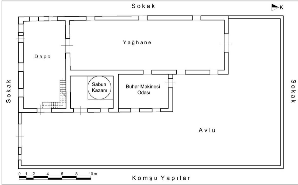
Çizim 55: Burhaniye Hüsnü Pazarbaşı Sabunhanesi Restorasyon Öncesi Zemin Kat Plânı (Ayvalık Belediyesi Arşivinden İşlenerek)
