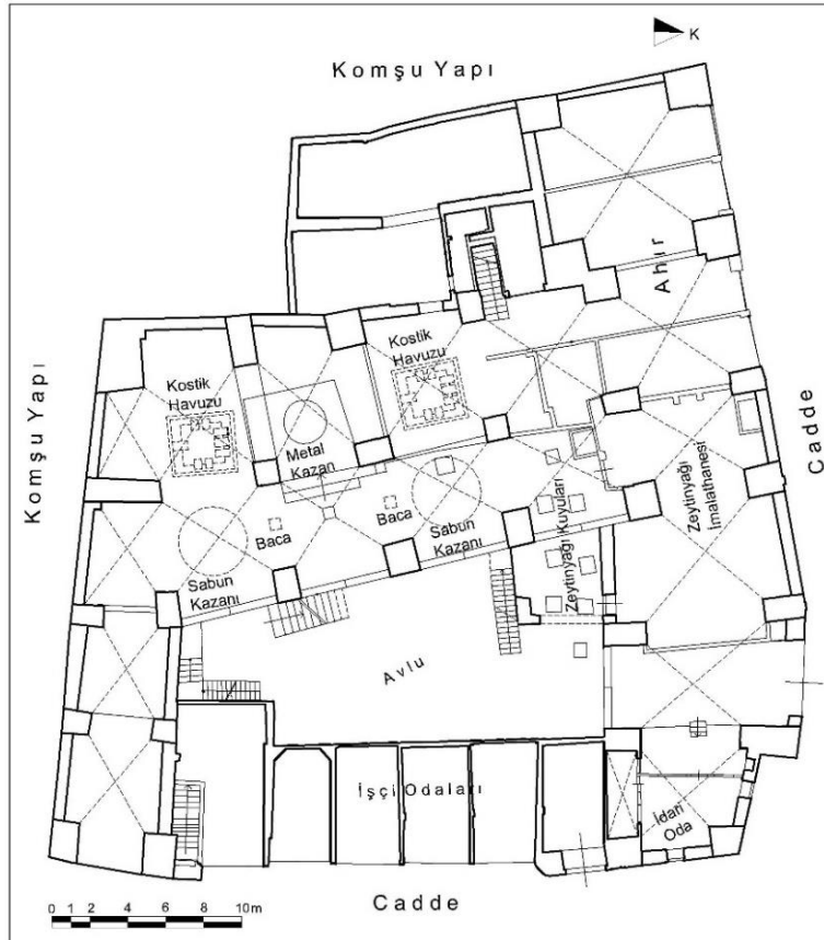
Çizim 88: Antakya Kuseyri Sabunhanesi Zemin Kat Planı (Mim. Deniz Emir)
