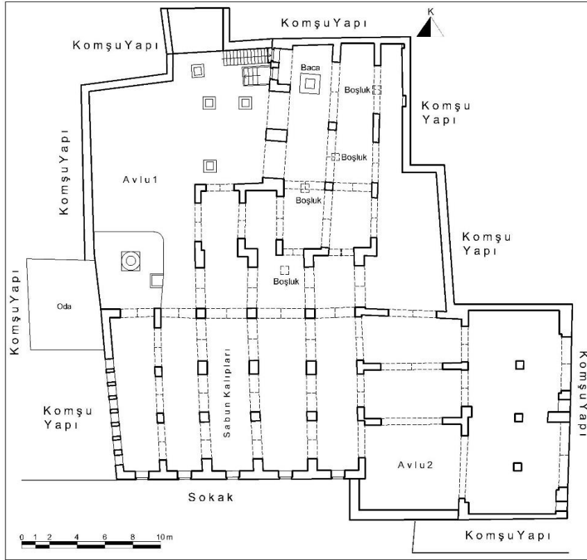
Çizim 117: Kilis Kalaycılar Sabunhanesi Birinci Kat Plânı (Gaziantep KVKBKM Arşivinden İşlenerek)
