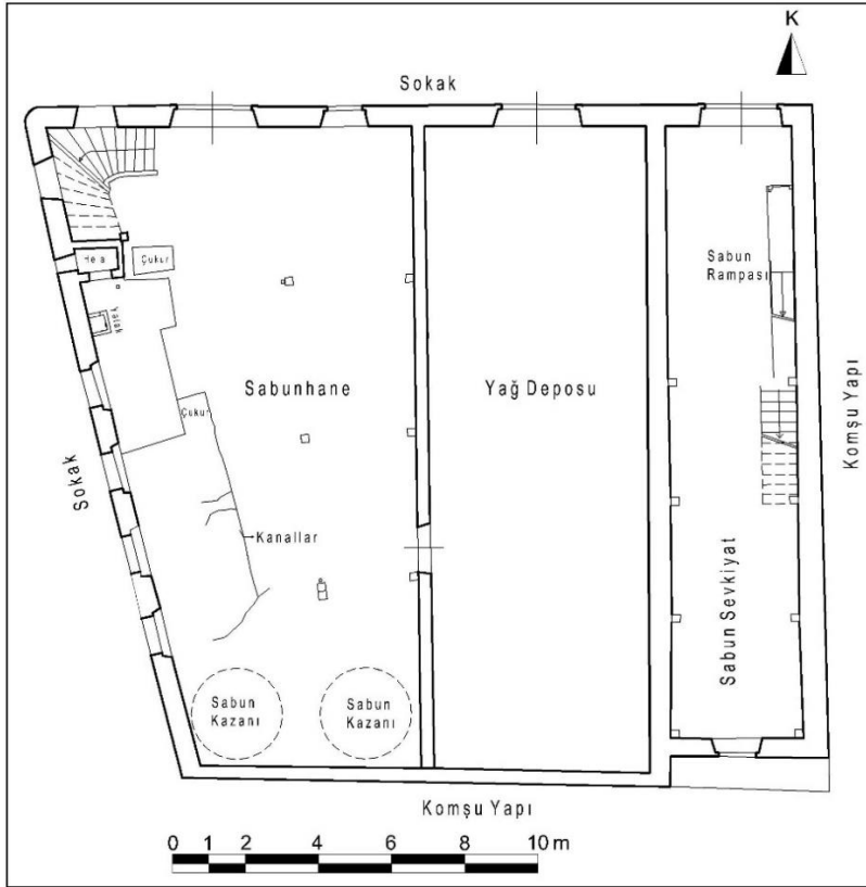
Çizim 66: Konak Hamdi Dalan Sabunhanesi Zemin Kat Plânı (Konak Belediyesi Arşivinden İşlenerek)
