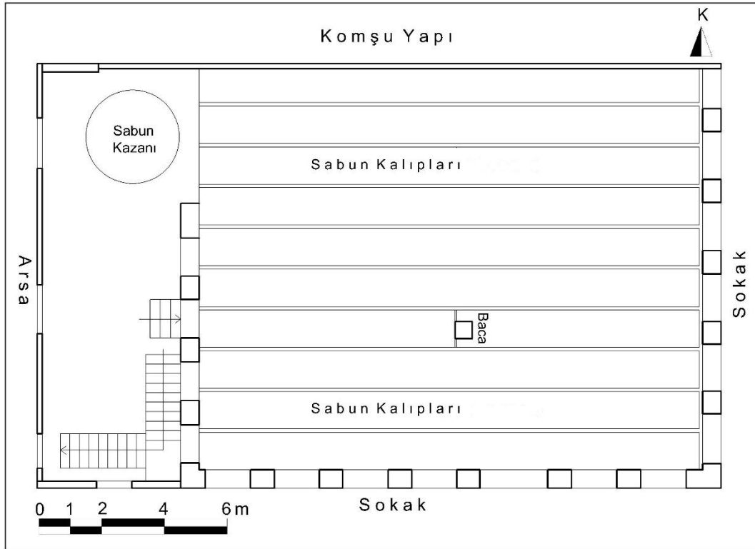
Çizim 112: Nizip Okanlar Sabunhanesi Birinci Kat Plânı (M. Çiftyürek)
