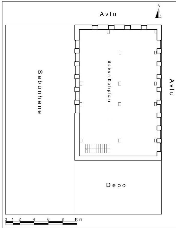
Çizim 68: Konak Sabunhanesi Birinci Kat Plânı (M. Çiftyürek)
