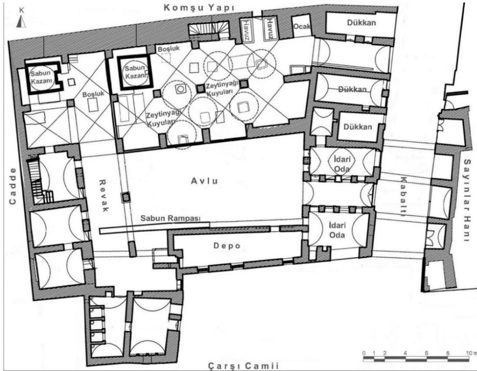
Çizim 104: Nizip Sayınlar Sabunhanesi Zemin Kat Plânı (Ö. Bozgeyik, YLT'den İşlenerek)
