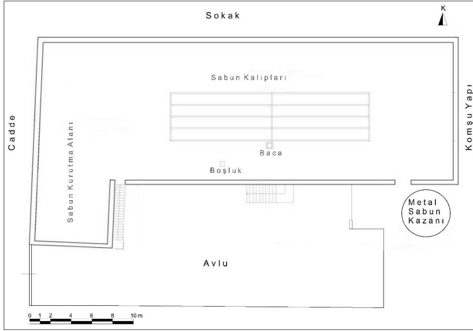
Çizim 87: Antakya Selahattin Ökten Sabunhanesi Birinci Kat Planı (F.R. Polat, YLT'den İşlenerek)
