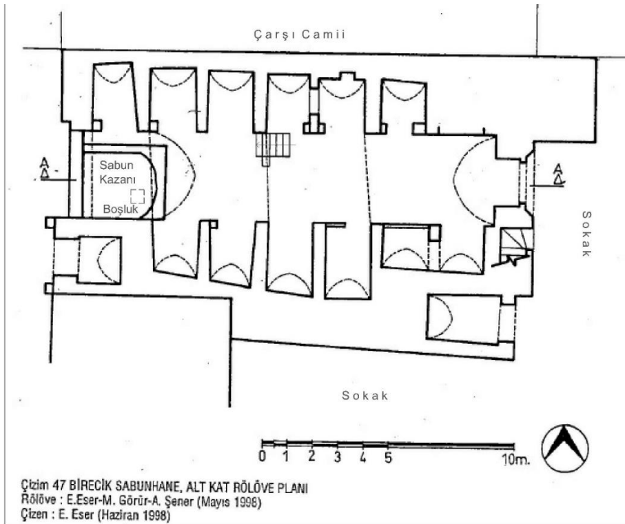
Çizim 126: Birecik Akçakanat Sabunhanesi Zemin Kat Plânı (A. Durukan vd., age, s. 127)
