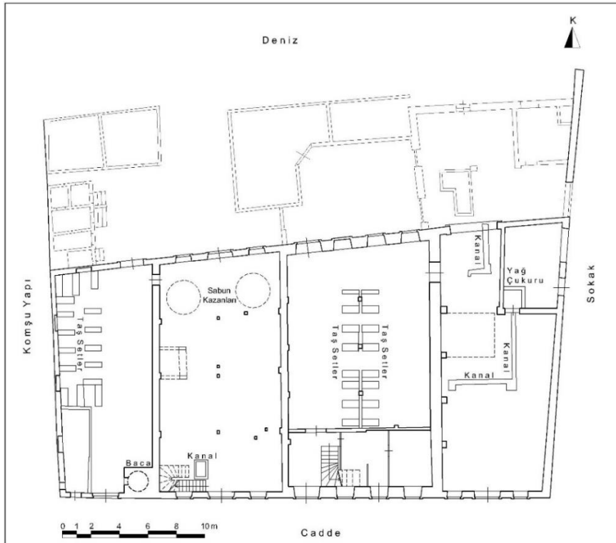
Çizim 122: Ayvalık Sezai Ömer Madra Sabunhanesi Zemin Kat Plânı (Bursa KVKBKM Arşivinden İşlenerek)
