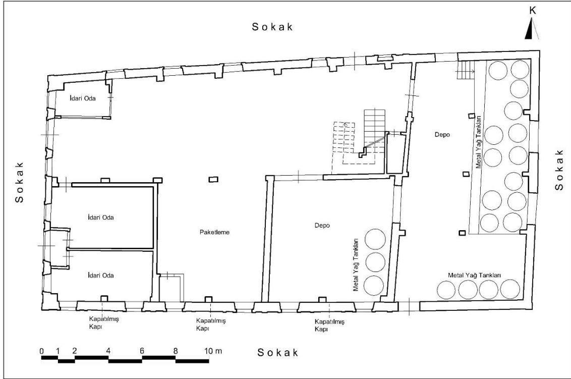
Çizim 20: Ayvalık Hüsnü Rıfki Kazaz Sabunhanesi Restorasyon Öncesi Zemin Kat Plânı (Ayvalık Belediyesi Arşivinden İşlenerek)
