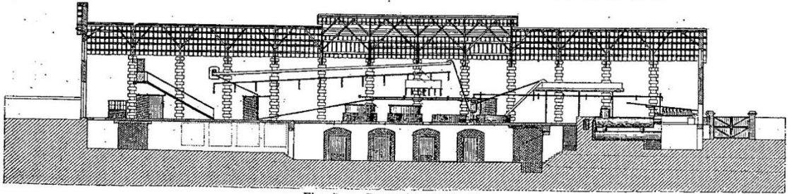
Çizim 10: Marsilya Baron Sabun Fabrikası Enine ve Boyuna Kesiti (E. Moride, age, 1895, s. 79)
