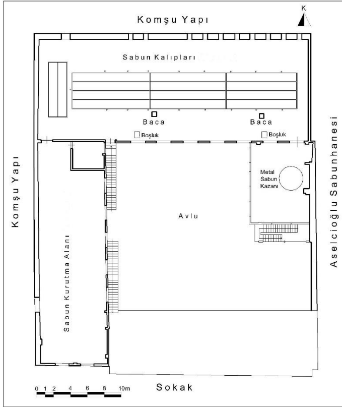
Çizim 81: Antakya Hasan Ökten Sabunhanesi Birinci Kat Plânı (Hatay KVKBKM Arşivinden İşlenerek)
