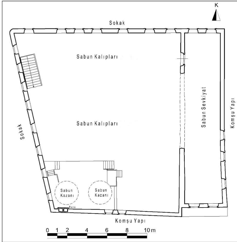
Çizim 67: Konak Hamdi Dalan Sabunhanesi Birinci Kat Plânı (Konak Belediyesi Arşivinden İşlenerek)
