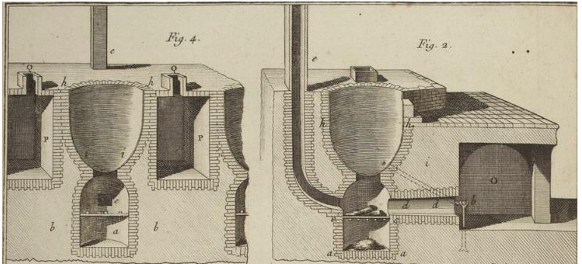
Çizim 2: Ateş Sistemi ile Çalışan Sabun Kazanının Boyuna ve Enine Kesiti (M. D. Monceau, age, Fig. 2-4)
