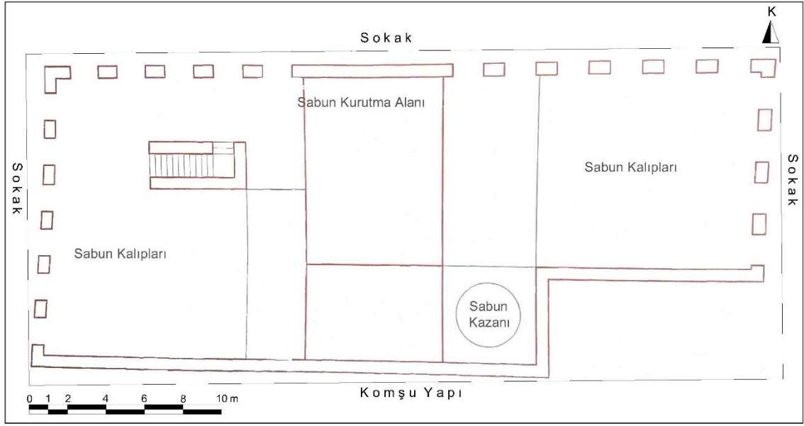
Çizim 113: Nizip Özkaya Sabunhanesi Krokisi (Gaziantep KVKBKM Arşivinden İşlenerek)
