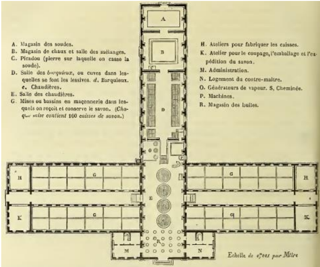
Çizim 6: Marsilya'da Bir Sabun Fabrikası Plânı (L. Figuiet, age, s. 416)
