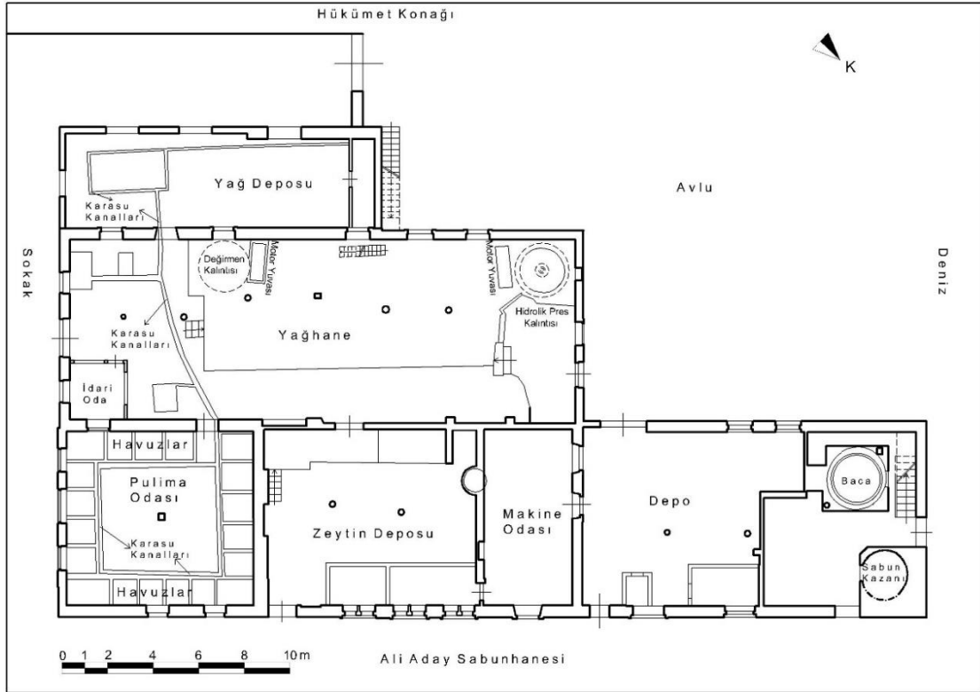
Çizim 43: Ayvalık Ertemler Sabunhanesi Zemin Kat Plânı (Ayvalık Belediyesi Arşivinden İşlenerek)
