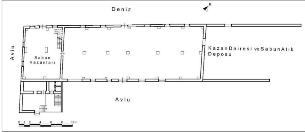
Çizim 33: Ayvalık Fazıl Doğan Sabunhanesi Zemin Kat Plânı (Bursa KVKBKM Arşivinden İşlenerek)
