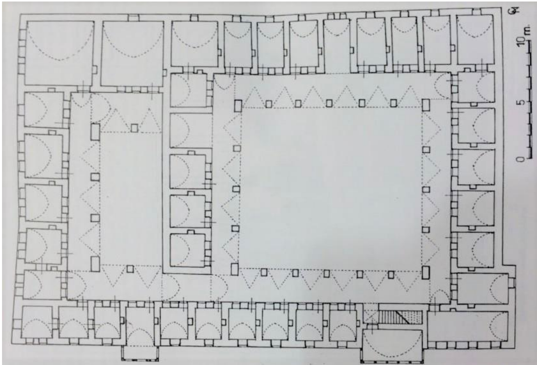
Çizim 100: Gaziantep Elbeyli Sabunhanesi Birinci Kat Plânı (N. Çam, age, s. 450)
