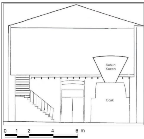
Çizim 38: Ayvalık Fevzi Paşa Mahallesi'ndeki Sabunhanenin Ocak ve Kazan Kesiti (Bursa KVKBKM Arşivinden İşlenerek)
