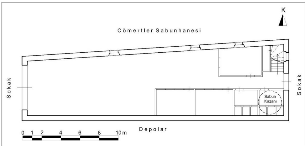
Çizim 27: Ayvalık Sabuncuğil Sabunhanesi Zemin Kat Plânı ( http://cyddayvalikiktisadiisletme.com/ayvalik-cydd-konukevi/ İşlenerek)
