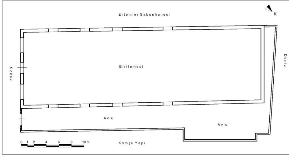
Çizim 22: Ayvalık Ali Aday Sabunhanesi Zemin Kat Plânı (M. Çiftiyürek)
