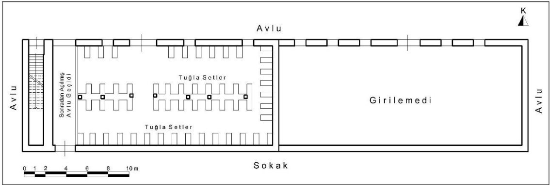
Çizim 46: Havran Eminzade Sabunhanesi Zemin Kat Plânı (M. Çiftyürek)
