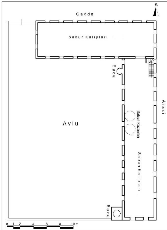
Çizim 70: Urla Sabunhanesi Birinci Kat Plânı (M. Çiftyürek)
