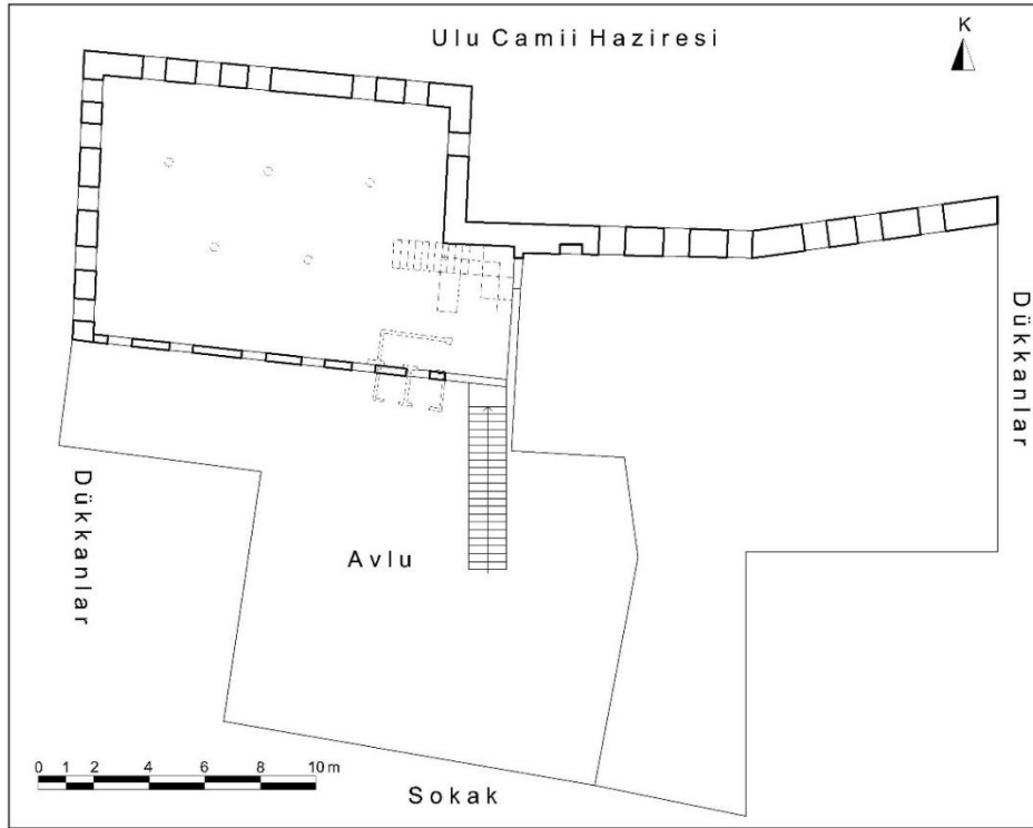
Çizim 119: Kahramanmaraş Cumhuriyet Hanı Sabunhanesi Birinci Kat Plânı (Gaziantep KVKBKM Arşivinden İşlenerek)
