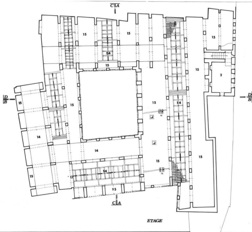
Çizim 17: Halep Sabuni Sabunhanesi Birinci Kat Plânı (T. Grandin, agm, P. XIIB)
