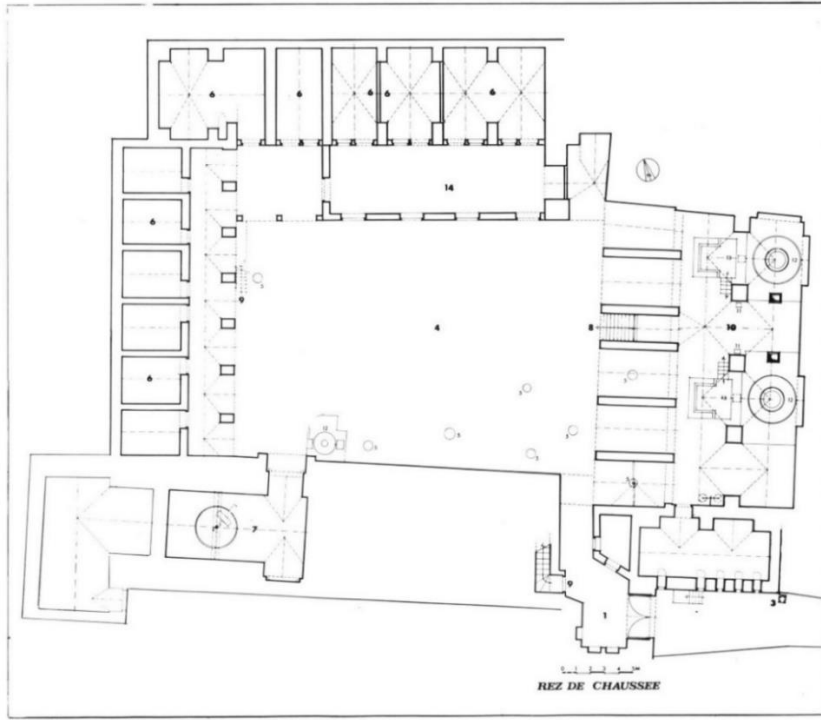
Çizim 14: Halep Zenabli Mar'Aslı Sabunhanesi Zemin Kat Plânı (T. Grandin, agm, P. XIA)
