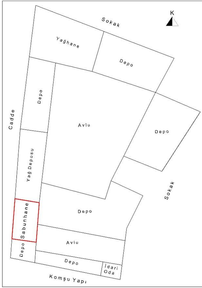
Çizim 52: Edremit Ali Rıza Karagözoğlu Sabunhanesi Vaziyet Plânındaki Yeri (M. Çiftyürek)
