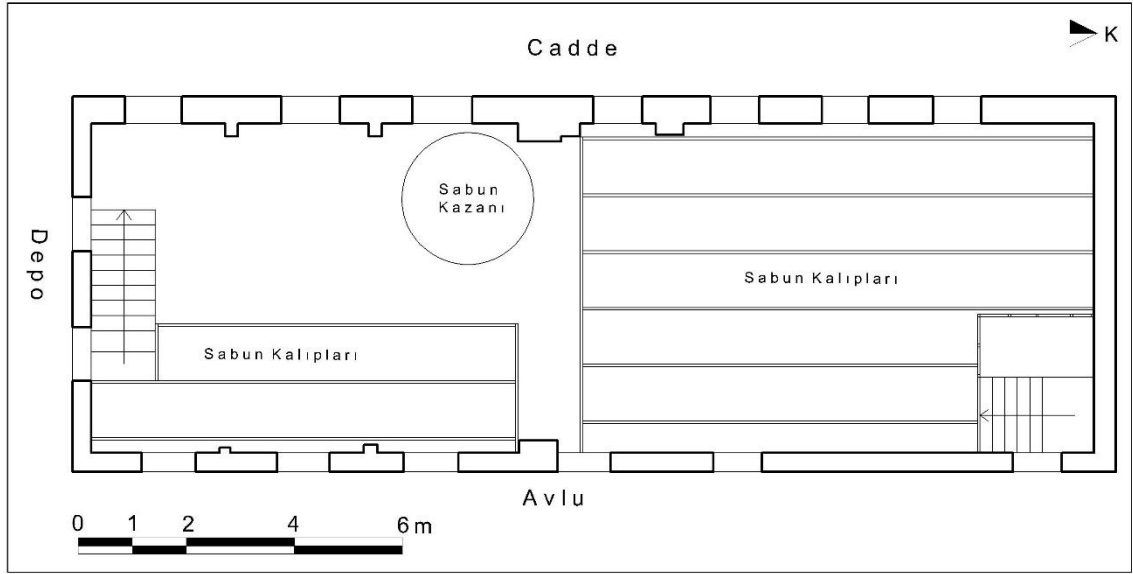
Çizim 54: Edremit Ali Rıza Karagözoğlu Sabunhanesi Birinci Kat Plânı (M. Çiftyürek)
