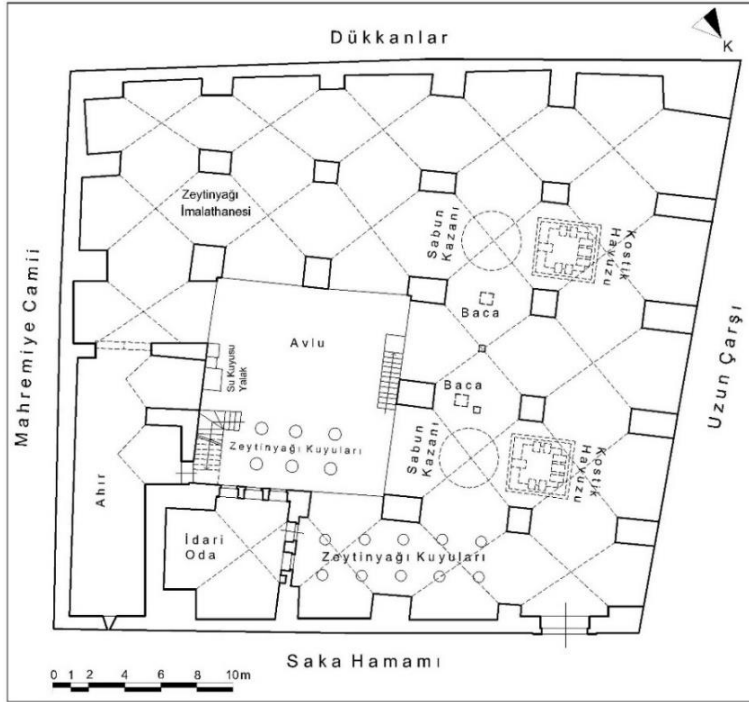
Çizim 71: Antakya Haytoğlu Sabunhanesi Zemin Kat Plânı (Hatay KVKBKM Arşivinden İşlenerek)
