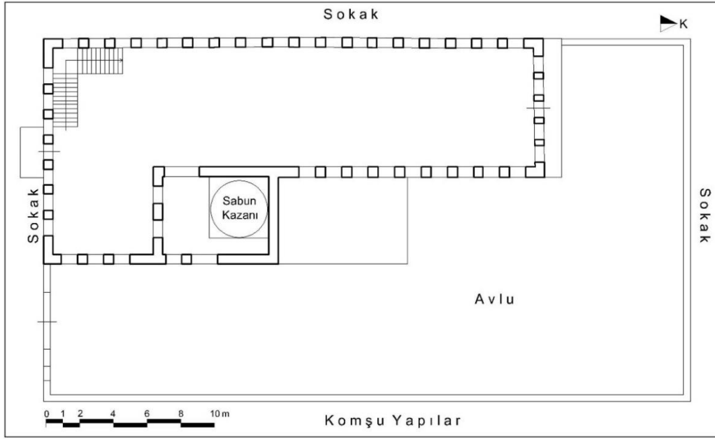
Çizim 58: Burhaniye Hüsnü Pazarbaşı Sabunhanesi Restorasyon Sonrası Birinci Kat Plânı (Ayvalık Belediyesi Arşivinden İşlenerek)
