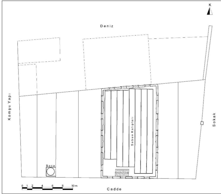
Çizim 125: Ayvalık Sezai Ömer Madra Sabunhanesi Üçüncü Kat Plânı (Bursa KVKBKM Arşivinden İşlenerek)
