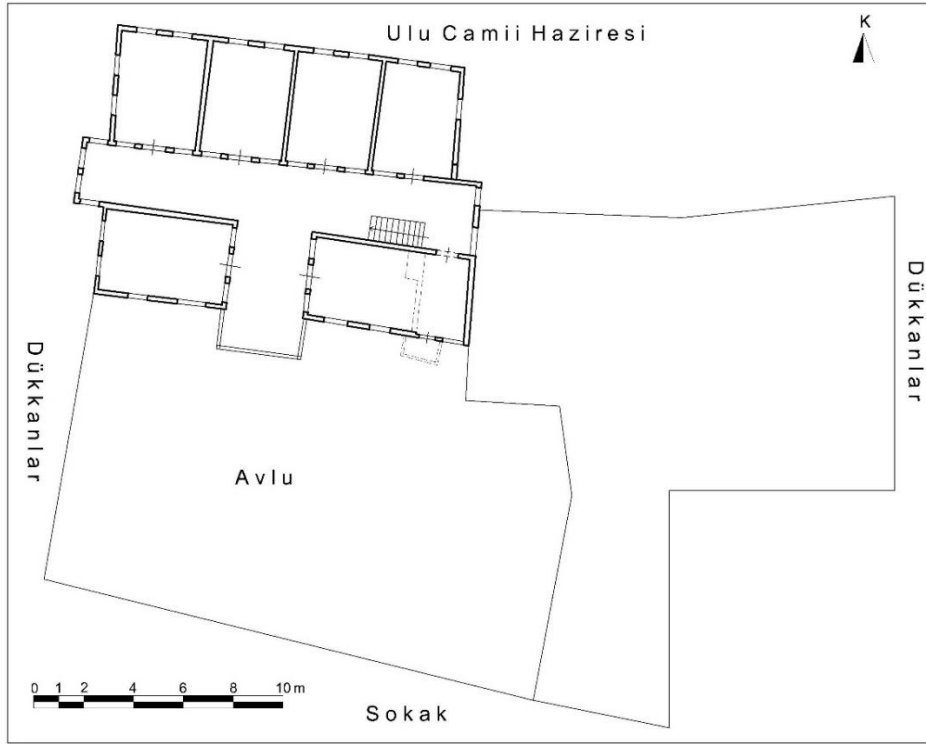
Çizim 121: Kahramanmaraş Cumhuriyet Hanı Sabunhanesi İkinci Kat Plânı (Gaziantep KVKBKM Arşivinden İşlenerek)
