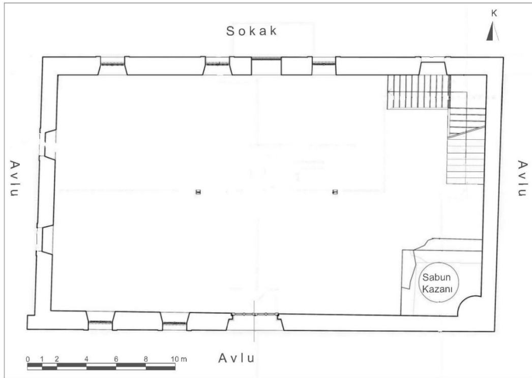
Çizim 49: Burhaniye Hüsnü Tolun Sabunhanesi Zemin Kat Plânı (D. Akın, YLT'den İşlenerek)
