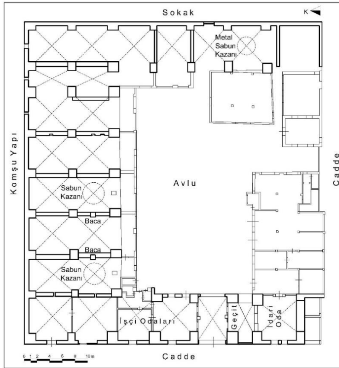
Çizim 82: Antakya Şehoğlu Sabunhanesi Zemin Kat Plânı (Hatay KVKBKM Arşivinden İşlenerek)
