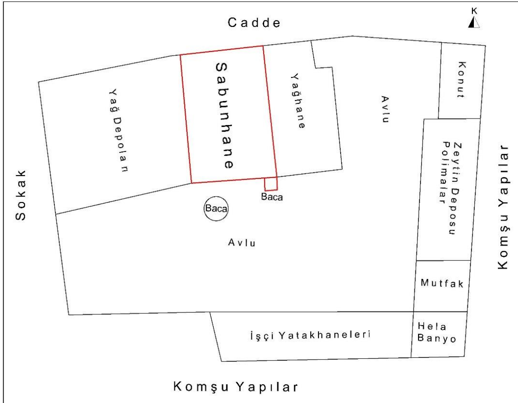
Çizim 29: Burhaniye Yağcı Sabunhanesi Vaziyet Plânındaki Yeri (M. Çiftyürek)
