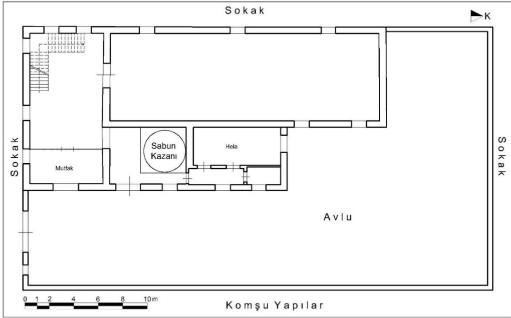
Çizim 56: Burhaniye Hüsnü Pazarbaşı Sabunhanesi Restorasyon Sonrası Zemin Kat Plânı (Ayvalık Belediyesi Arşivinden İşlenerek)
