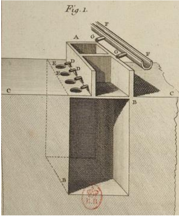
Çizim 5: Alkali Çözeltilerin Hazırlanıldığı Bugadieres veya Barquieux (M. D. Monceau, age, Fig. 1)
