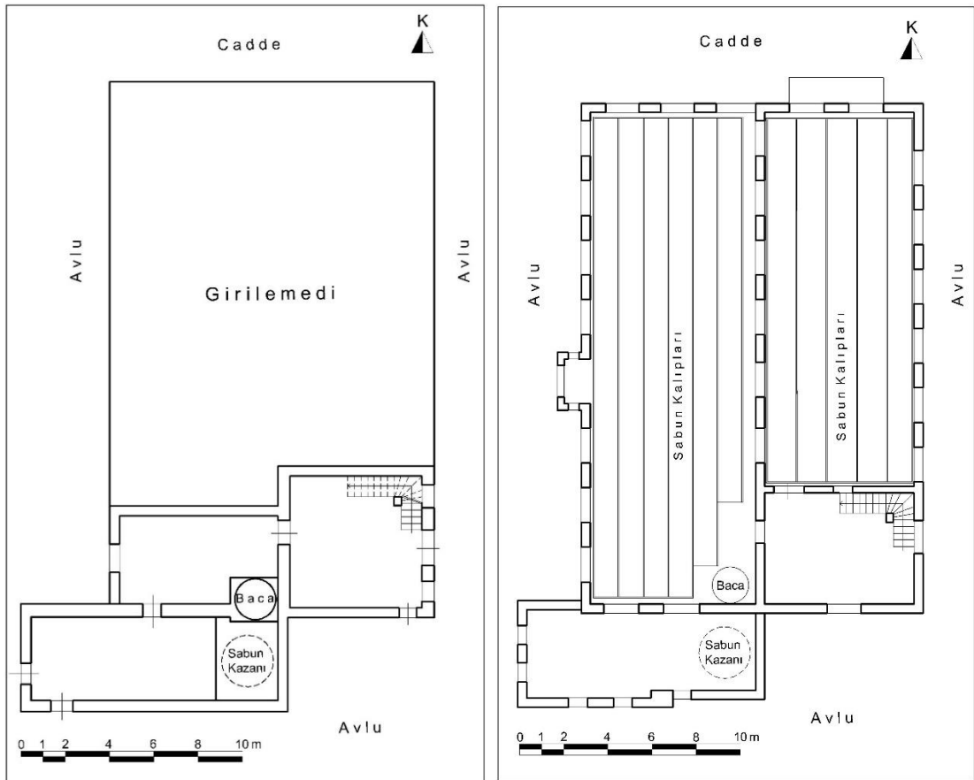
Çizim 62: Burhaniye Pelitköy Halil İbrahim Selçuk Sabunhanesi Zemin ve Birinci Kat Plânı (M. Çiftyürek)
