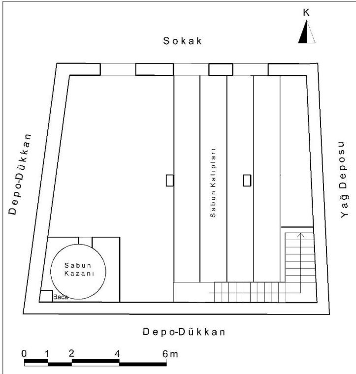
Çizim 130: Ayvalık Karşınlar Sabunhanesi Asma Kat Plânı (M. Çiftyürek)
