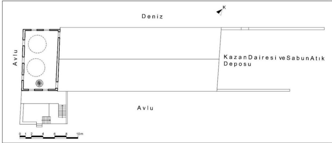
Çizim 35: Ayvalık Fazıl Doğan Sabunhanesi Asma Kat Plânı (Bursa KVKBKM Arşivinden İşlenerek)
