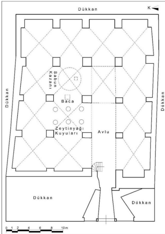
Çizim 92: Antakya Müftüoğlu Sabunhanesi Zemin Kat Plânı (M.Çiftyürek)
