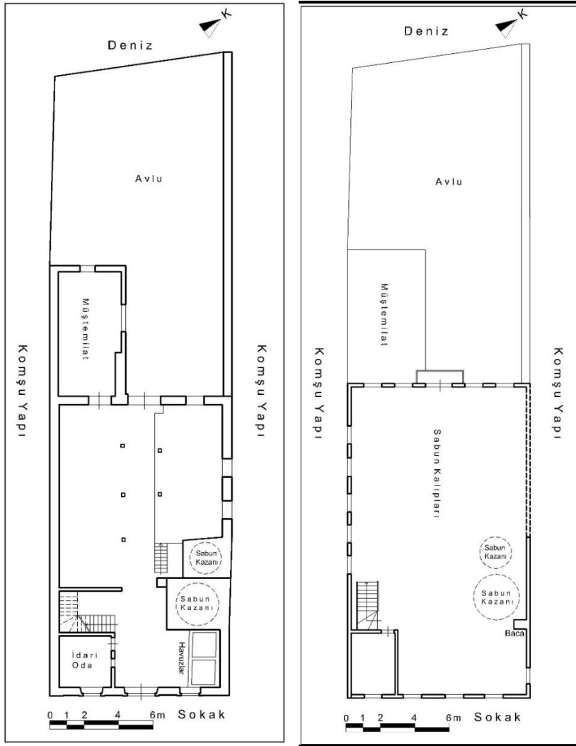
Çizim 37: Ayvalık Fevzi Paşa Mahallesi'ndeki Sabunhanenin Zemin ve Birinci Kat Plânları (Bursa KVKBKM Arşivinden İşlenerek)
