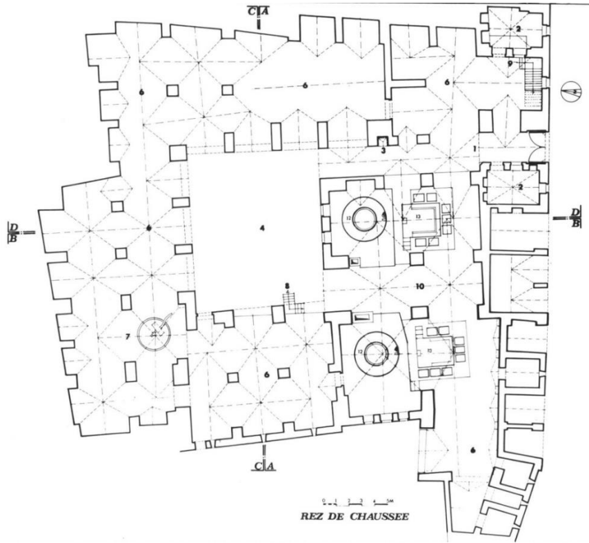
Çizim 16: Halep Sabuni Sabunhanesi Zemin Kat Plânı (T. Grandin, agm, P. XIIA)
