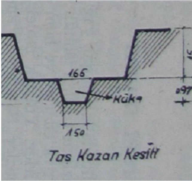
Çizim 73: Antakya Sabunhanelerindeki Taş Sabun Kazanı Kesiti (TSOTBB, age, s. 9)
