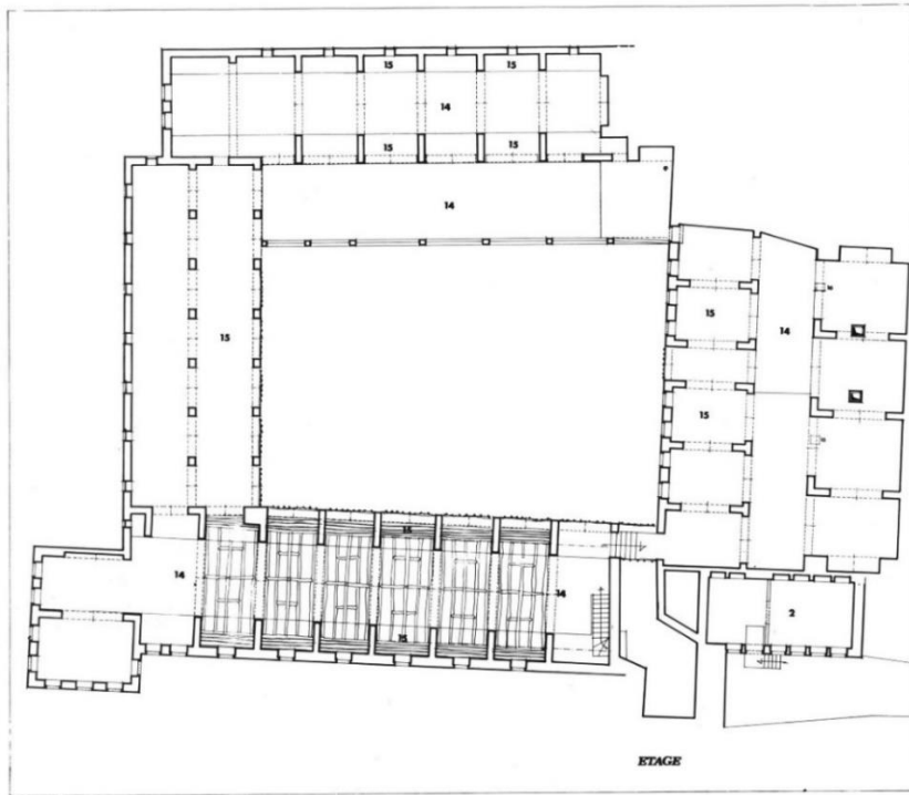
Çizim 15: Halep Zenabli Mar'Aslı Sabunhanesi Birinci Kat Plânı (T. Grandin, agm, P. XIB)
