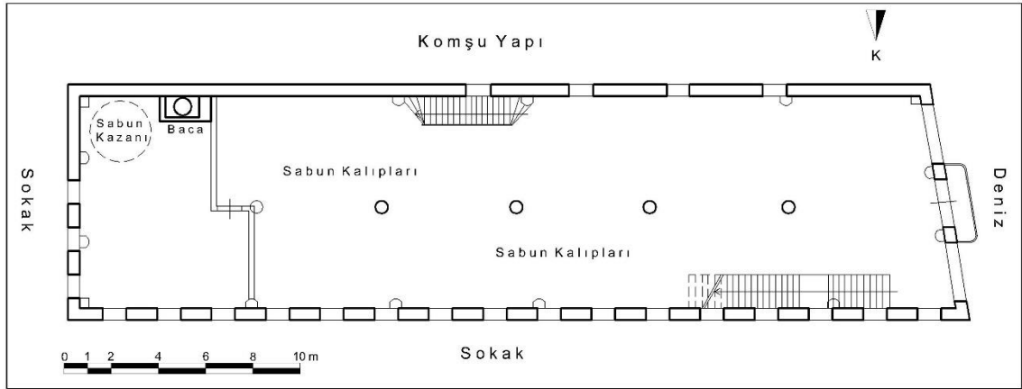
Çizim 25: Ayvalık Erman Sabunhanesi Birinci Kat Plânı (Ayvalık Belediyesi Arşivinden İşlenerek)
