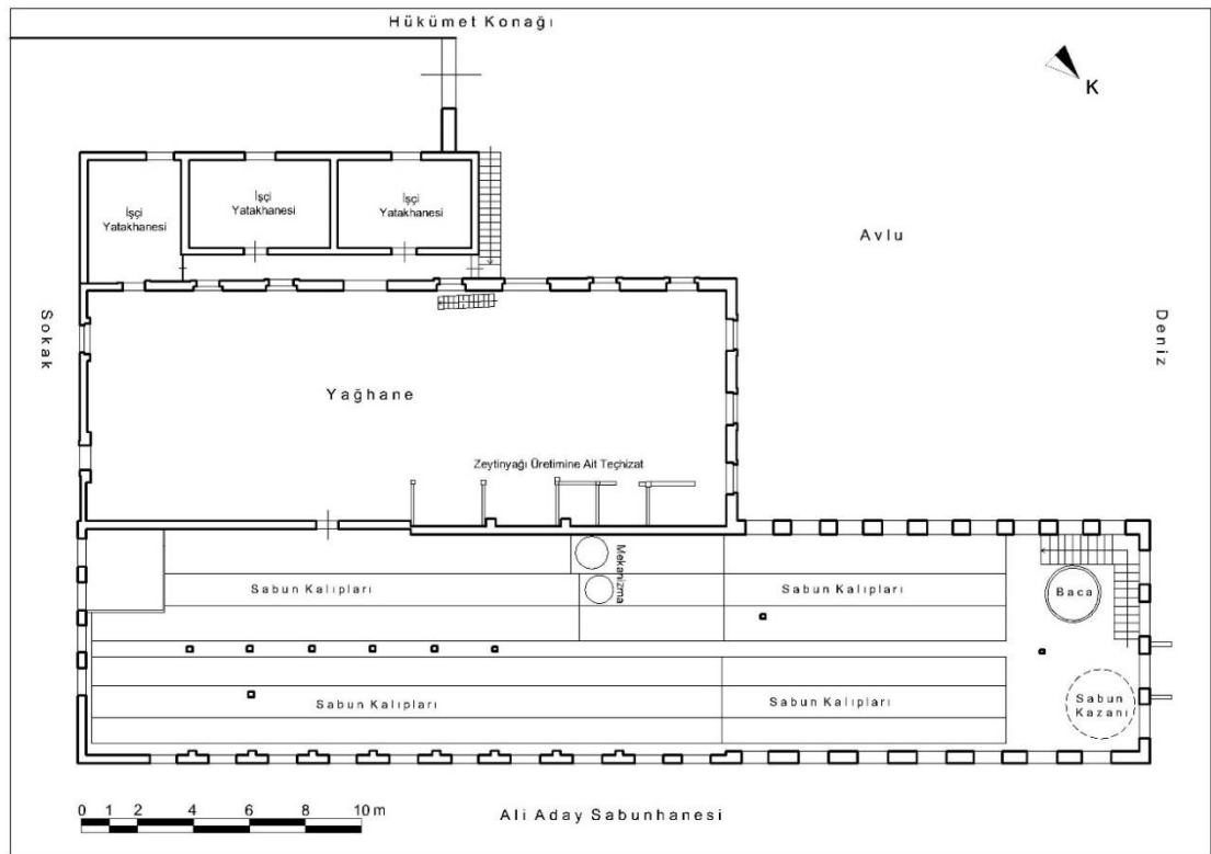
Çizim 44: Ayvalık Ertemler Sabunhanesi Birinci Kat Plânı (Ayvalık Belediyesi Arşivinden İşlenerek)
