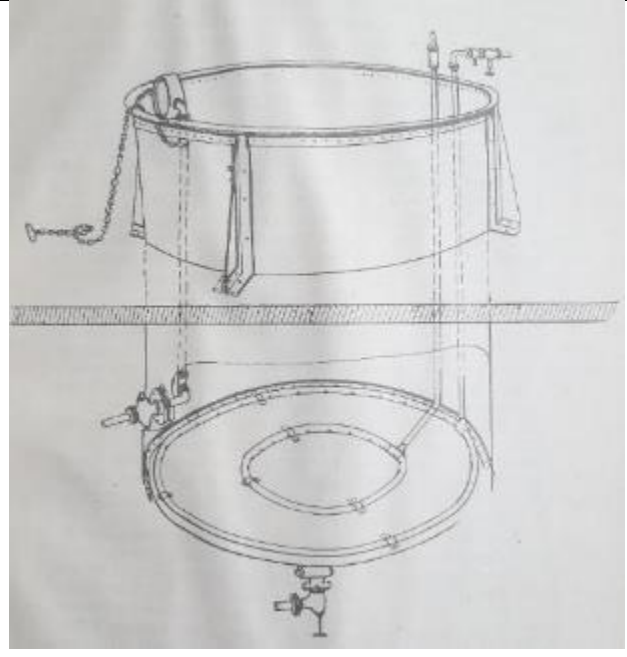
Fotoğraf 25: Buharlı Sabun Kazanı (TSOTBB, age, s. 47)
