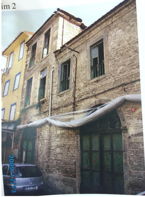
Fotoğraf 289: Konak Hamdi Dalan Sabunhanesi Kuzey Cephe, 2009 (Konak Belediyesi Arşivi)
