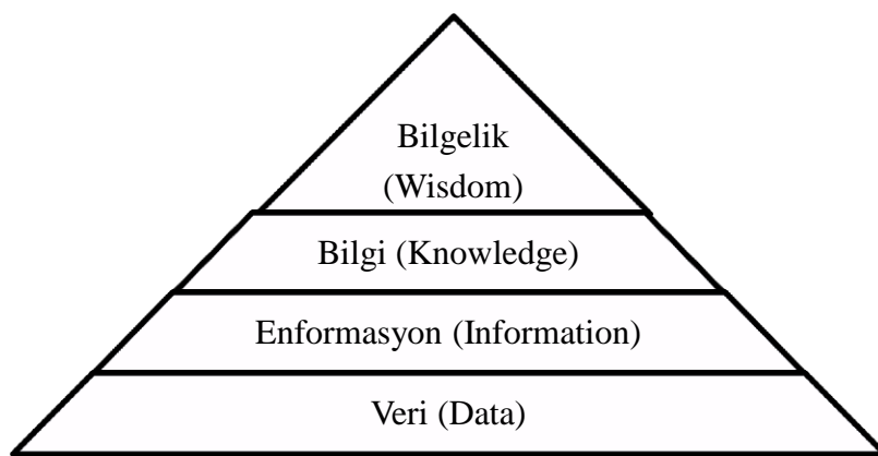
Şekil 2: DIKW Piramiti
