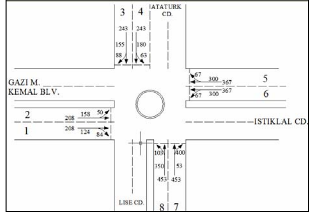
Şekil 2. Örnek kavşak link numaraları ve trafik yükleri
