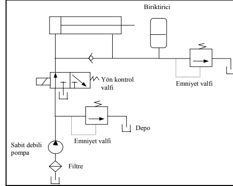
Şekil 8. Enerji güç kaynağı olarak biriktiricinin kullanılması (Esposito, 1997)
