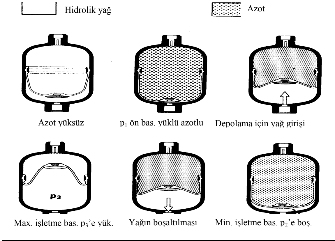
Şekil 4. Diyaframalı tip biriktiricinin çalışması
