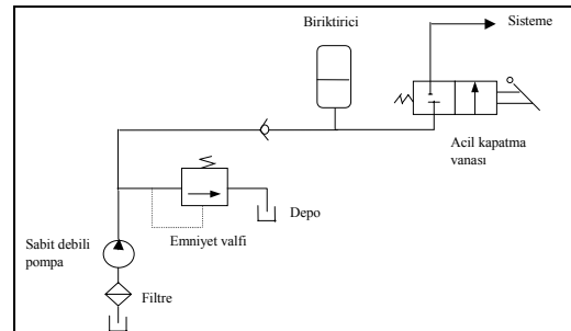
Şekil 9. Hidrolik şoku absorblayıcı olarak biriktiricinin kullanılması (Esposito, 1997)
