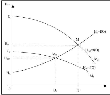
Şekil 7. Seri bağlı eş iki pompanın debi-yük karakteristikleri
