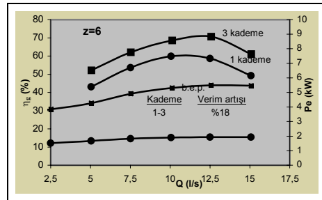
Şekil 11. Tek kademeli ve üç kademeli dalgıç pompaların performans karakteristiklerinin karşılaştırılması ( z = 6 )
