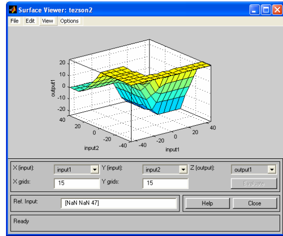
Şekil 9. Girişlerin ve çıkışın 3 boyutlu gösterimi
