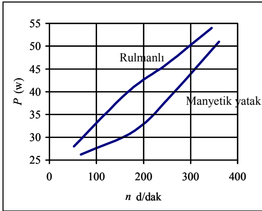
Şekil 13. Rulmanlı ve manyetik yatağa ait devir sayısı ve boşta çalışma gücü değişimi eğrileri
