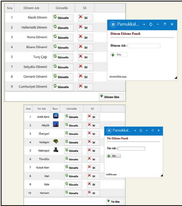
Şekil 7.Sistem ayarları
