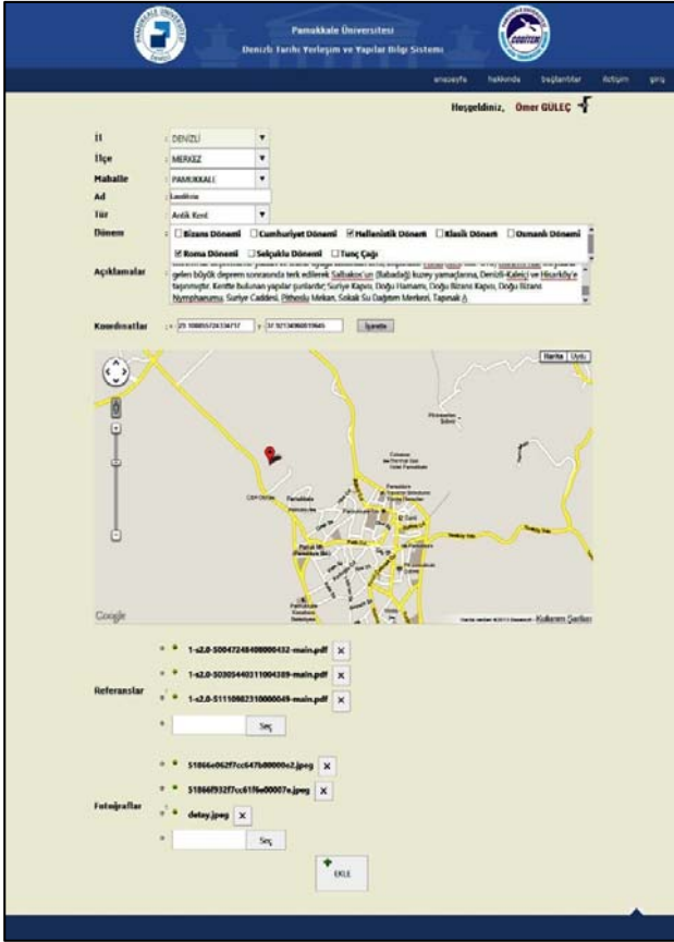
Şekil 6.Yapı ekleme sayfası
