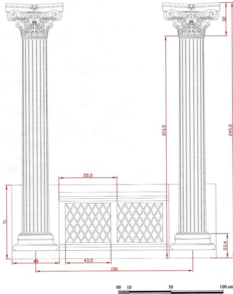
Çizim 1: Paye ve parapetlerin dıştan görünüşü ve ölçüleri
