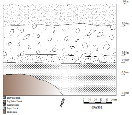
Çizim 3: Sondajın Kuzeybatı Kesiti
