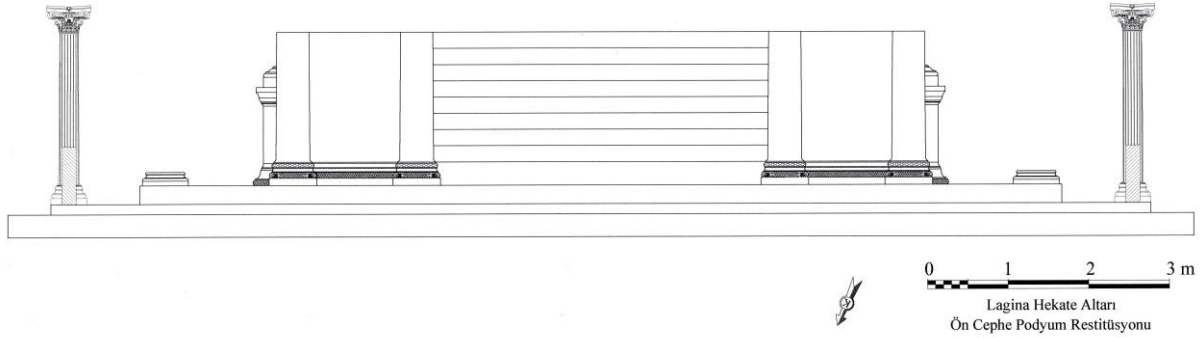
Çizim 8: Giriş Cephesinin Restitüsyonu
