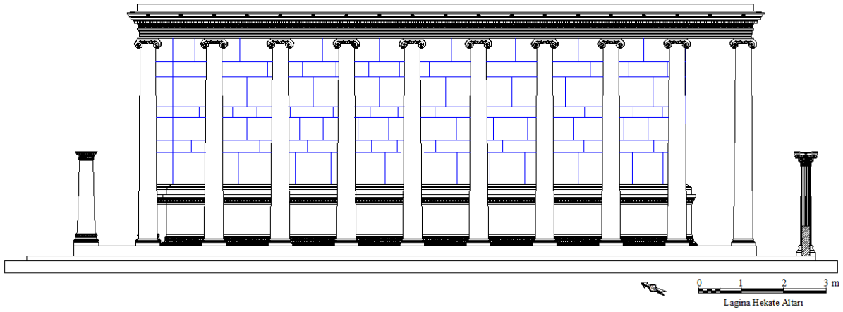
Çizim 14: Peristasisin Cephe Restitüsyonu
