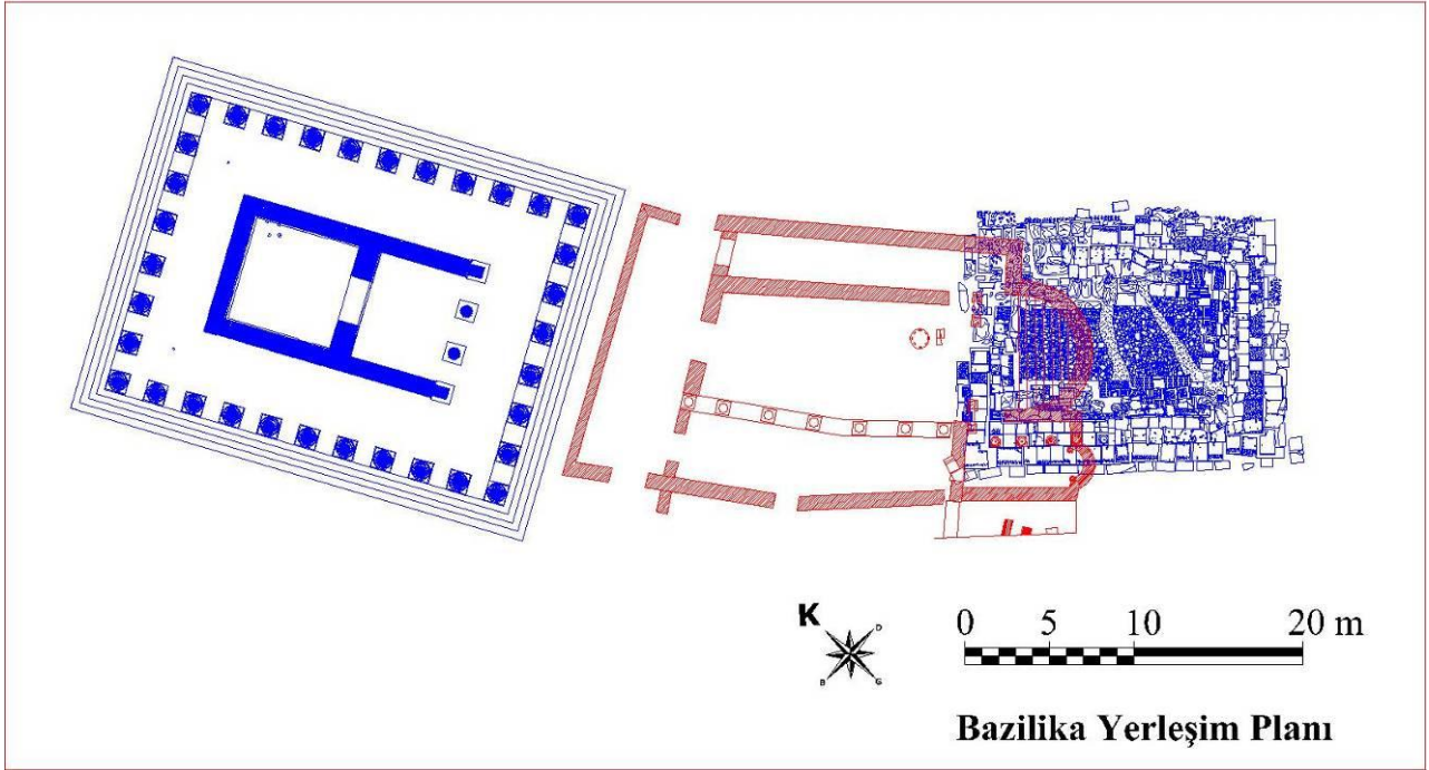
Çizim 1. Lagina Kutsal Alanı Kilisesi planı ve konumu
