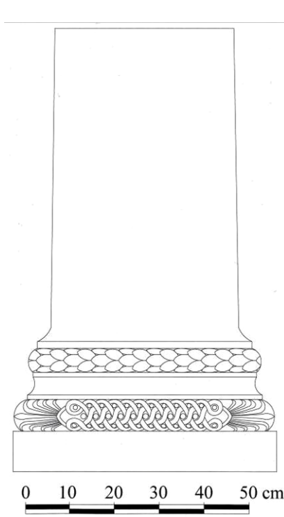
Çizim 5: Anta Kaidesi
