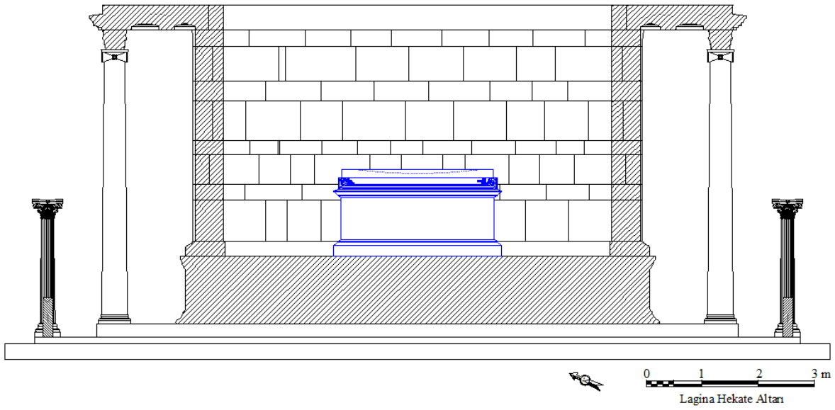
Çizim 16: Naos Duvarları ve Peristasis Sütunlarının Kesiti
