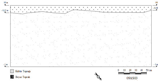
Çizim 5: Sondajın Batı Kesiti
