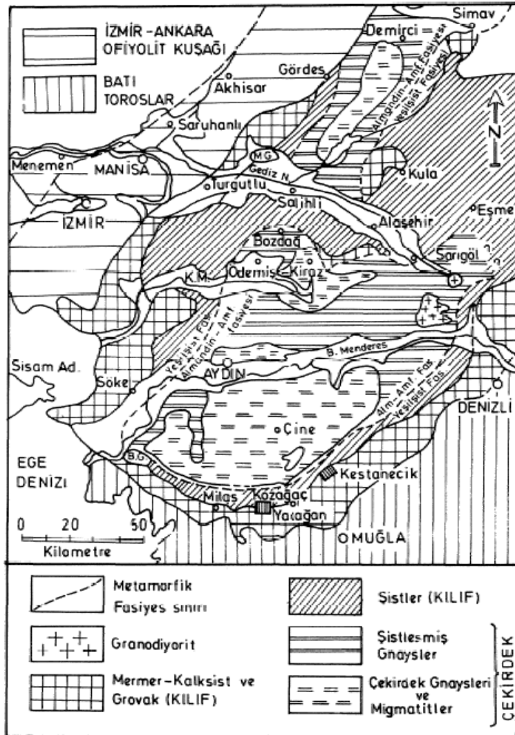
Şekil 1. Menderes Masifi'nin metamorfik birimleri (Dora, 1975).
