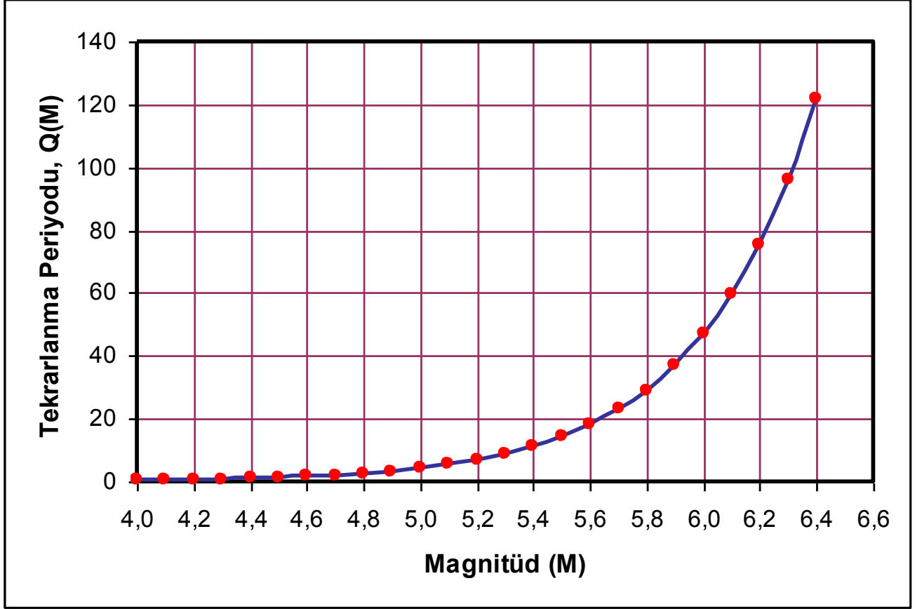
Şekil 6. Gumbel modeli kullanılarak belirlenmiş deprem tekrarlanma periyotları.
