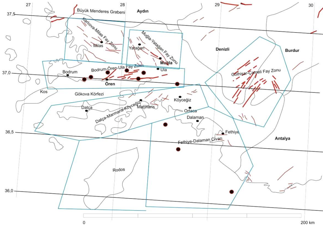
Şekil 4. İnceleme alanının da içinde bulunduğu bölgenin tektonik unsurları ve fay zonları.
