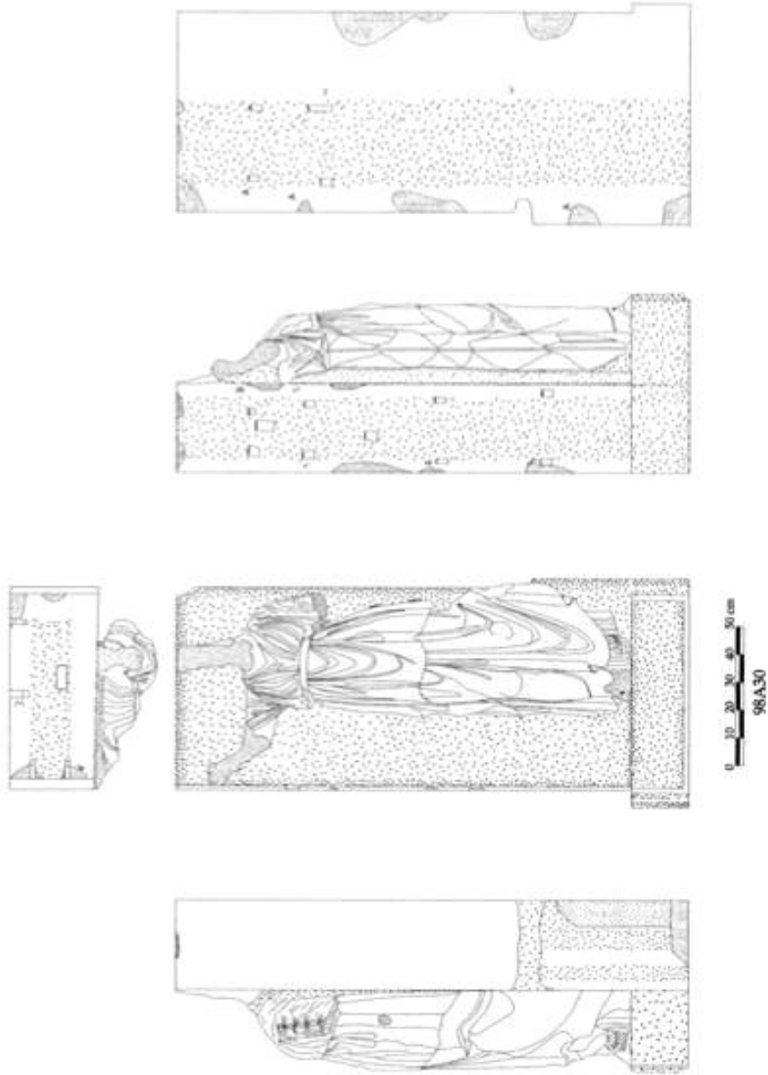
Çizim 1: Kabartmalı bloğun kesit ve görünüşleri
