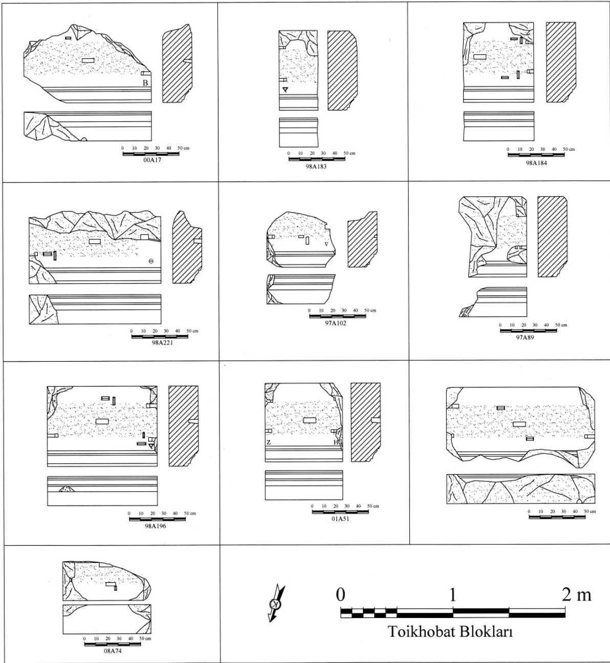
Çizim 7: Toikhobat Bloklarının Tasnif Alanındaki Mevcut Durumunu Gösteren Çizim
