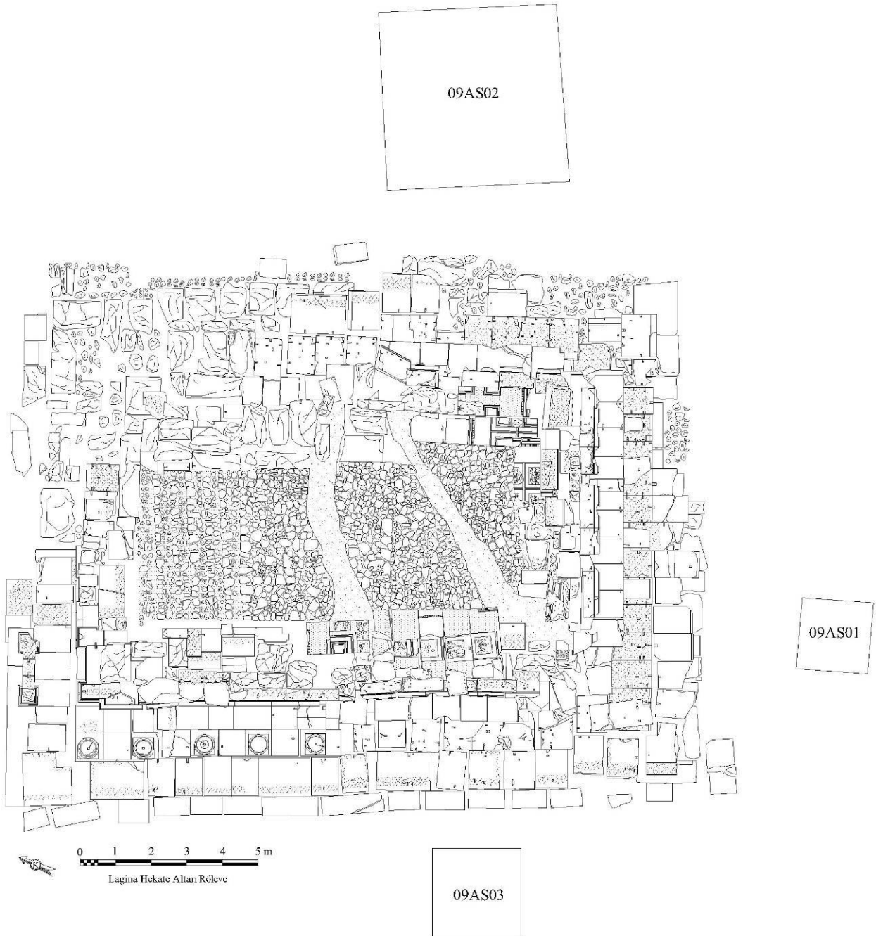
Çizim 1: Altar Çevresinde Açılan Sondajların Yeri ve Numaraları
