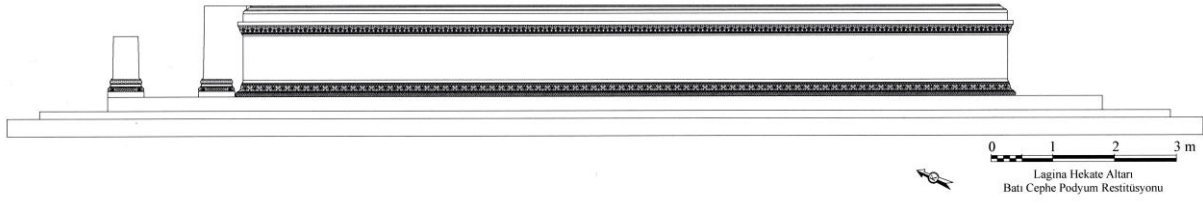
Çizim 9: Altarın Batı Cephesinin Restitüsyonu
