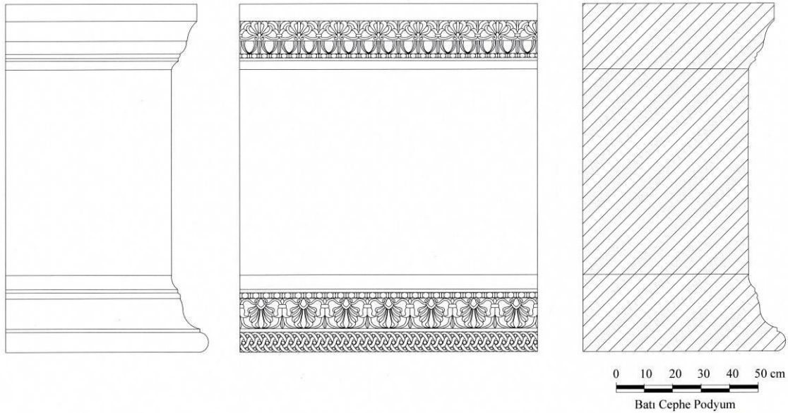
Çizim 4: Altarın Podyum Kısmı
