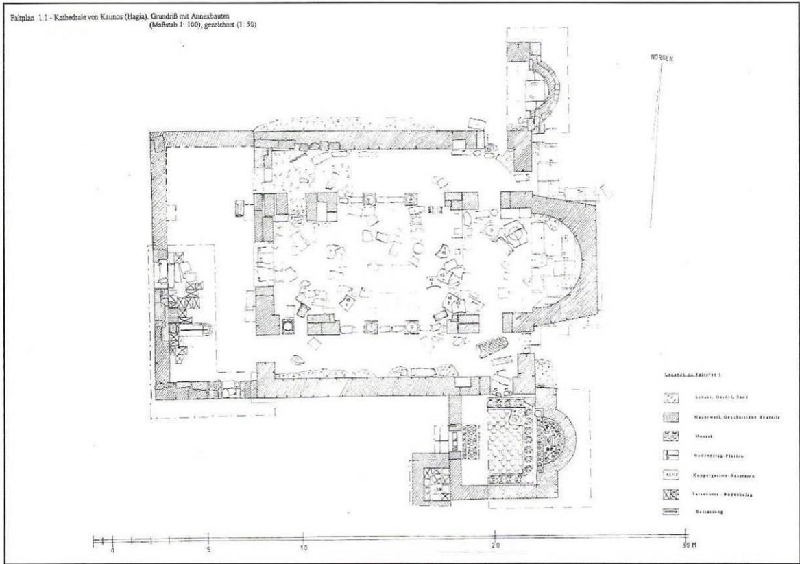
Çizim 4: Kaunos Bazilikası
