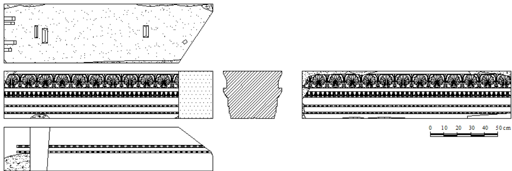
Çizim 15: Peristasis'e Ait Arşitrav-Friz Bloğu
