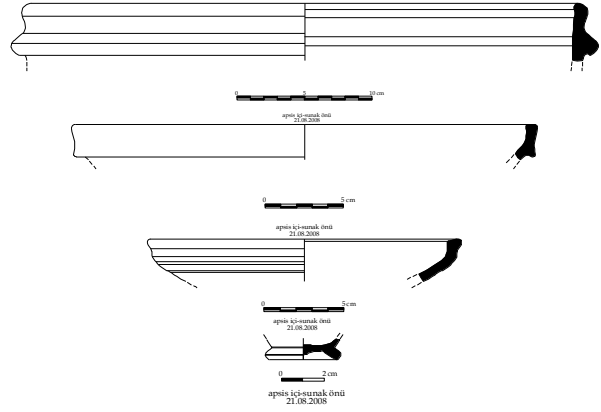
Çizim 5: Apsis içi-sunak önü buluntuları
