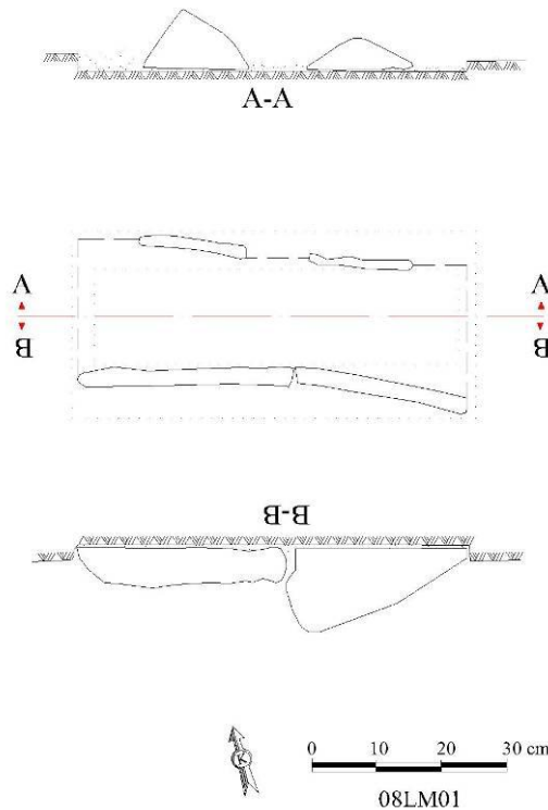
Çizim 8: 08LM01 Numaralı Mezarın Plan ve Görünüş Çizimleri
