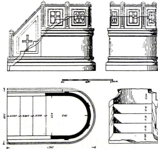
Çizim 7: Ambon Düzenlemesi
