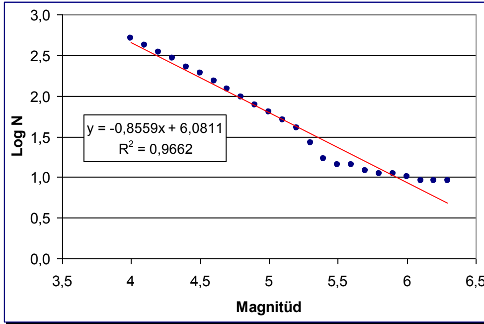
Şekil 5. İncelenen veriler için ortaya konulan magnitüd – frekans ilişkisi
