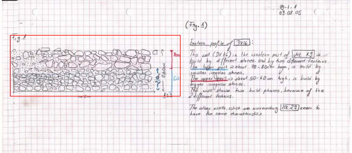
Fig. 41: Dv. 16'nın Kesit Çizimi
