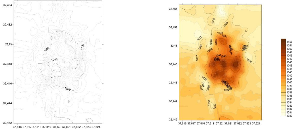
Figür 3: Surfer 13 ile Oluşturulmuş Topoğrafik Planlar.
