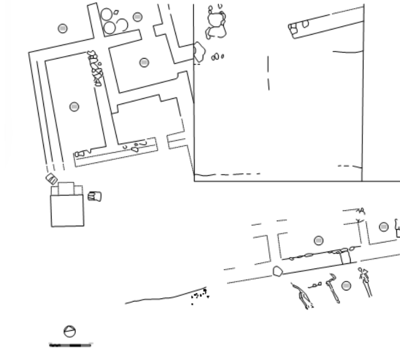
Figür 7: T Açması Planı (Alp 1980a, Lev. XXXIV).
