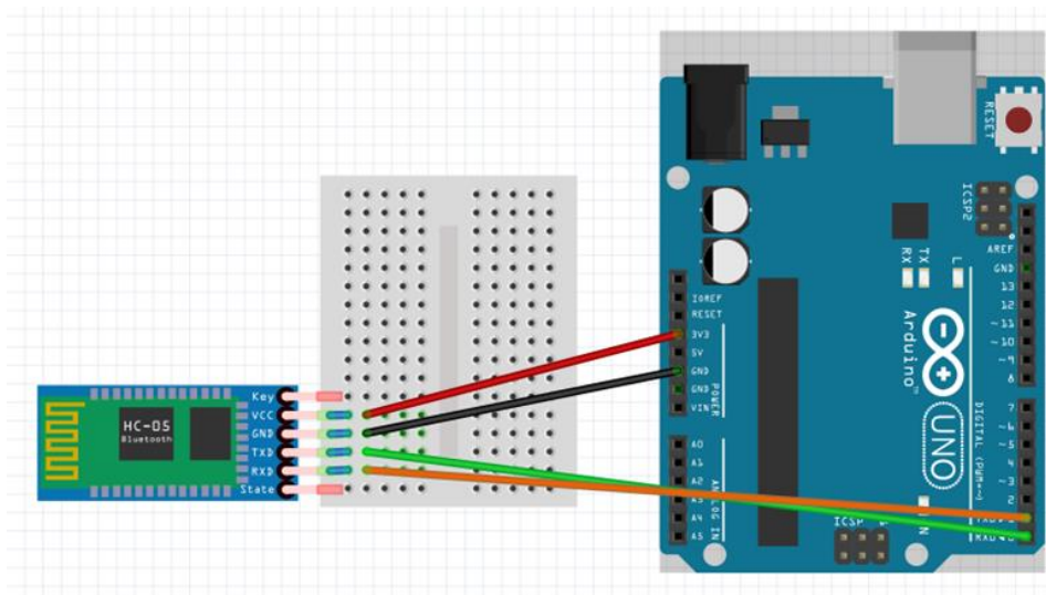
Şekil 1. Bluetooth Modülünün Arduino ile Bağlantısı
