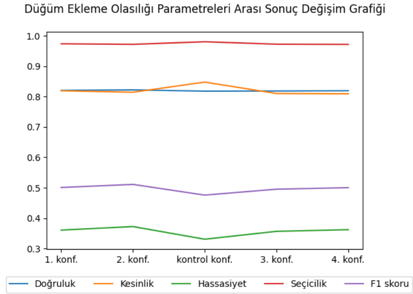
Şekil 5.3: Düğüm ekleme olasılığına göre performans değişim grafiği
