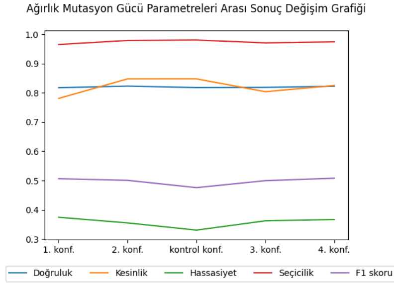
Şekil 5.5: Ağırlık mutasyon gücüne göre performans değişim grafiği
